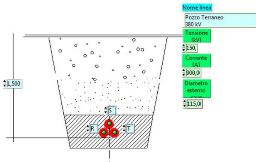
Figura 5 - Sezione tipo
