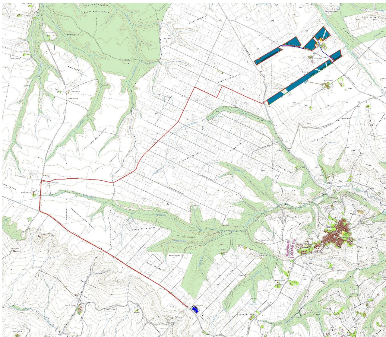
Figura 1 — Inquadramento della centrale fotovoltaica su CTR
