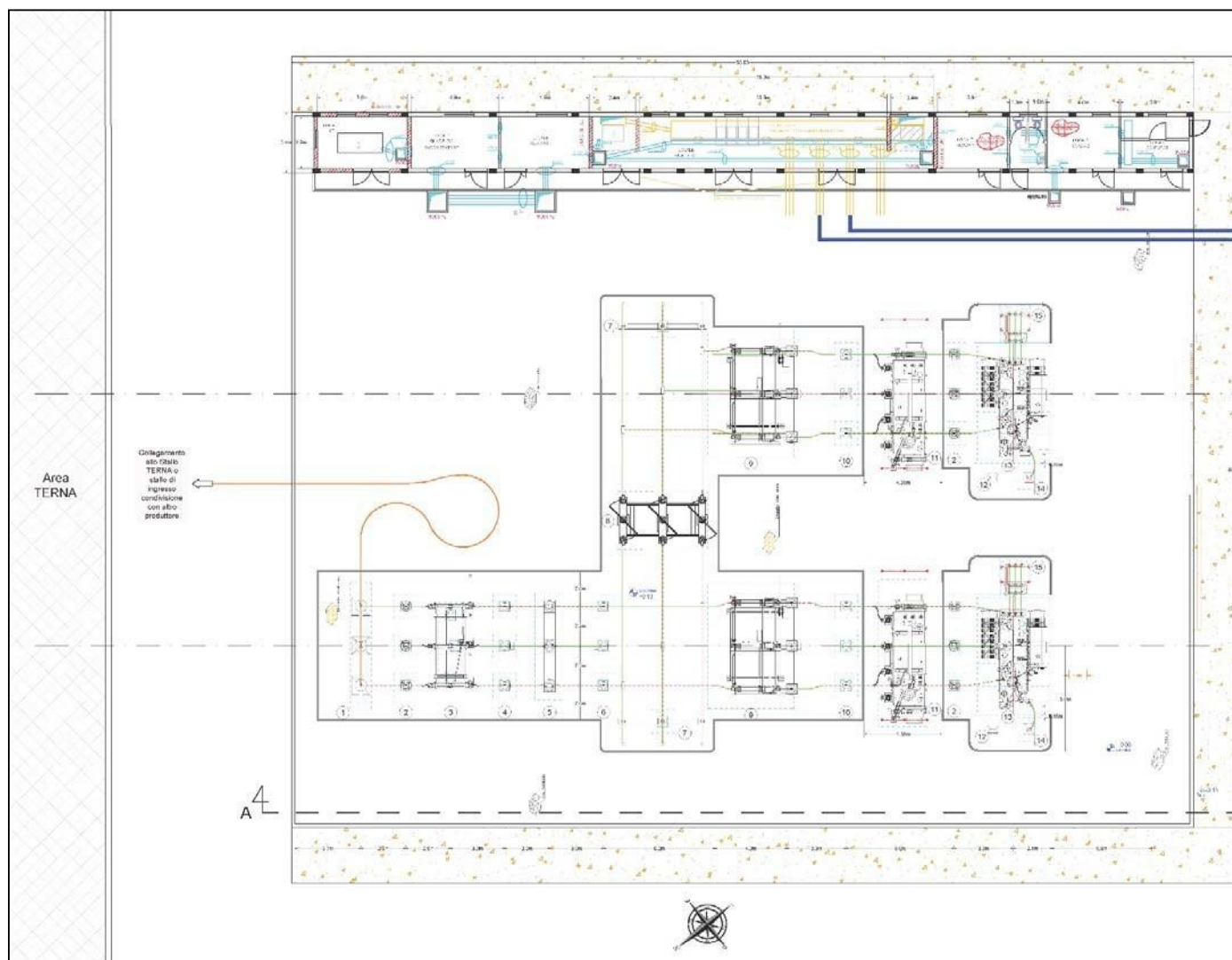
FIGURA 2: Planimetria elettromeccanica SottoStazione Produttore
