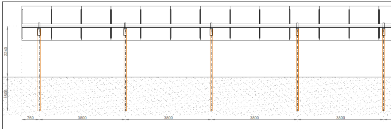
Figure 3: stralcio prospetto struttura di supporto 1x30P-30
