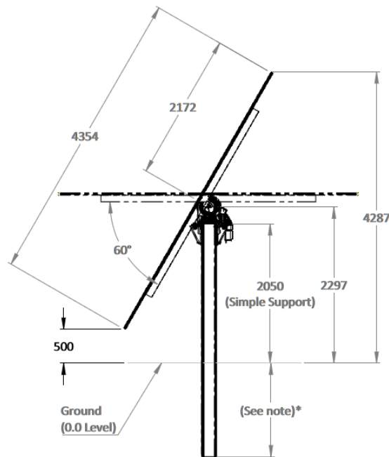
Figura 5-3: Sezione tipo struttura porta pannelli
