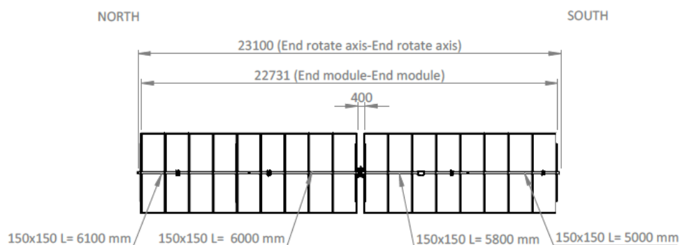
Figura 5-1: Struttura porta pannelli tipo Soltec 2x17
