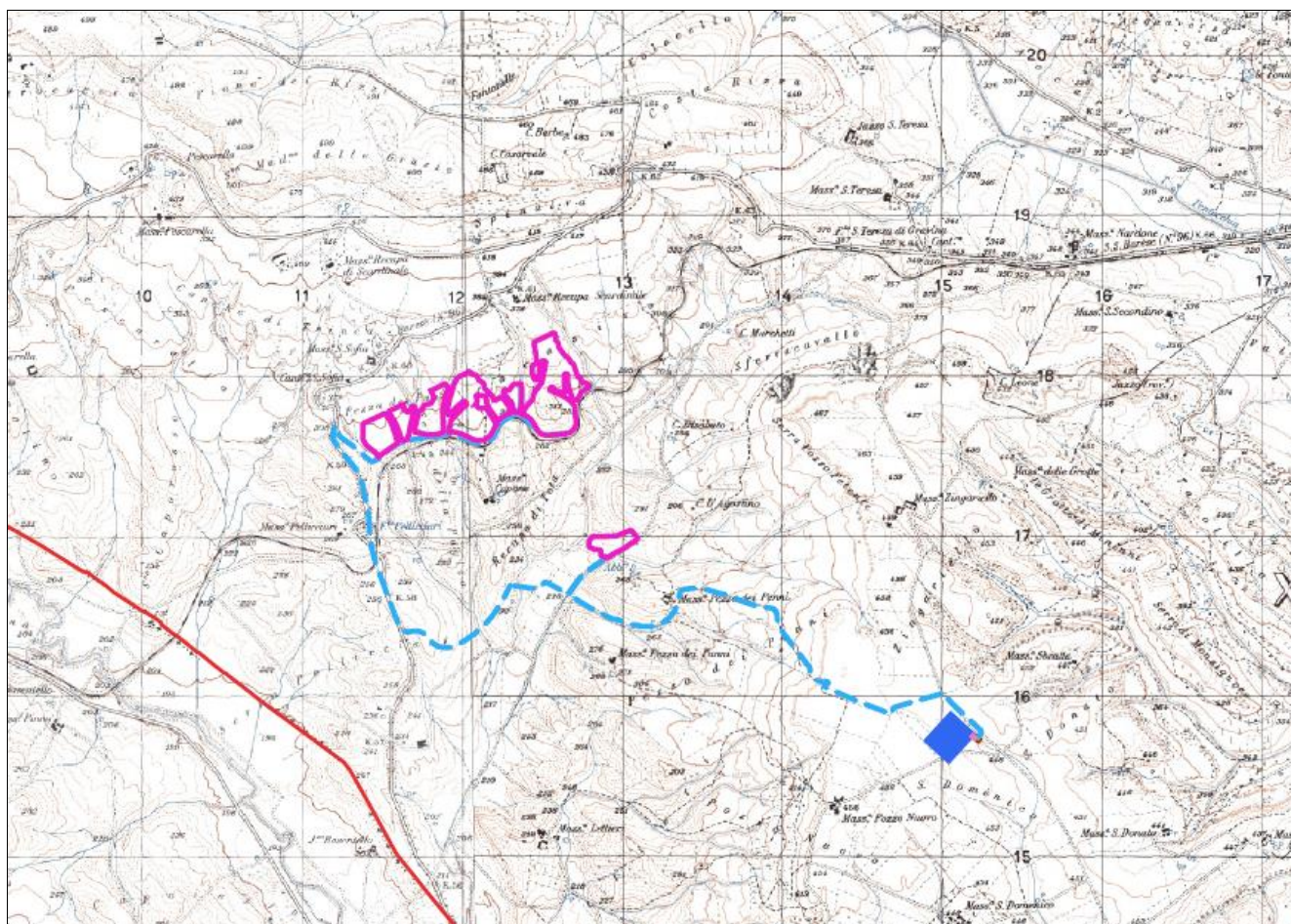
Figura 3-1: Inquadramento layout di impianto su base IGM
