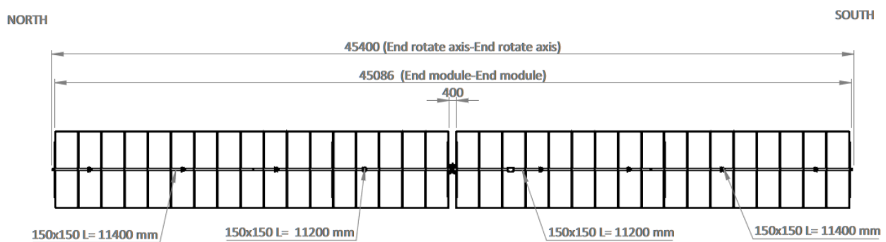
Figura 1-3: Struttura porta pannelli tipo Soltec 2x34
