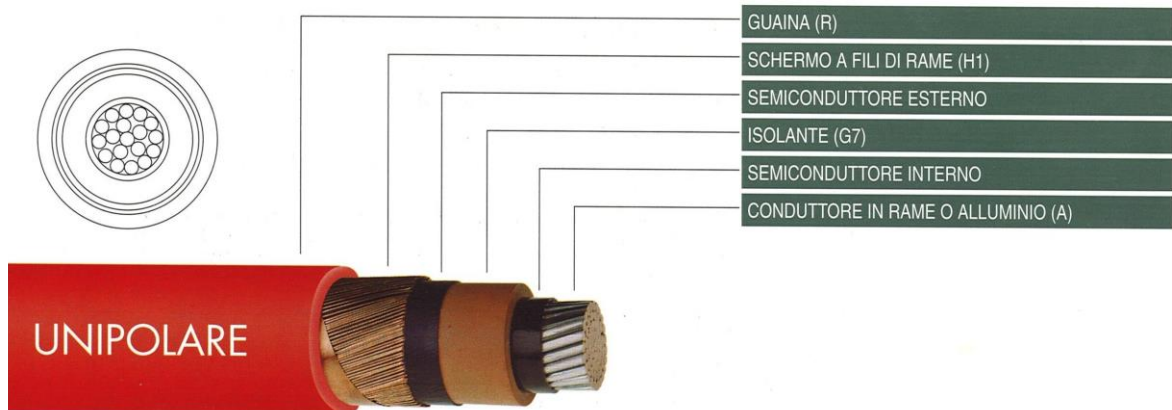
Fig. 1: caratteristiche cavi unipolari
