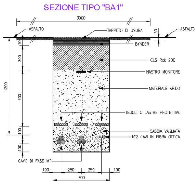
Figura 2: Sezione tipica di posa della linea in cavo su strade sterrate
