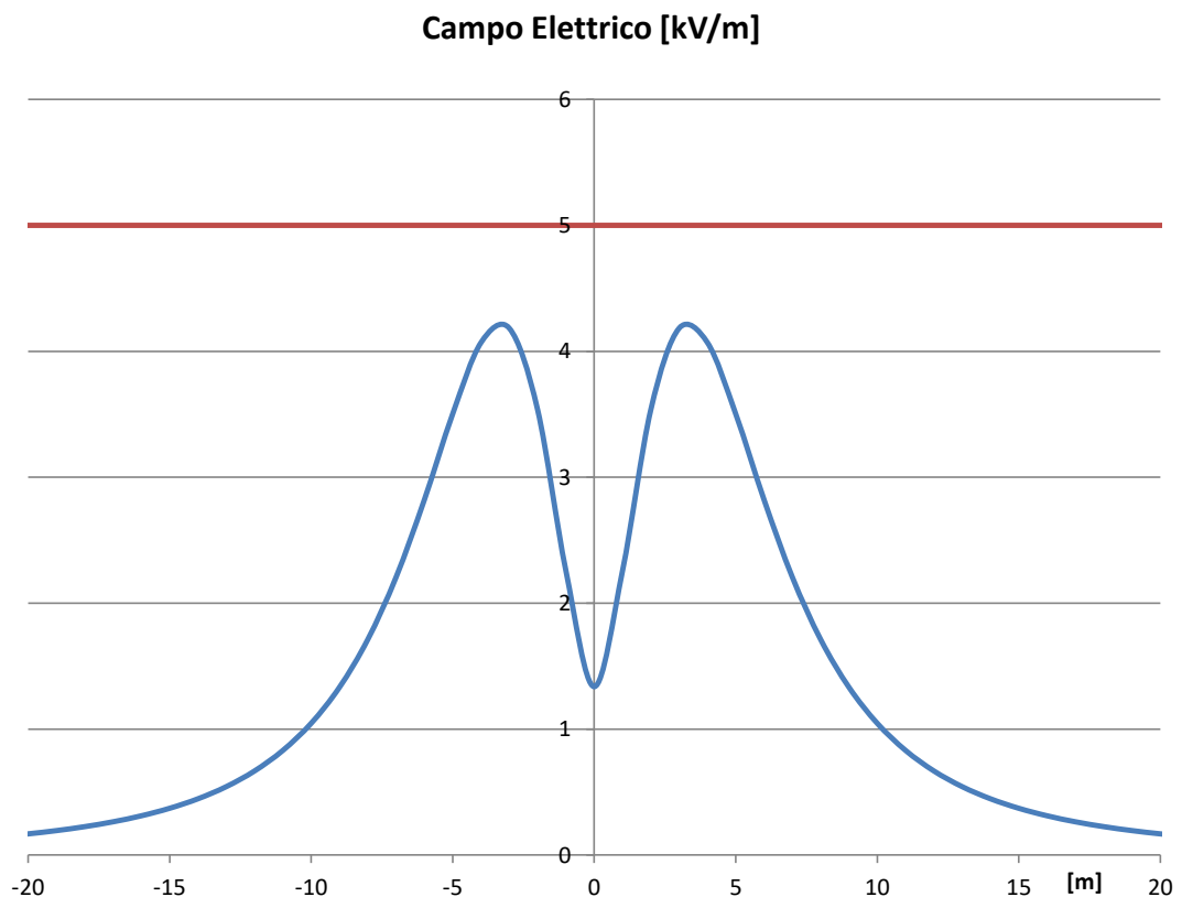
Figura 5: Campo elettrico al suolo generato dal sistema di sbarre a 150 kV
