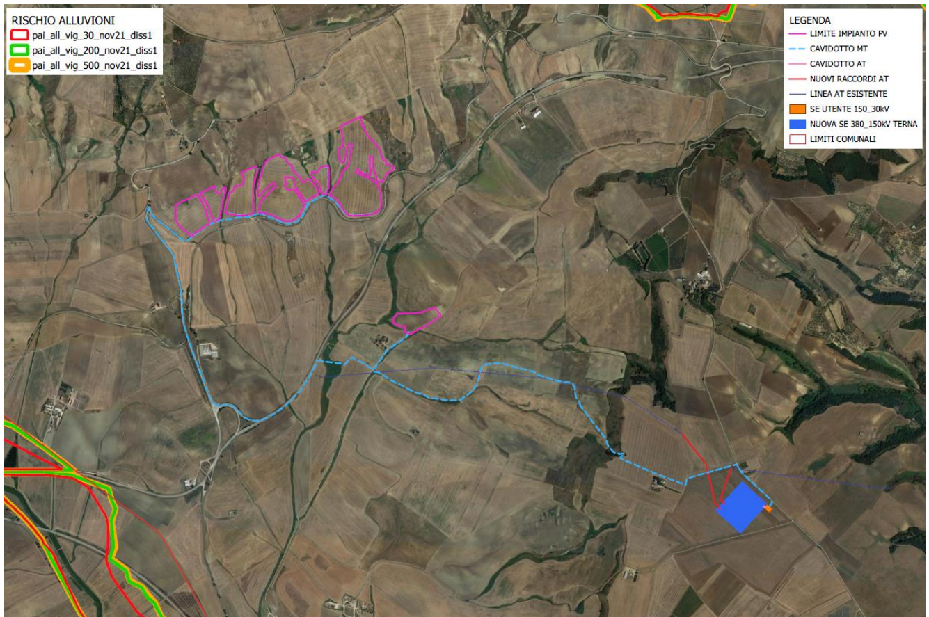
Figura 3-16: Estratto del Piano stralcio per la difesa dal rischio idrogeologico-Rischio alluvioni nell'area di intervento e layout di progetto
