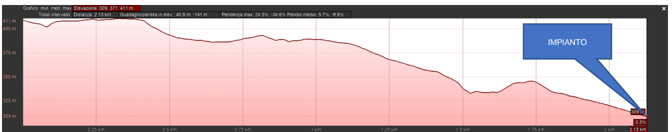
Figura 3-41: Profilo altimetrico dal punto di vista 05 verso l'impianto
