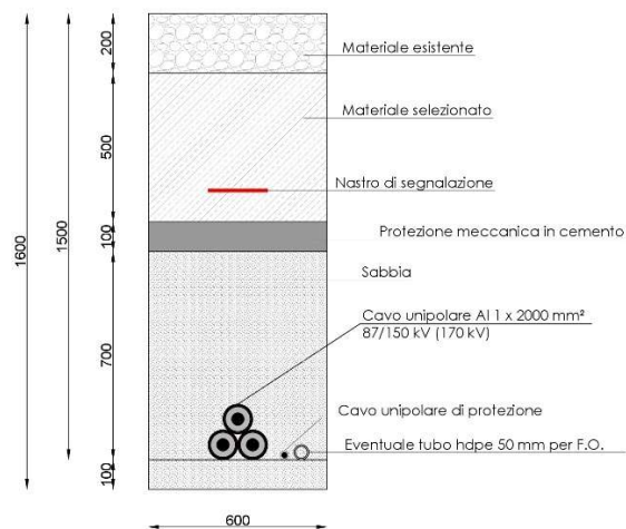
Figura 1 - Tipologico scavo per cavo AT
