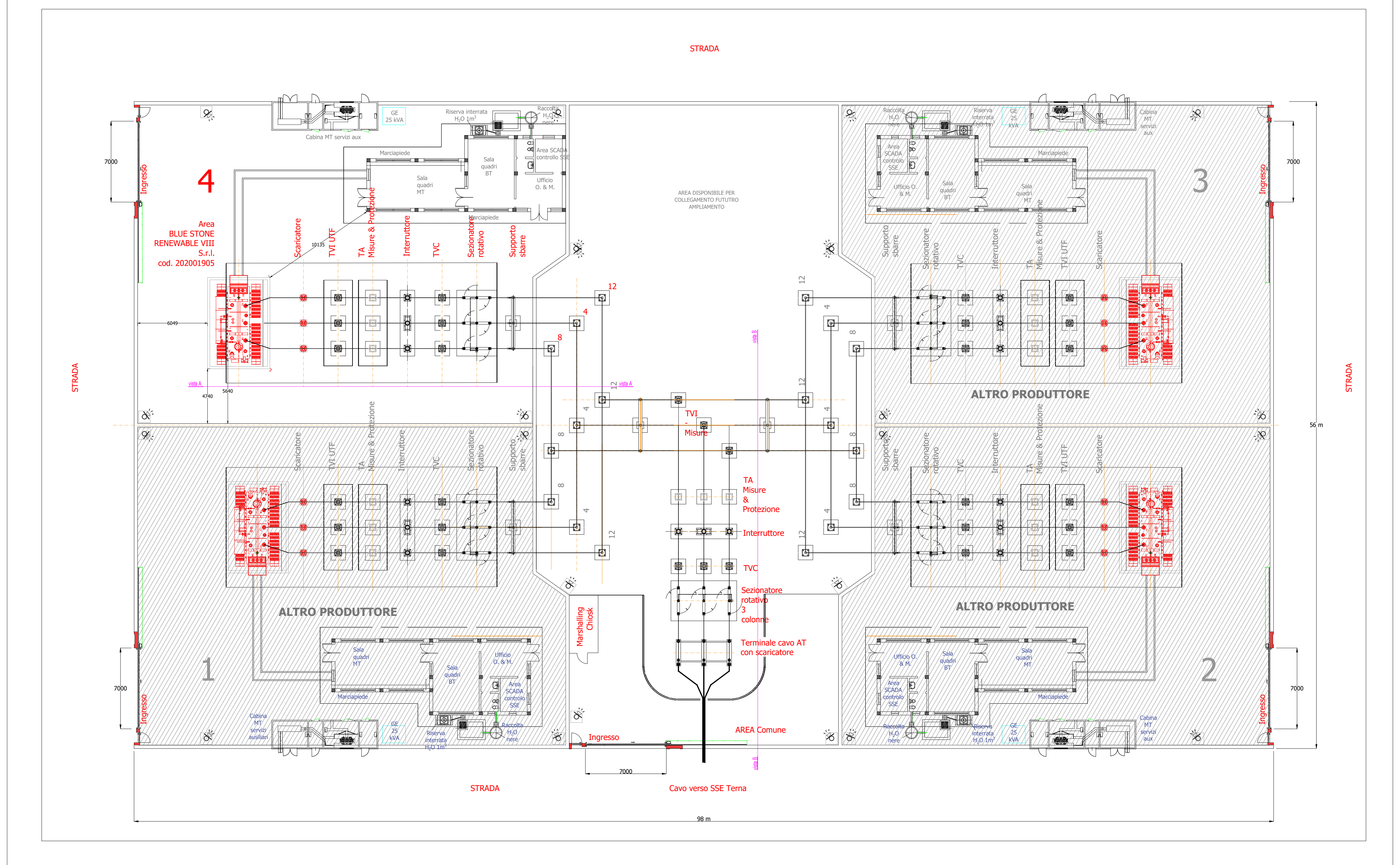
PLANIMETRIA SOTTOSTAZIONE
