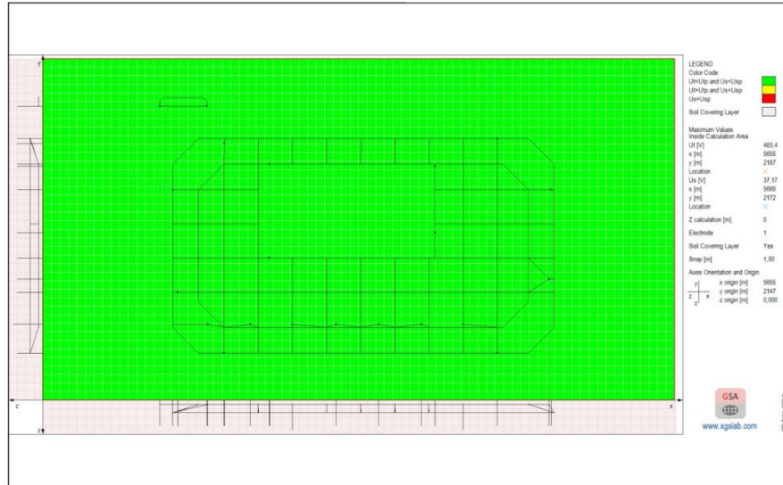
Figura 5 – Zona sicura (dove U_t < U_{tp} ed U_s < U_{sp} ) interna al piazzale, calcolata considerando lo strato superficiale di asfalto (SCL)
