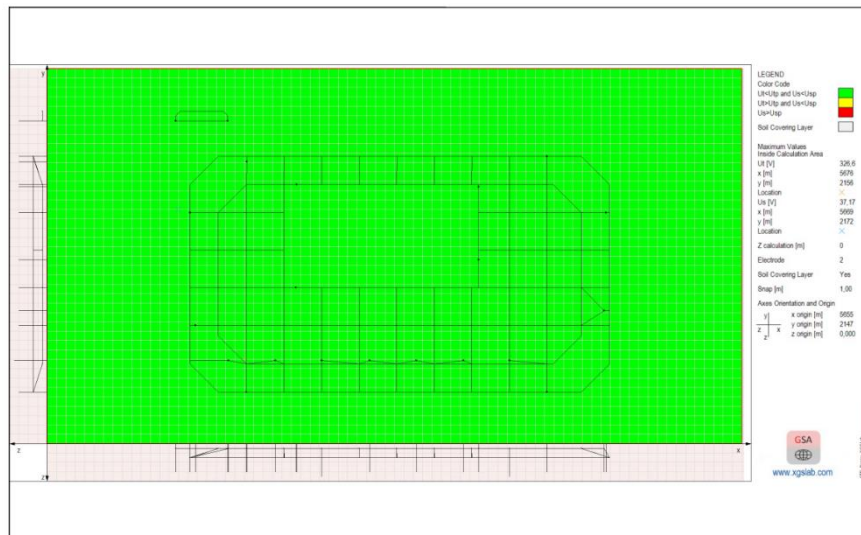
Figura 6 – Zona sicura (dove U_t < U_{tp} ed U_s < U_{sp} ), esterna al piazzale, calcolata considerando lo strato superficiale di asfalto (SCL)
