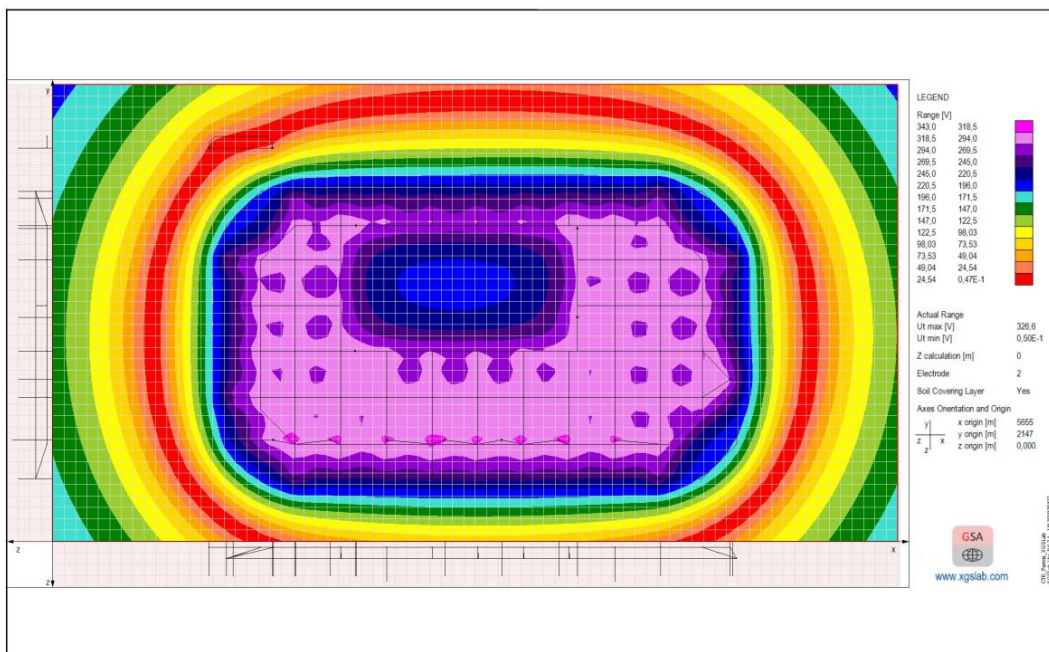
Figura 4 – Tensione di Contatto U_t calcolata considerando lo strato superficiale di asfalto (SCL)
