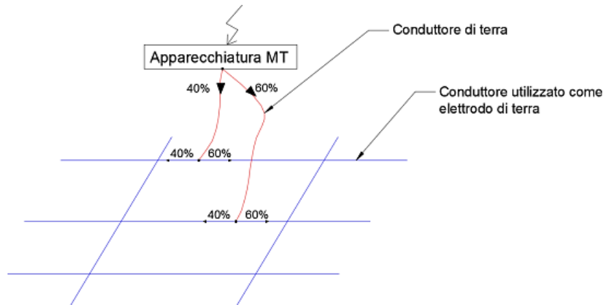
Figura 7 – Fattore di divisione k_M
