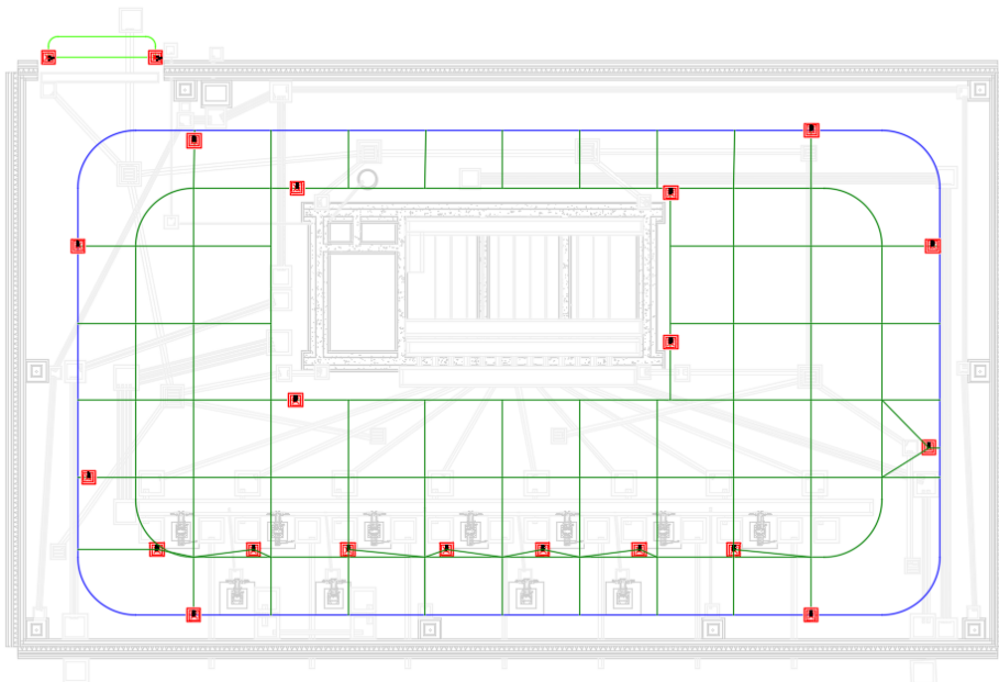
Figura 1– Impianto di terra di Piazzale
