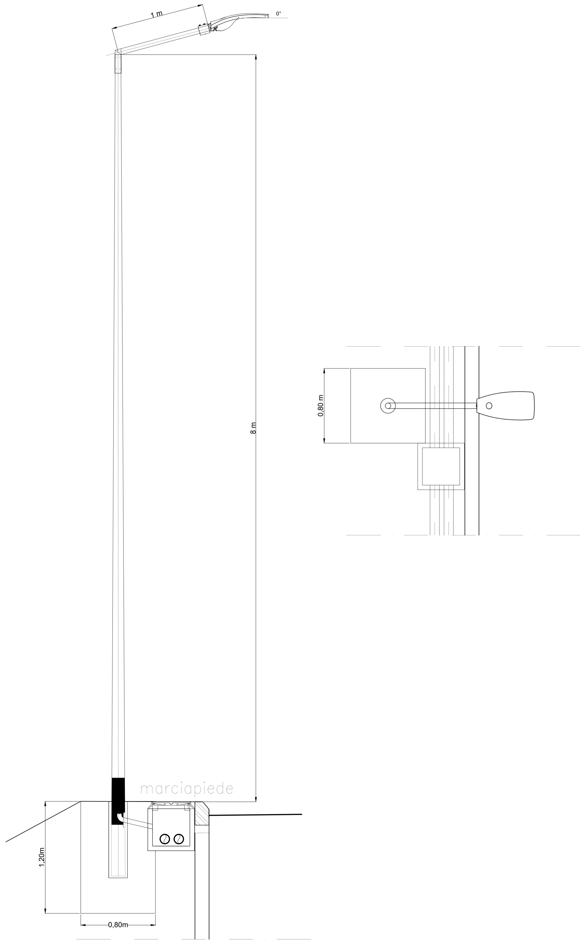
Sezione e pianta PALINA Scala 1:20
