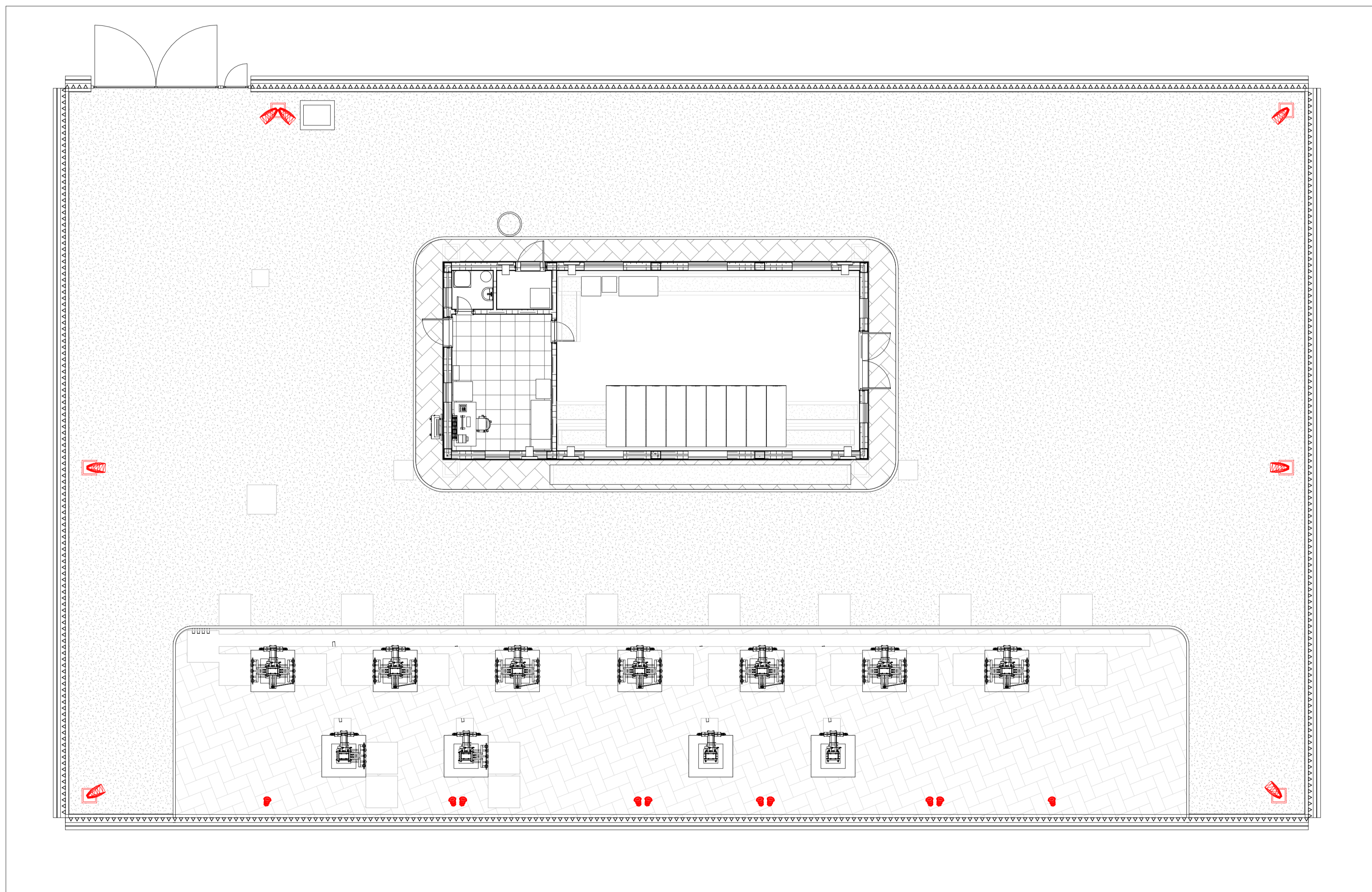
1 Layout LFM 1 : 100
