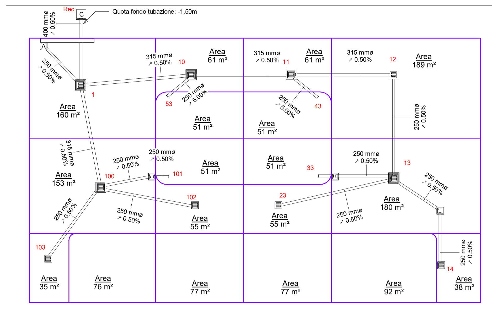
2 Rete Idrica 1 : 200
