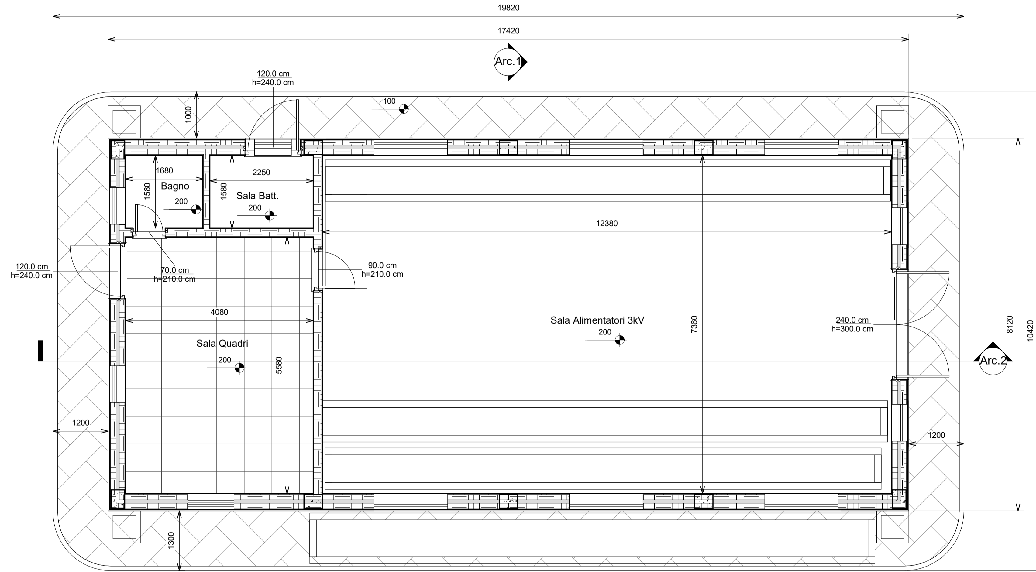
1 Pianta piano Terra 1 : 50
