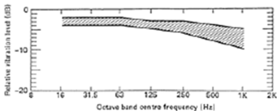
Figura 5-8 Attenuazione delle vibrazioni nel passaggio da un piano al successivo
