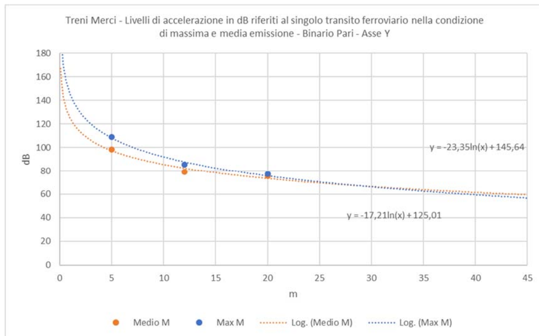
Figura 5-2 Individuazione della legge di propagazione delle vibrazioni nel terreno sulla base dei dati sperimentali lungo l'asse Y per la tipologia di treno merci nella condizione di massima e media emissione.
