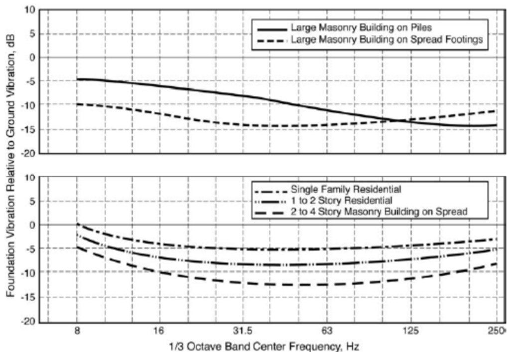
Figura 5-7 Risposta delle fondazioni per diverse tipologie di edifici (Fonte: FTA, USA)
