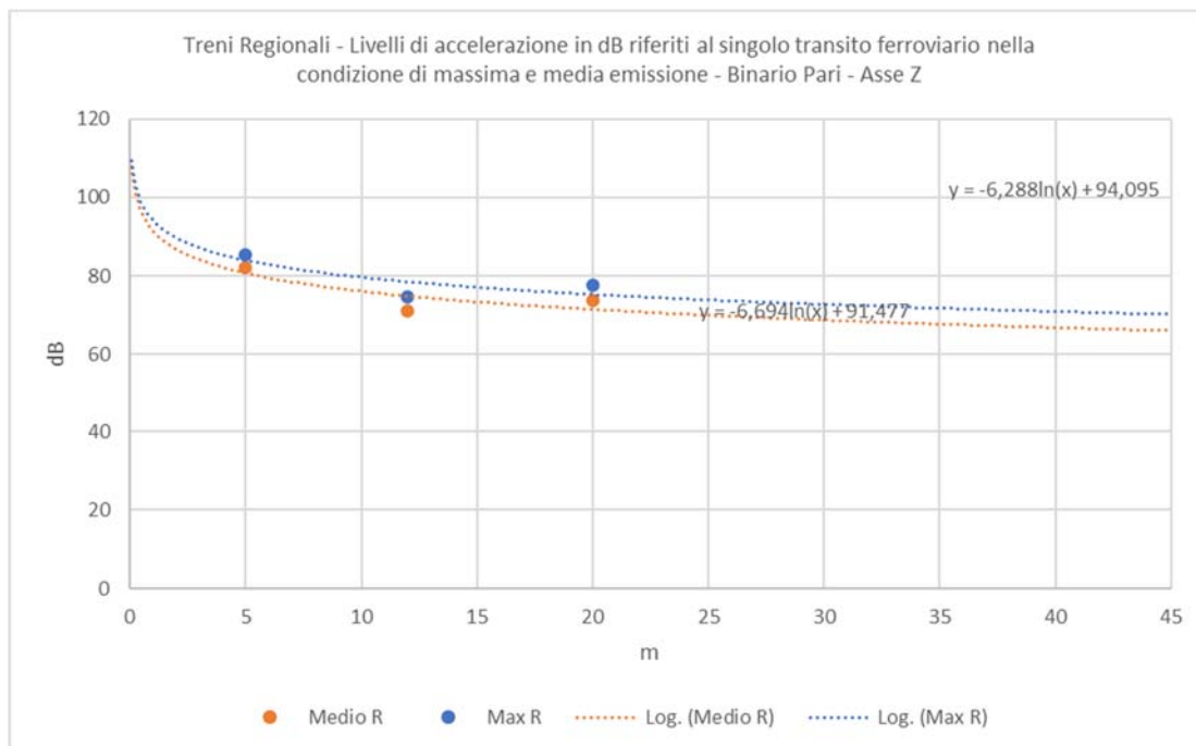
Figura 5-6 Individuazione della legge di propagazione delle vibrazioni nel terreno sulla base dei dati sperimentali lungo l'asse Z per la tipologia di treno regionale nella condizione di massima e media emissione.
