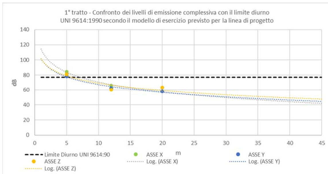
Figura 6-1 1° tratto - Confronto dei livelli di emissione complessiva all'interno degli edifici con i limiti UNI 9614:1990 in funzione della distanza dal binario secondo il modello di esercizio previsto – Periodo diurno.
