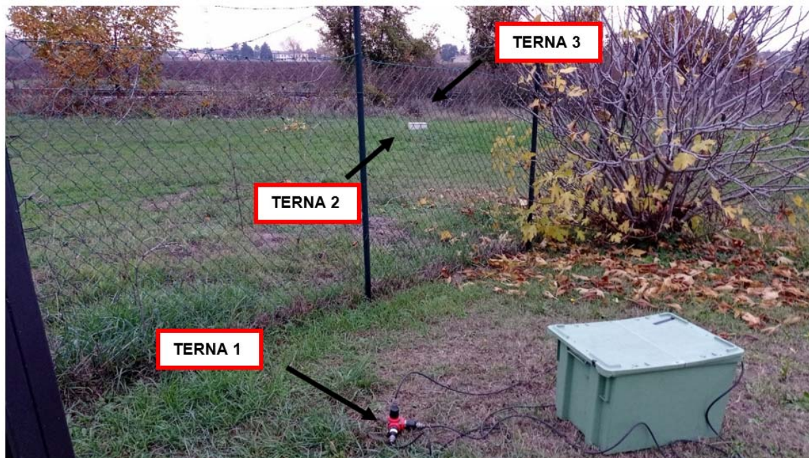
Figura 4-3 Foto di installazione
