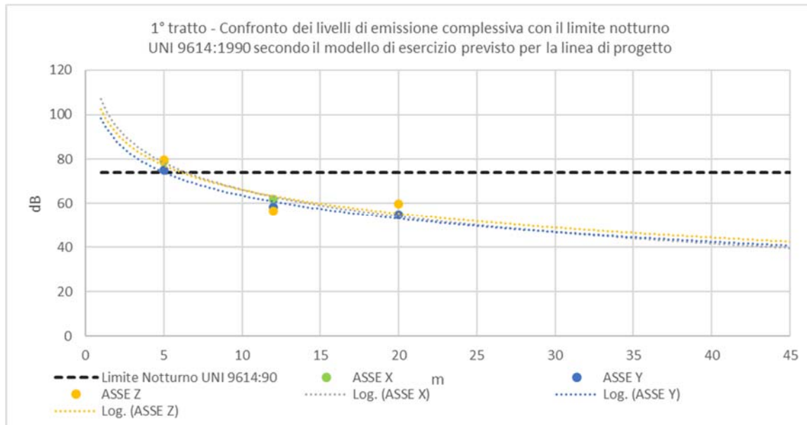
Figura 6-2 – 1° tratto. Confronto dei livelli di emissione complessiva all'interno degli edifici con i limiti UNI 9614:1990 in funzione della distanza dal binario secondo il modello di esercizio previsto – Periodo notturno.
