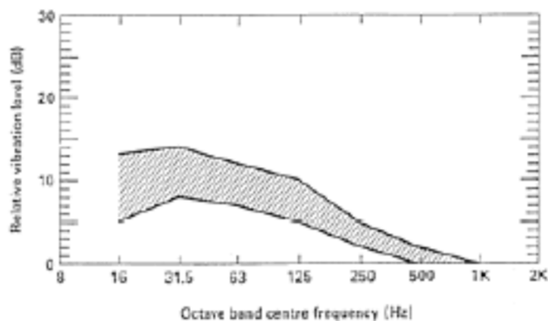
Figura 5-9 Amplificazione prodotta dai solai
