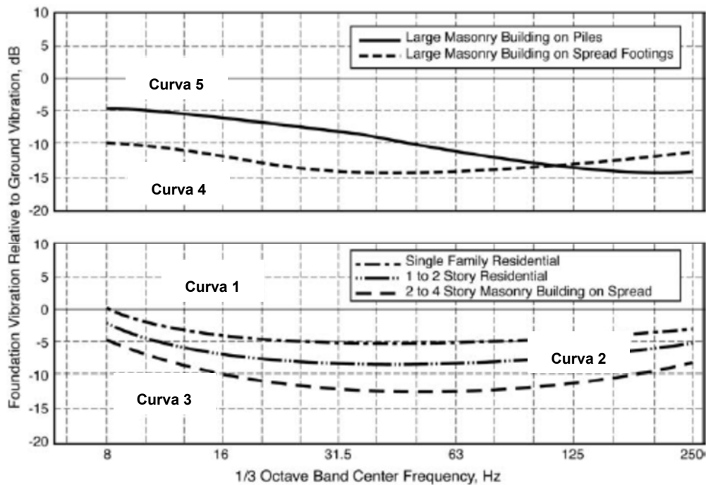
Figura 5-10 Fattori correttivi dovuti alla tipologia di fondazione
