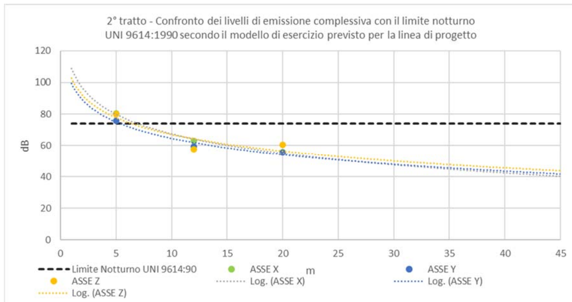
Figura 6-4 – 2° tratto. Confronto dei livelli di emissione complessiva all'interno degli edifici con i limiti UNI 9614:1990 in funzione della distanza dal binario secondo il modello di esercizio previsto – Periodo notturno.
