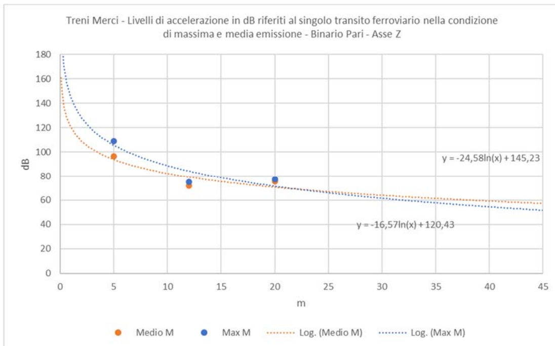
Figura 5-3 Individuazione della legge di propagazione delle vibrazioni nel terreno sulla base dei dati sperimentali lungo l'asse Z per la tipologia di treno merci nella condizione di massima e media emissione.
