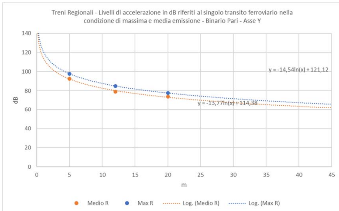
Figura 5-5 Individuazione della legge di propagazione delle vibrazioni nel terreno sulla base dei dati sperimentali lungo l'asse Y per la tipologia di treno regionale nella condizione di massima e media emissione.
