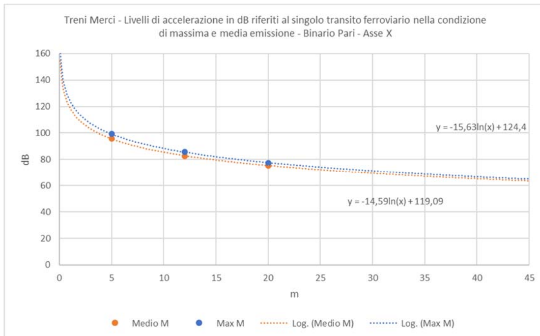
Figura 5-1 Individuazione della legge di propagazione delle vibrazioni nel terreno sulla base dei dati sperimentali lungo l'asse X per la tipologia di treno merci nella condizione di massima e media emissione.
