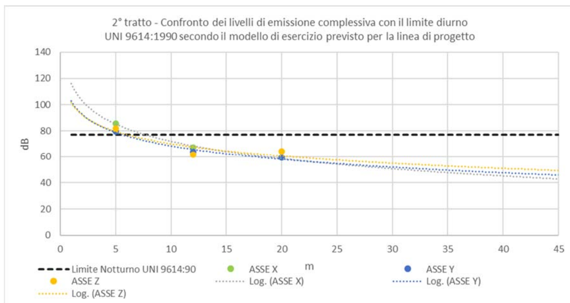
Figura 6-3 2° tratto - Confronto dei livelli di emissione complessiva all'interno degli edifici con i limiti UNI 9614:1990 in funzione della distanza dal binario secondo il modello di esercizio previsto – Periodo diurno.
