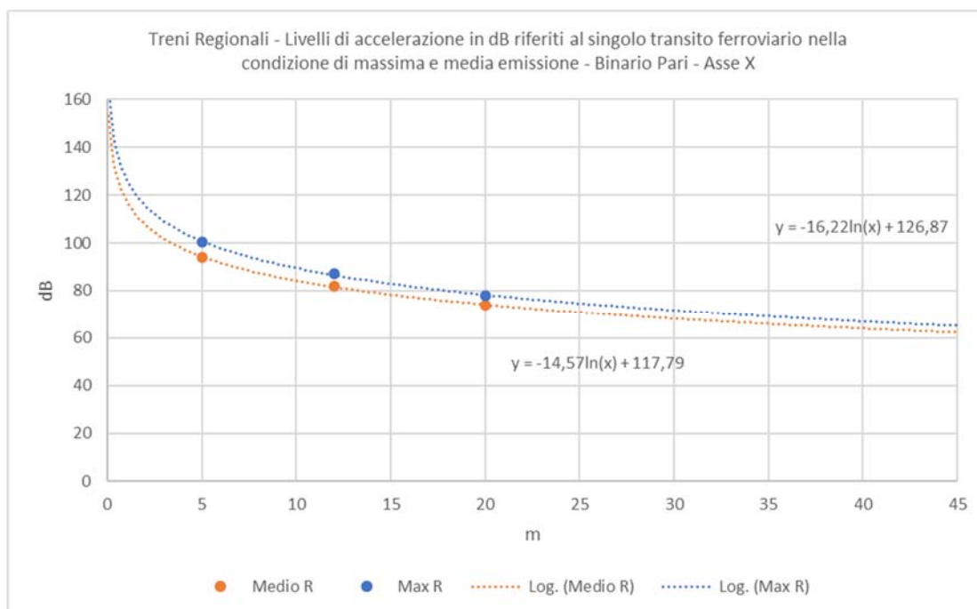
Figura 5-4 Individuazione della legge di propagazione delle vibrazioni nel terreno sulla base dei dati sperimentali lungo l'asse X per la tipologia di treno regionale nella condizione di massima e media emissione.
