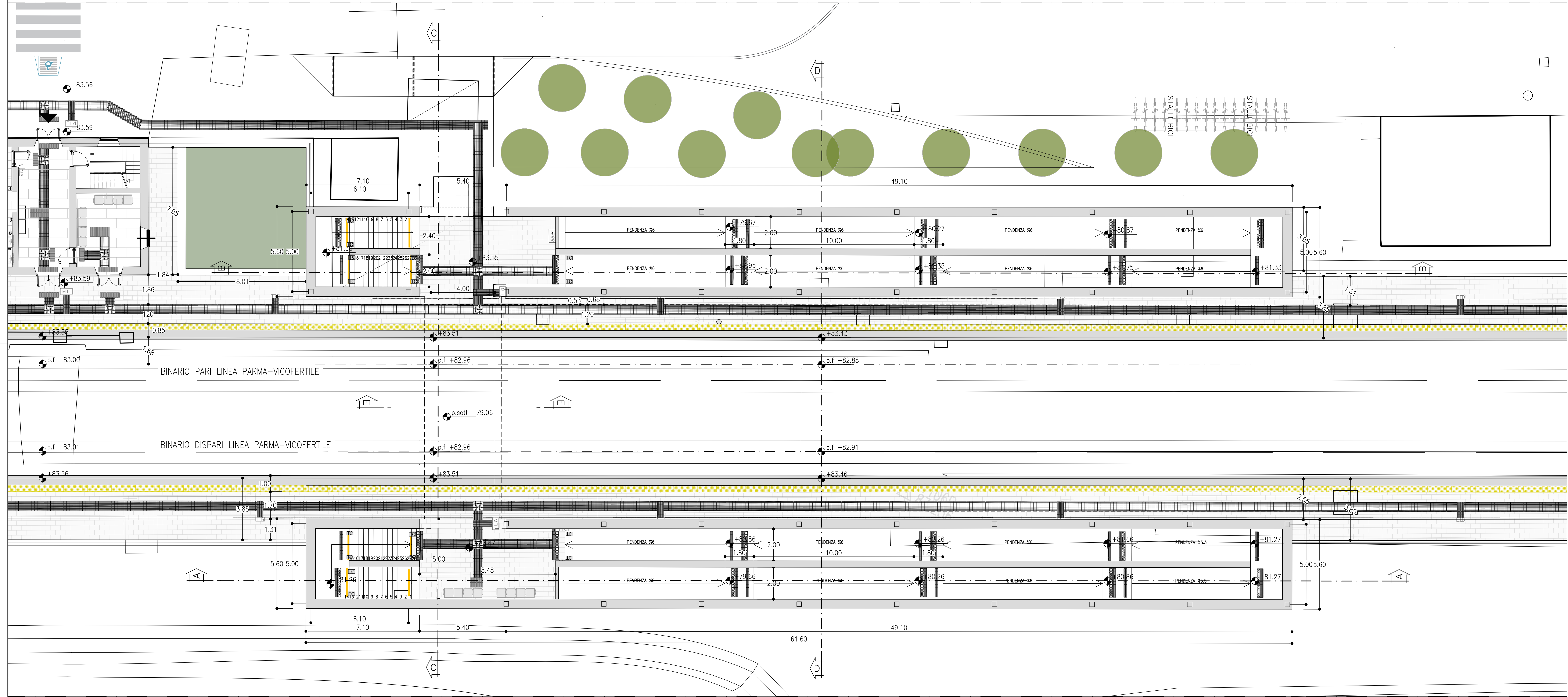
PIANTA QUOTA SOTTOPASSO SCALA 1:100
