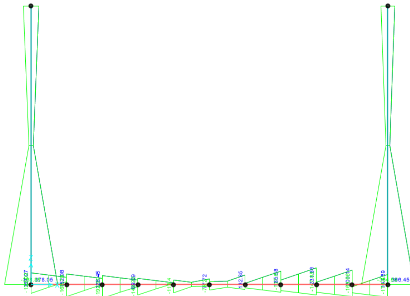
Fig. 15 – Involuppo SLU_Static – Sforzo di taglio
