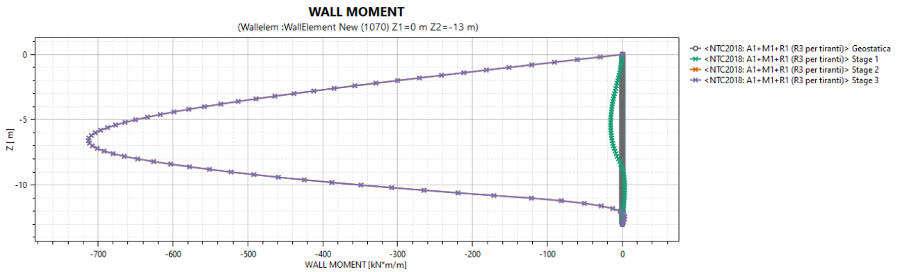
Figura 13 Andamento del momento flettente e taglio della diaframma sx in condizioni SLU e SLV per i vari fasi di calcolo (sulla condizione senza incastro soletta superiore, %0)
