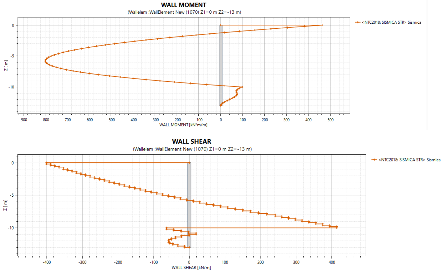
Figura 12 Andamento del momento flettente e taglio della diaframma dx in condizioni SLU e SLV per i vari fasi di calcolo (sulla condizione con incastro soletta superiore, %100)
