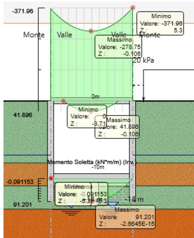
Figura 15 Andamento del momento flettente della soletta superiore in condizione SLU (sulla condizione con incastro soletta superiore).
