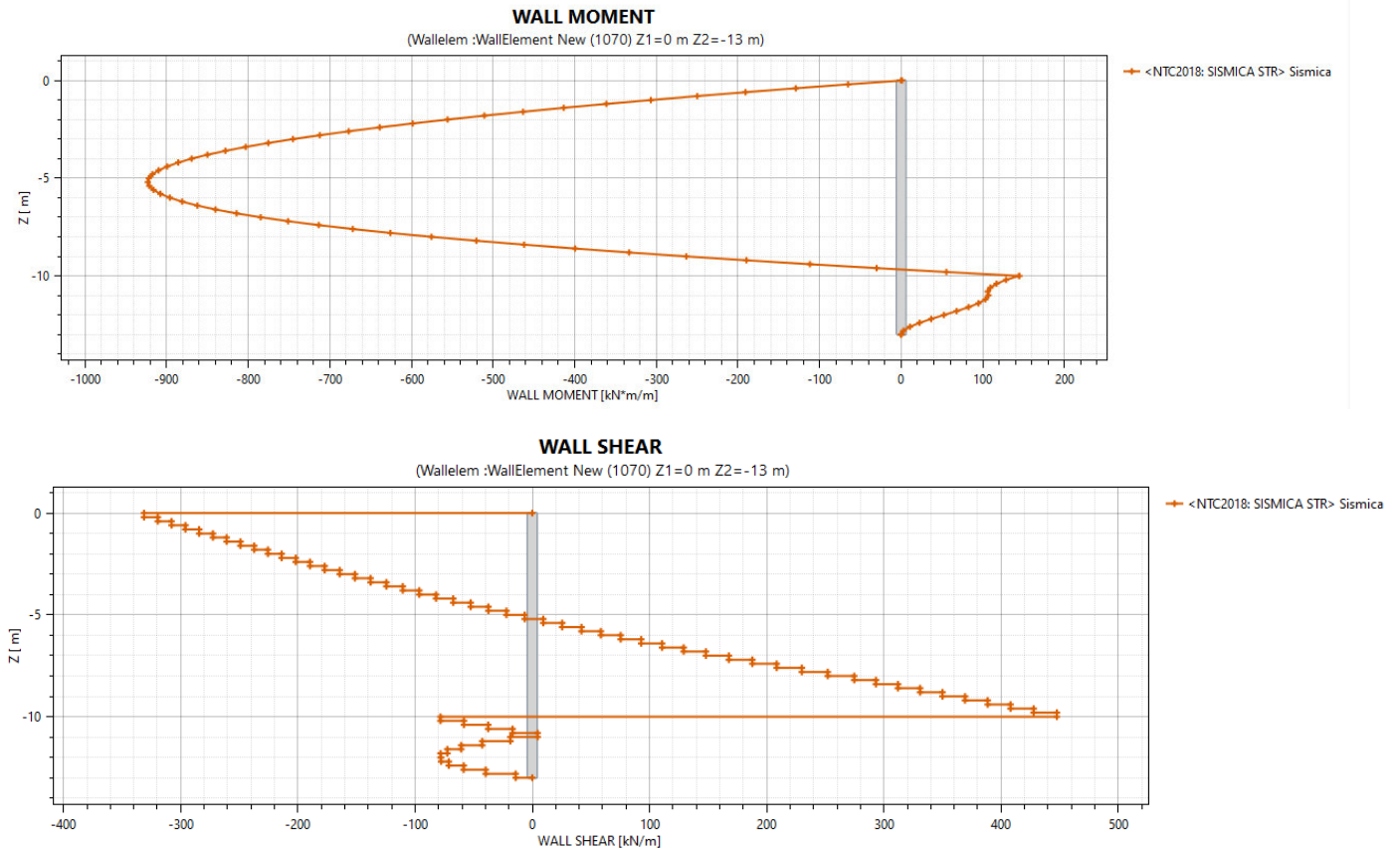
Figura 14 Andamento del momento flettente e taglio della diaframma dx in condizioni SLU e SLV per i vari fasi di calcolo (sulla condizione senza incastro soletta superiore, %0)
