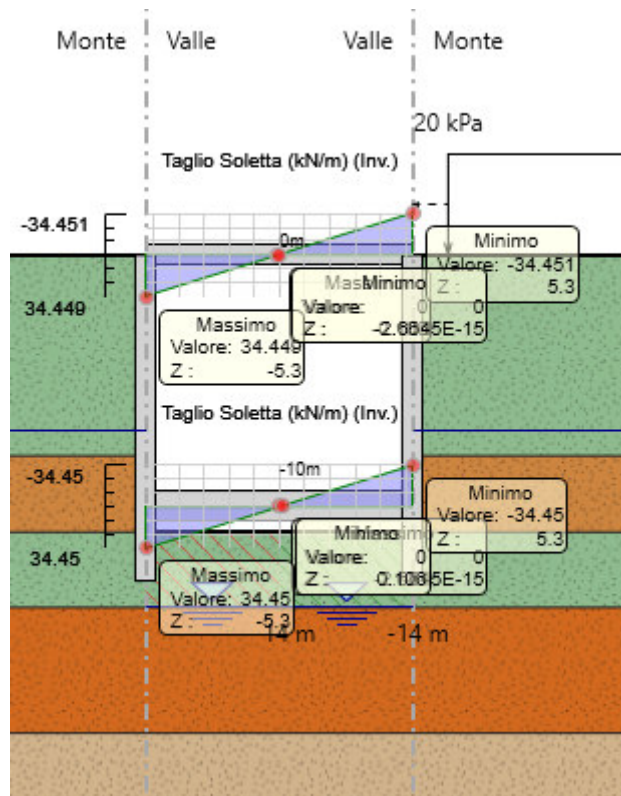
Figura 20 Andamento taglio della soletta superiore in condizione SLU (sulla condizione senza incastro soletta superiore).
