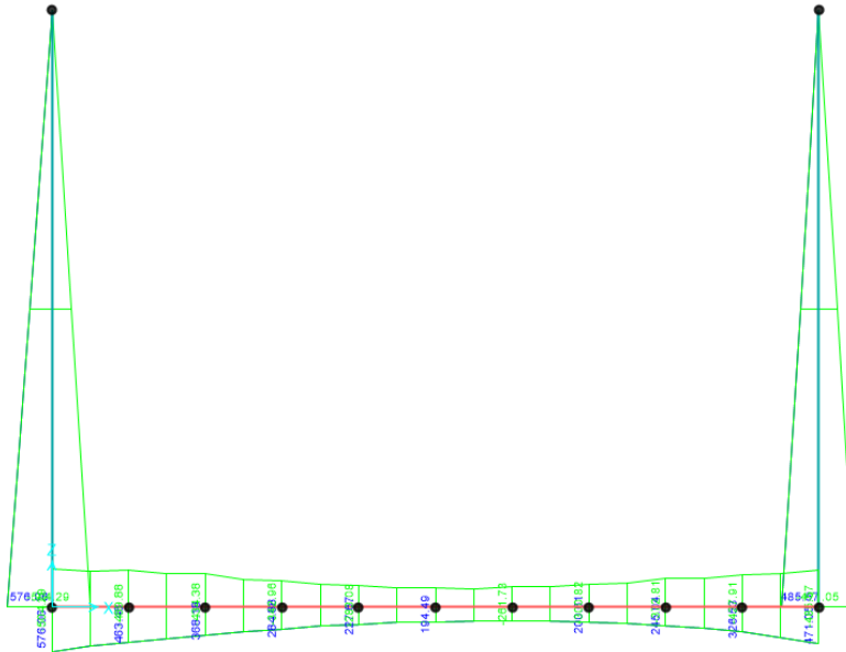
Fig. 14 – Involuppo SLU_Static – Momenti Flettenti
