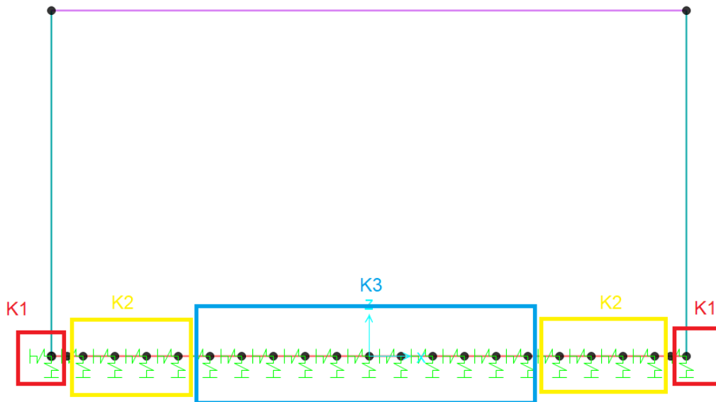
Fig. 8 – Vincoli alla base del modello di calcolo -tipico-
