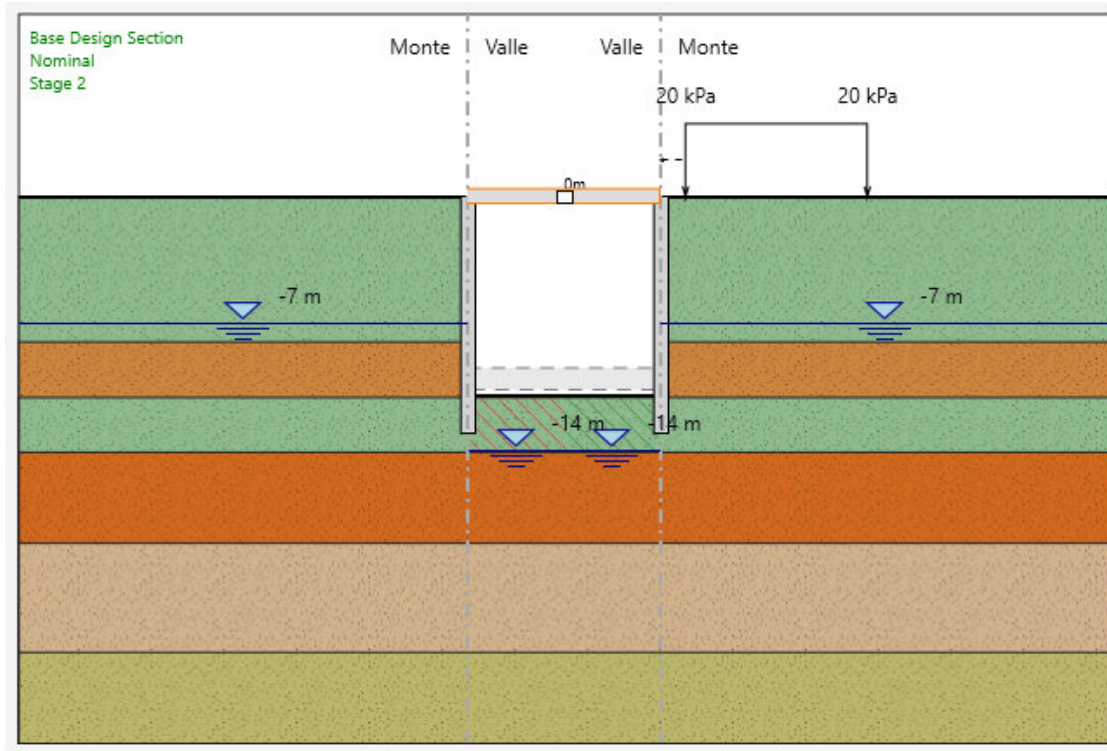
Figura 8 Scavo fino a quota -11m;
