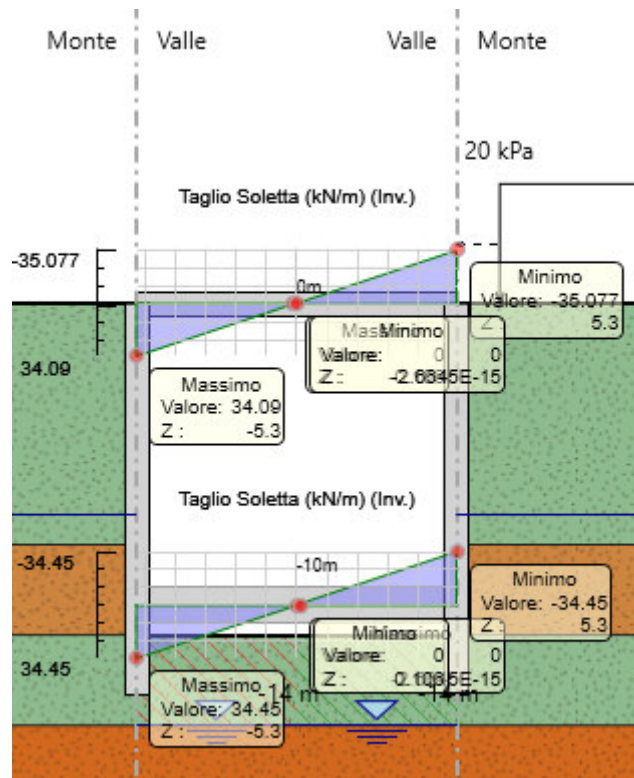
Figura 16 Andamento taglio della soletta superiore in condizione SLU (sulla condizione con incastro soletta superiore).
