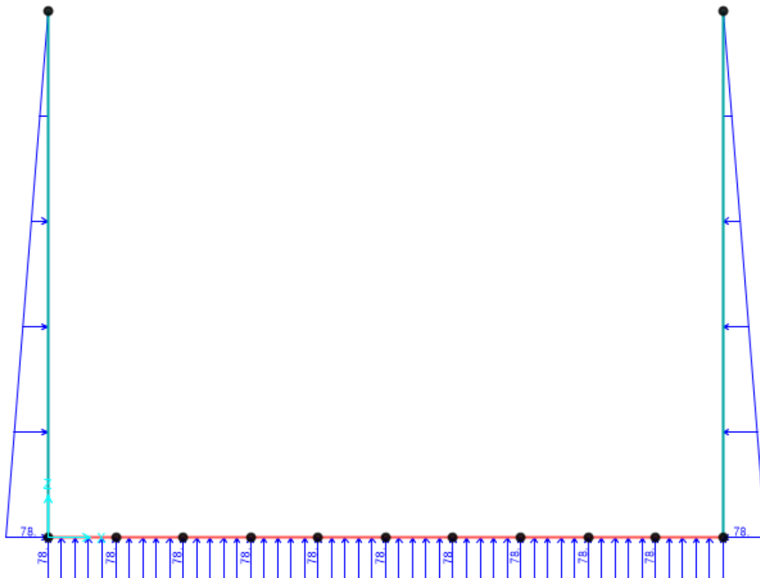
Figura 25 Q_{acqua\_ug} . effetti dell'acqua sotterranea
