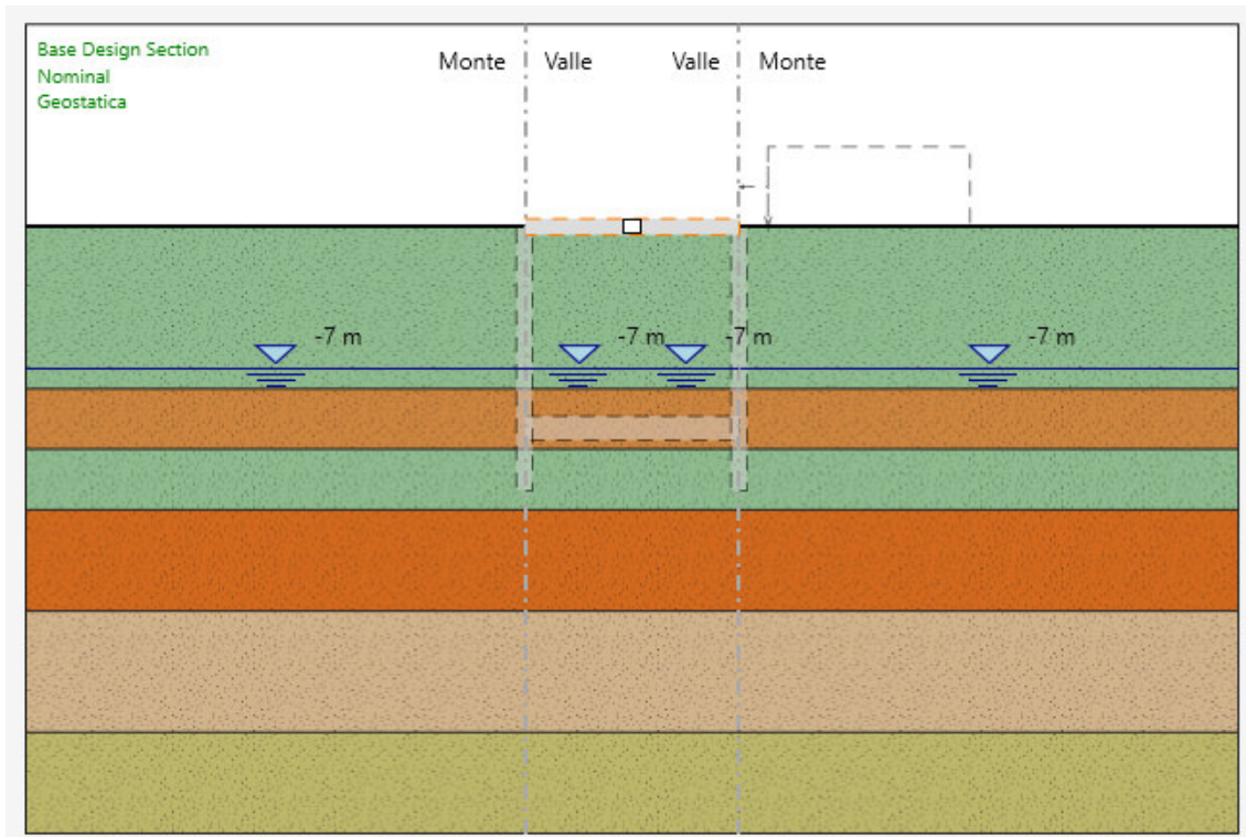
Figura 6: Inizializzazione geostatica;
