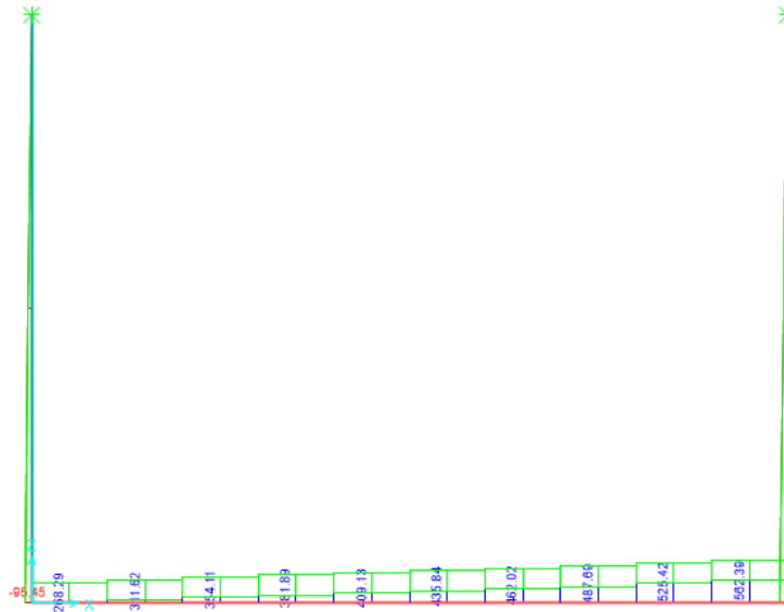
Fig. 22 – Involuppo SLV_Sismic – Sforzo Normale
