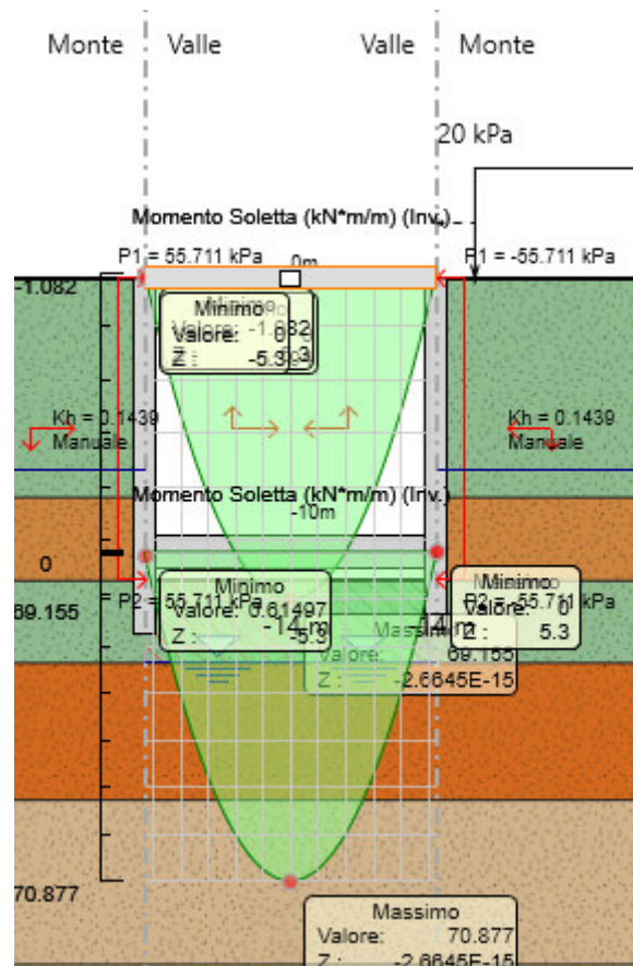
Figura 21 Andamento del momento flettente della soletta superiore in condizione SLV (sulla condizione senza incastro soletta superiore).
