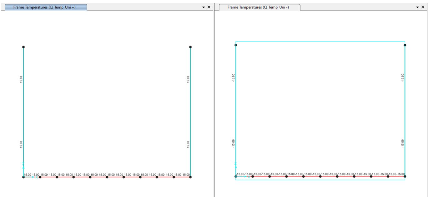
Fig. 10 – Q_Temp_Uni +/-: Forza termiche uniformi
