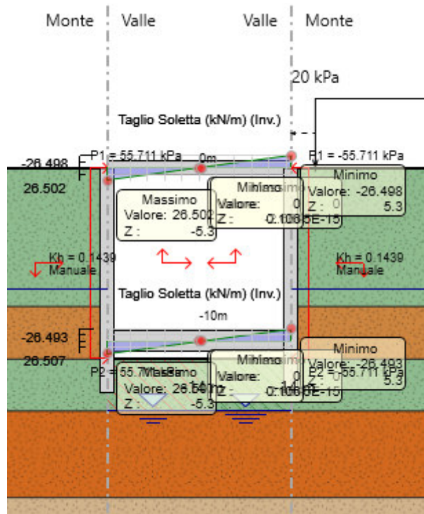
Figura 22 Andamento taglio della soletta superiore in condizione SLV (sulla condizione senza incastro soletta superiore).
