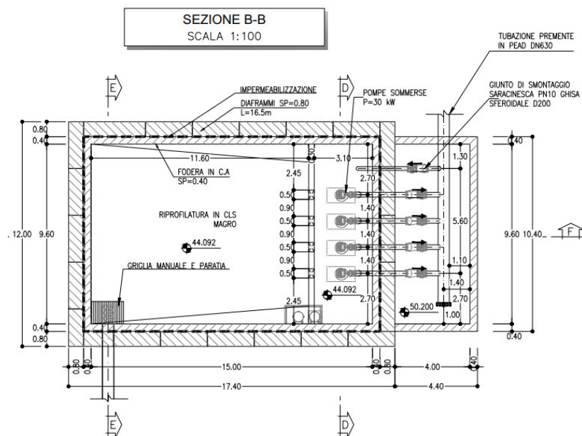
Fig. 3 – Sezione B-B
