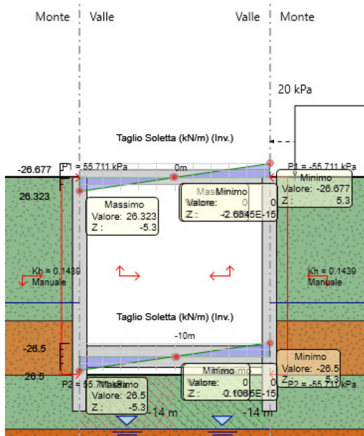
Figura 18 Andamento taglio della soletta superiore in condizione SLV (sulla condizione con incastro soletta superiore).
