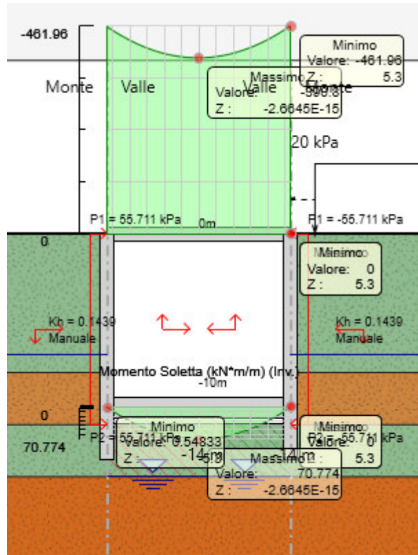
Figura 17 Andamento del momento flettente della soletta superiore in condizione SLV (sulla condizione con incastro soletta superiore).
