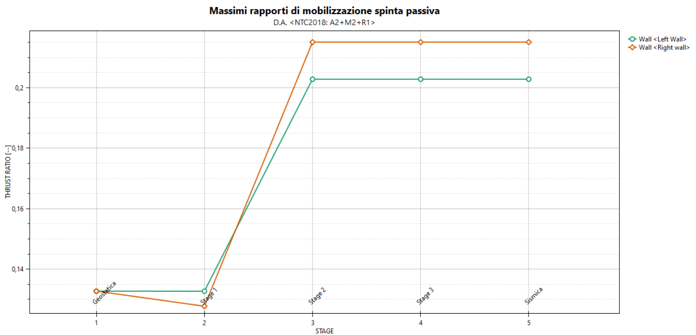
Figura 23 Rapporto di mobilitazione della spinta passiva.
