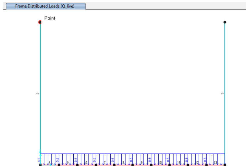
Figura 26 Q_{live} carico di manutenzione
