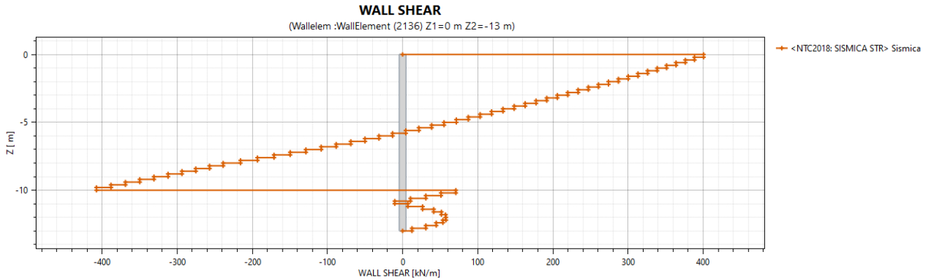
Figura 11 Andamento del momento flettente e taglio della diaframma sx in condizioni SLU e SLV per i vari fasi di calcolo (sulla condizione con incastro soletta superiore, %100)
