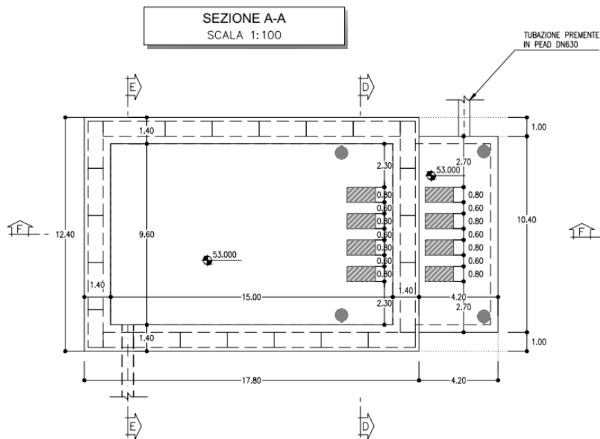
Fig. 2 – Sezione A-A
