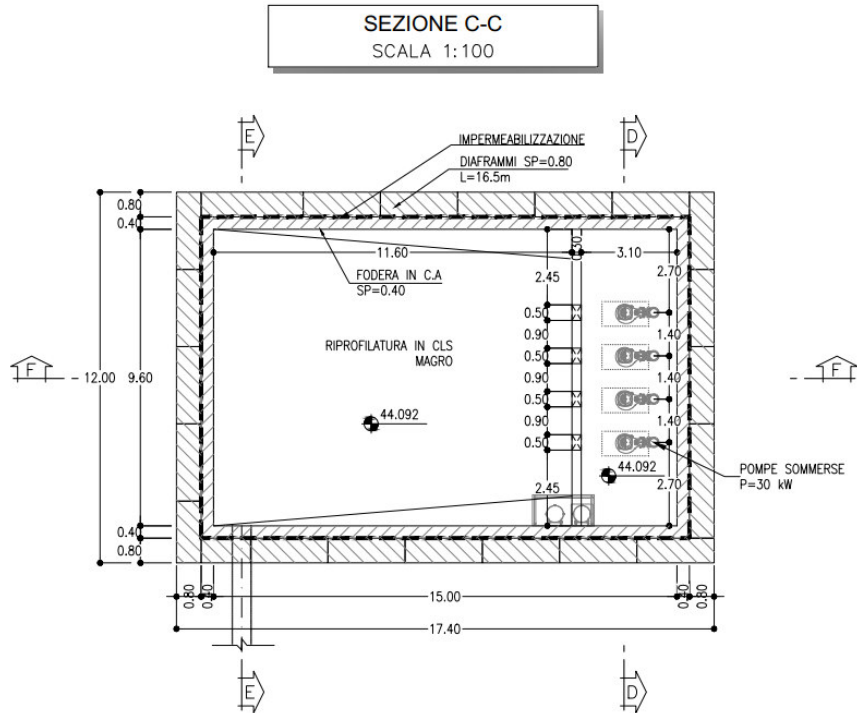
Fig. 4 – Sezione C-C
