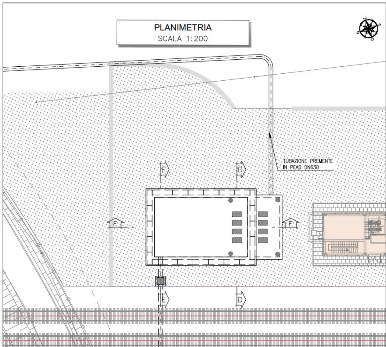
Fig. 1 – Planimetria generale
