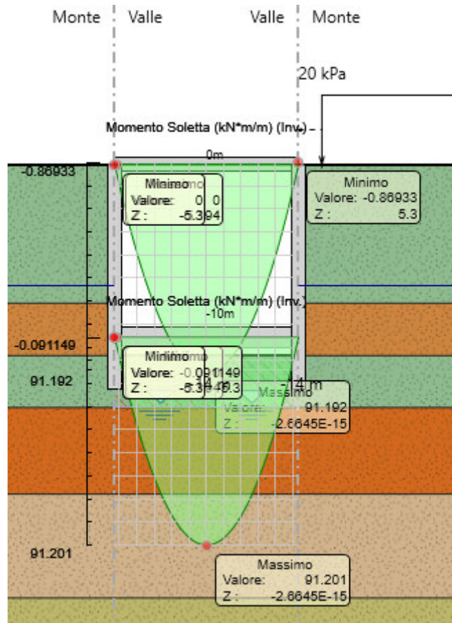
Figura 19 Andamento del momento flettente della soletta superiore in condizione SLU (sulla condizione senza incastro soletta superiore).
