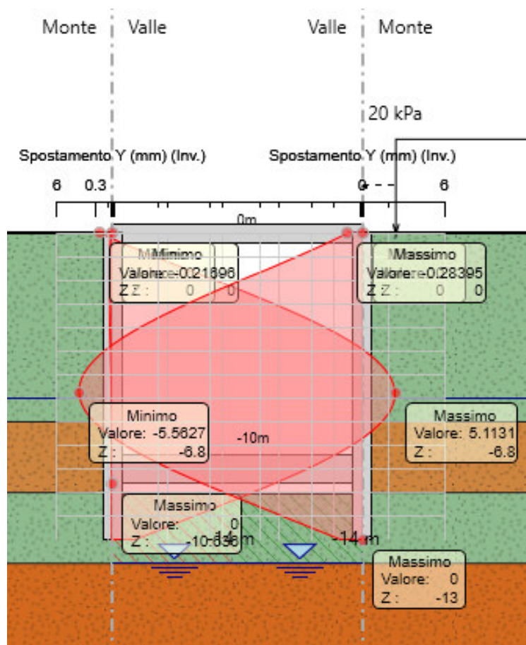
Figura 24 Inviluppo spostamenti SLE.
