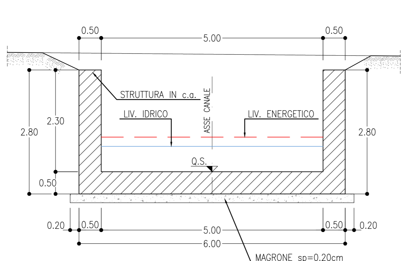
DEVIATIONE - SEZIONE TIPO SCALA 1:50
