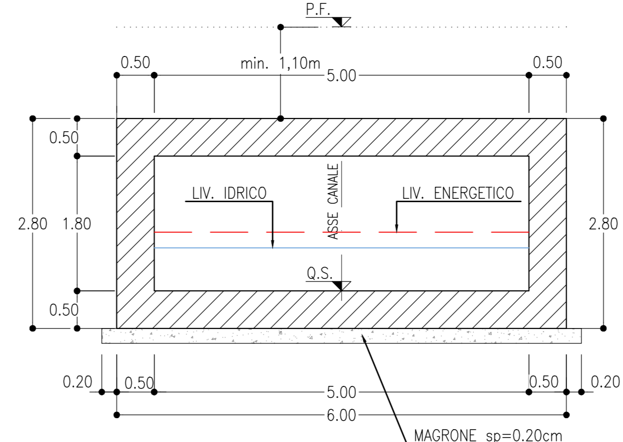
TOMBINO SCATOLARE - SEZIONE TIPO SCALA 1:50
