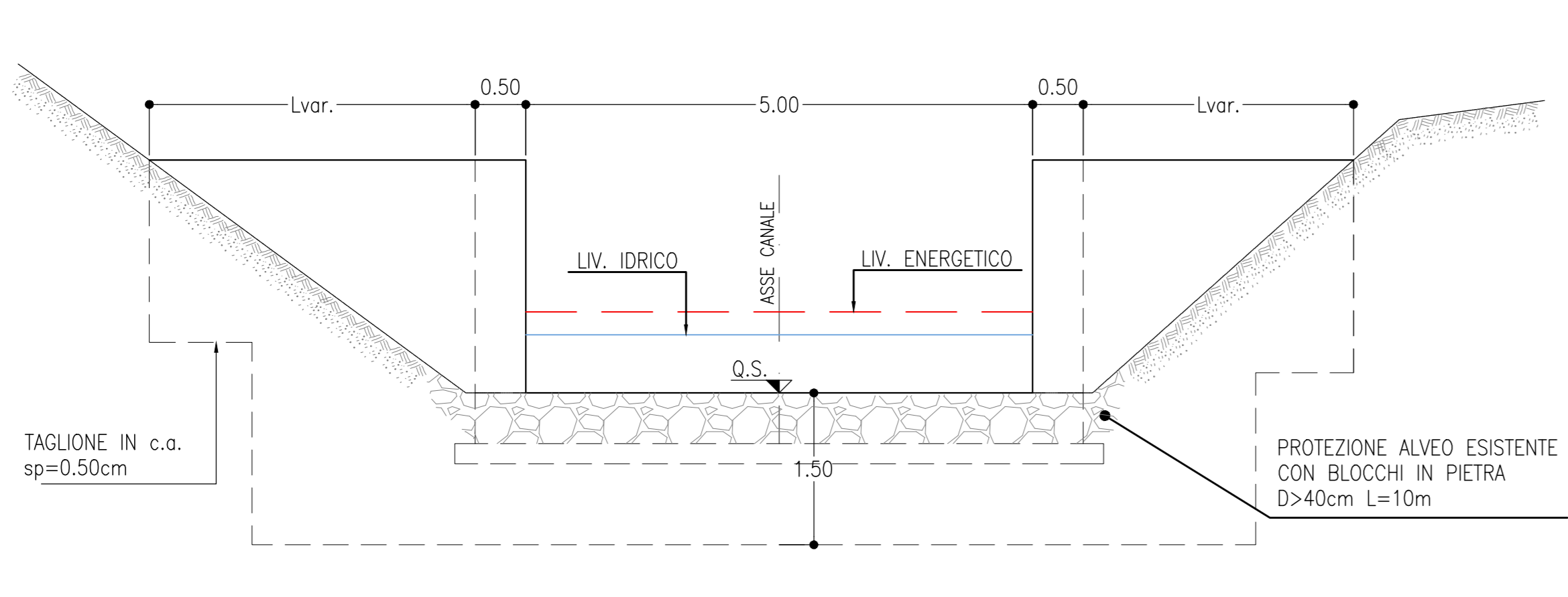
TAGLIONE DI AMMORSAMENTO - SEZIONE TIPO SCALA 1:50
