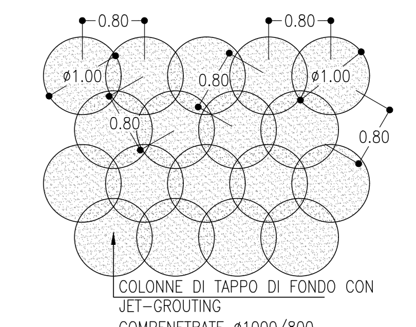
DISPOSIZIONE DEGLI ELEMENTI DI JET-GROUTING SCALA 1:50
