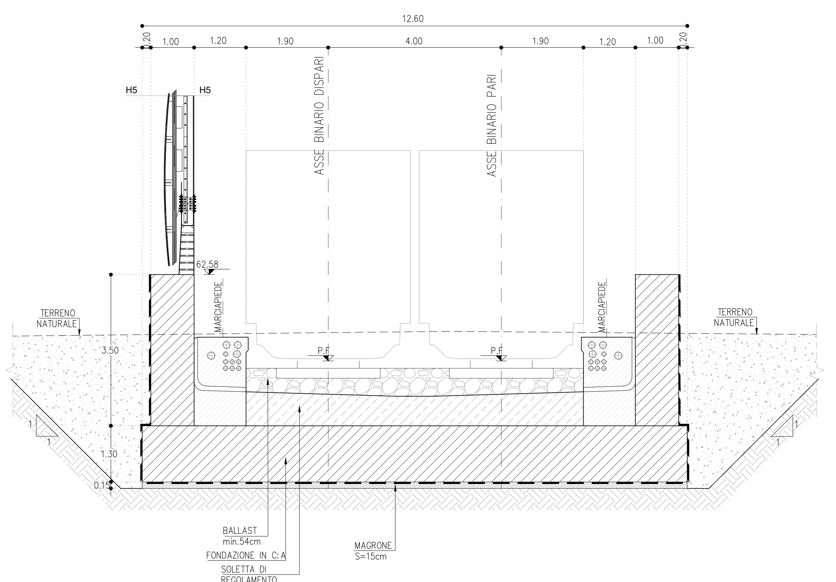
MURO AD U IN TRINCEA SCALA 1:50 SEZIONE TRASVERSALE SEZIONE DOPPIO BINARIO TRO5
