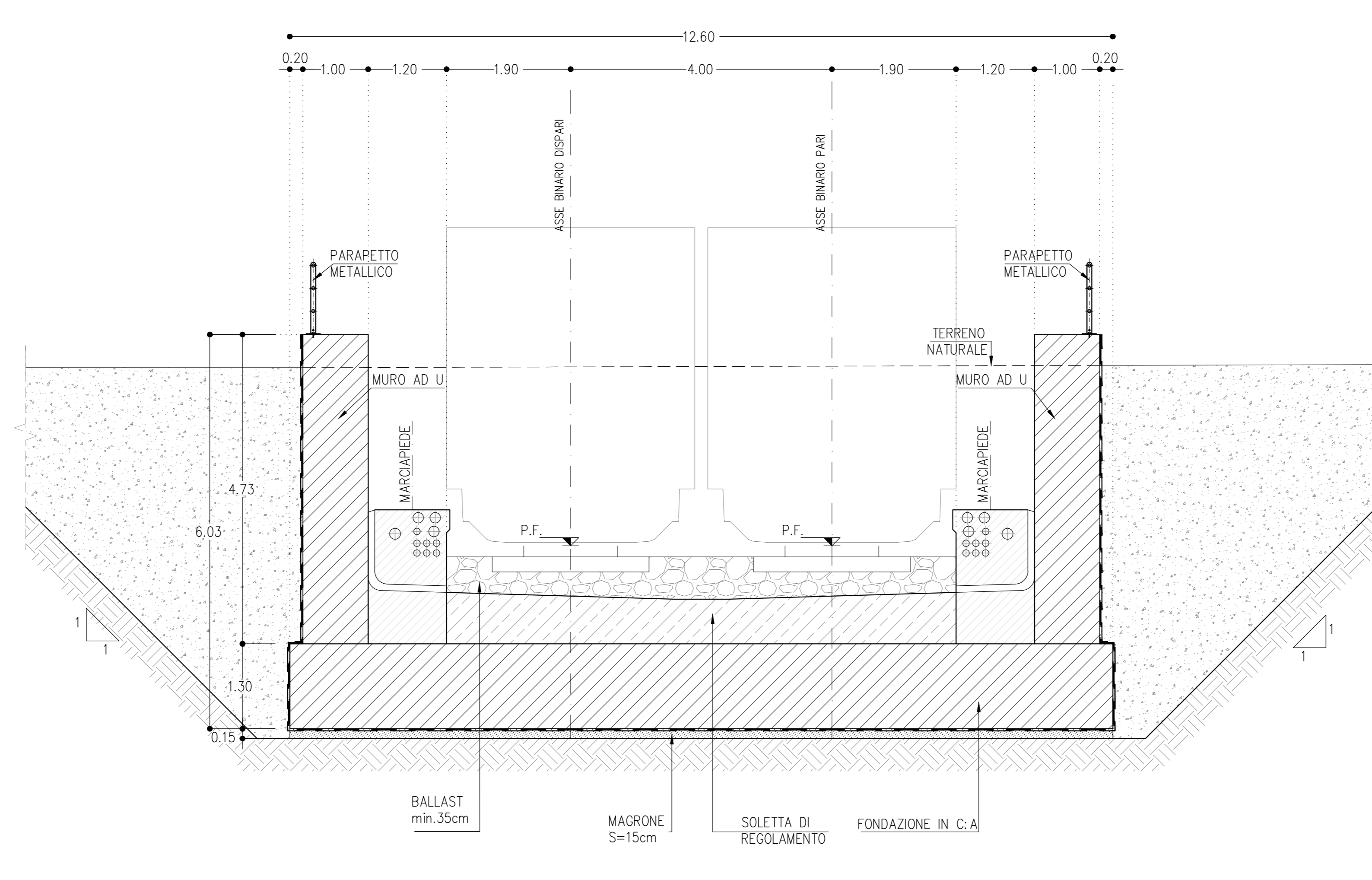
MURO AD U IN TRINCEA SCALA 1:50 SEZIONE TRASVERSALE SEZIONE DOPPIO BINARIO TRO4B
