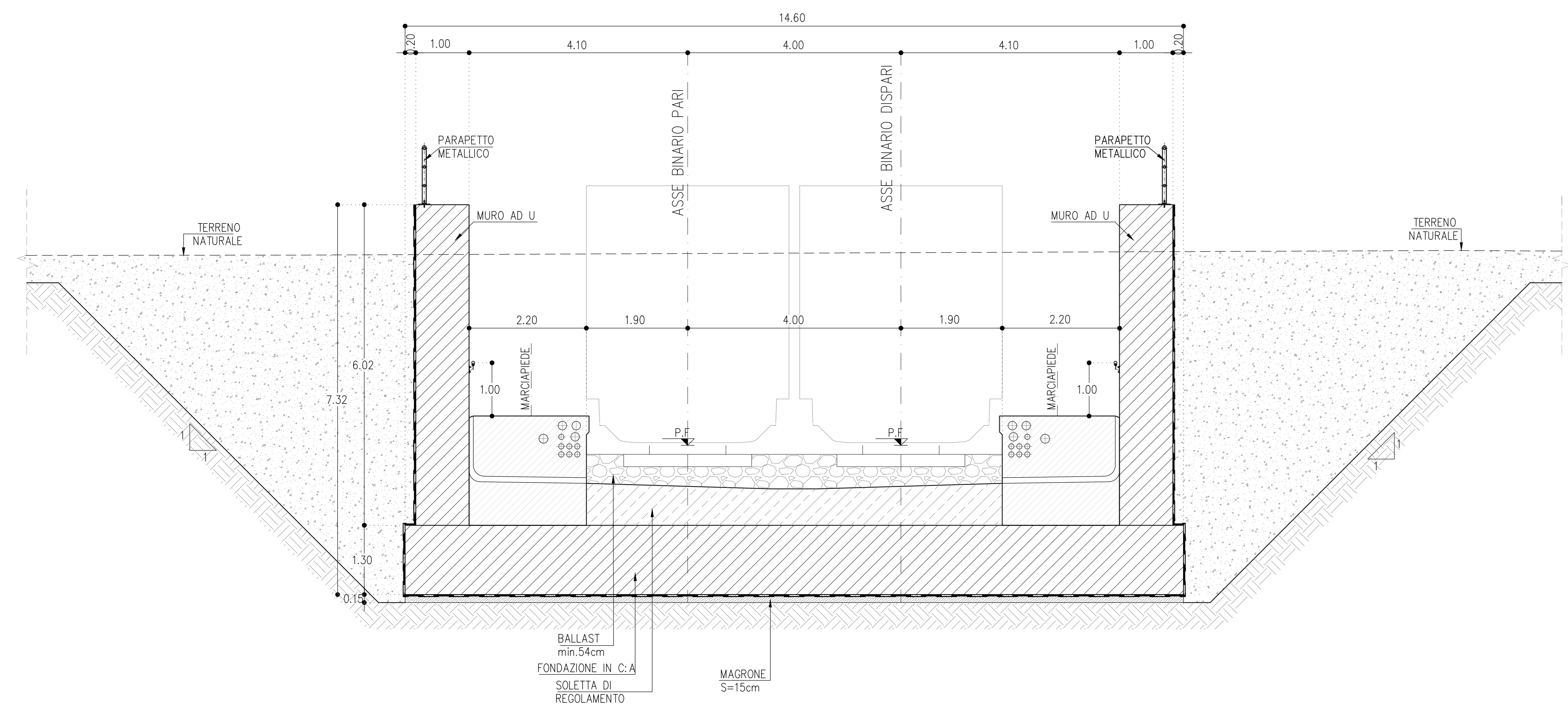
MURO AD U IN TRINCEA SCALA 1:50 SEZIONE TRASVERSALE SEZIONE DOPPIO BINARIO TRO4A
