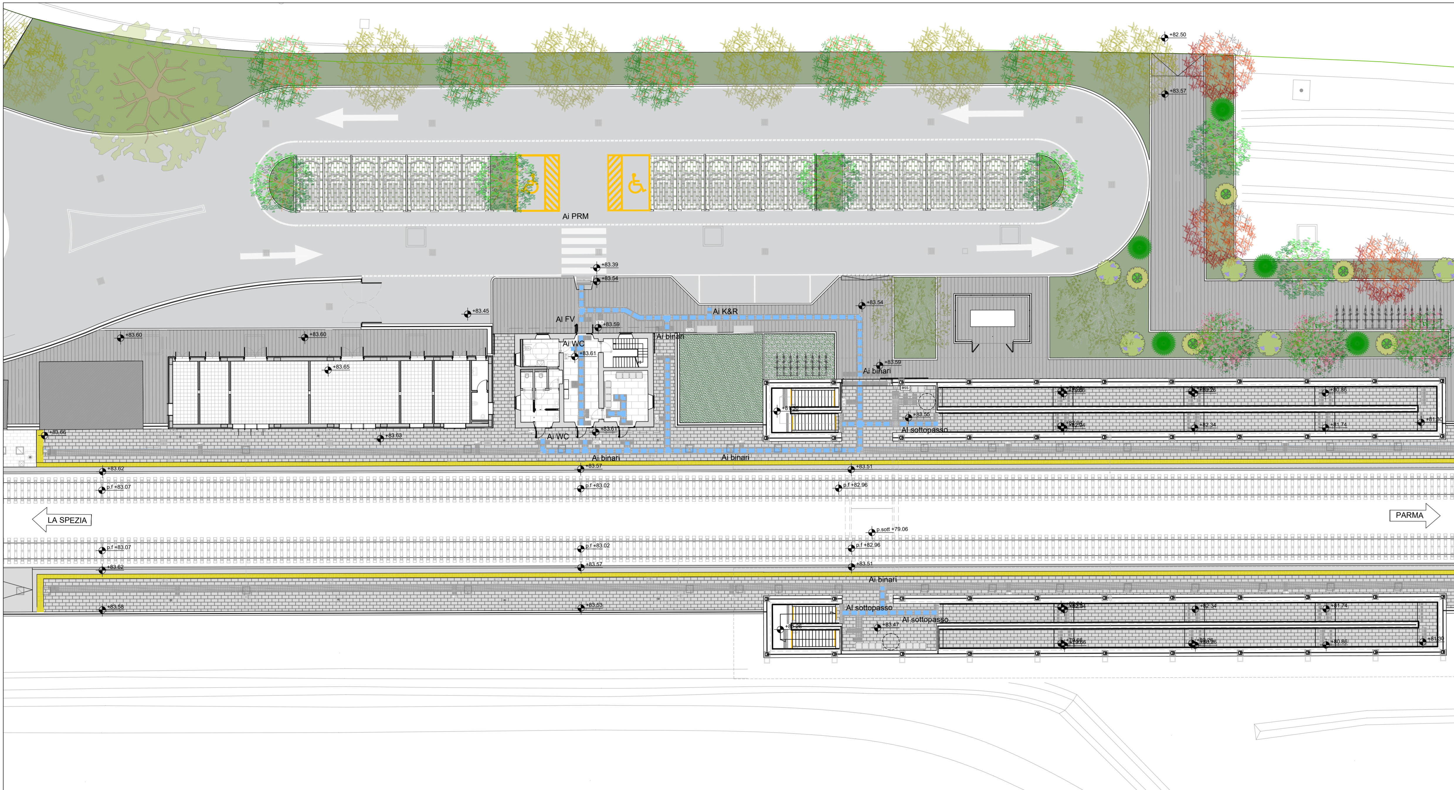
PIANTA QUOTA BANCHINA scala 1:200
