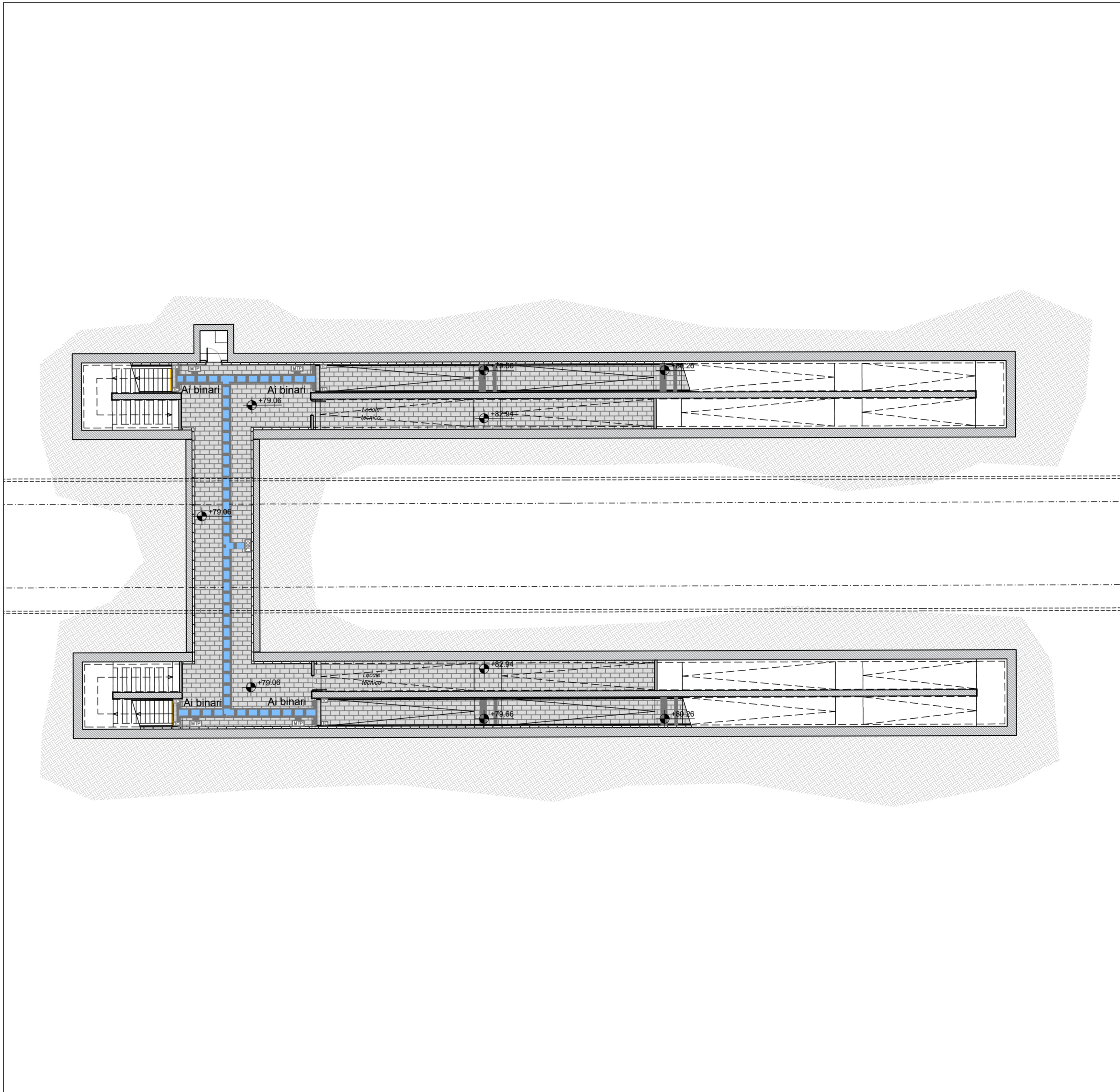
PIANTA SOTTOPASSO scala 1:200
