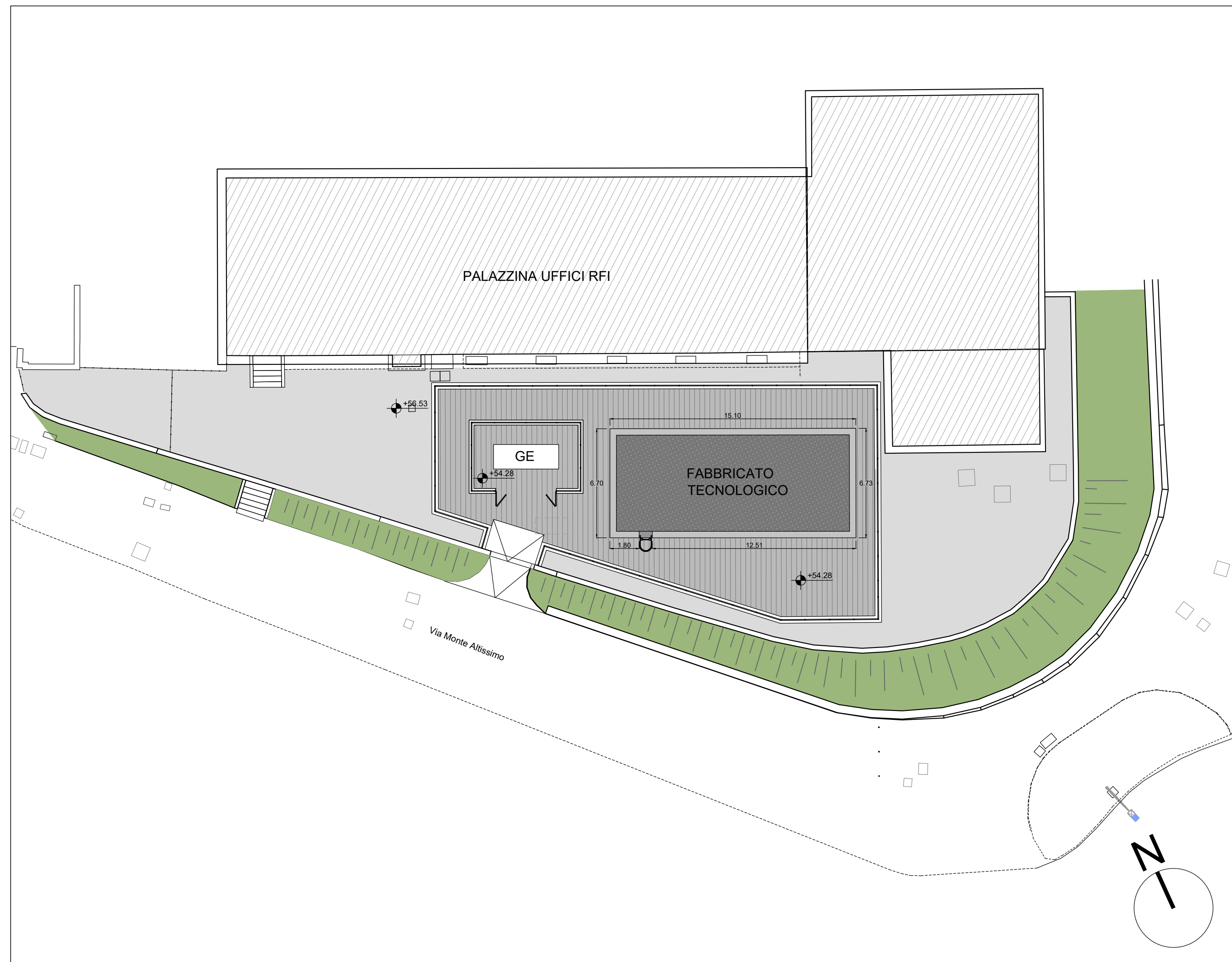
PIANTA QUOTA COPERTURE scala 1:200
