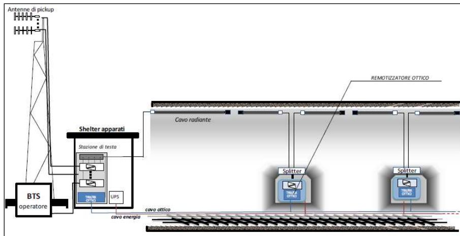
Figura 3: impianto di tipo elettro ottico
