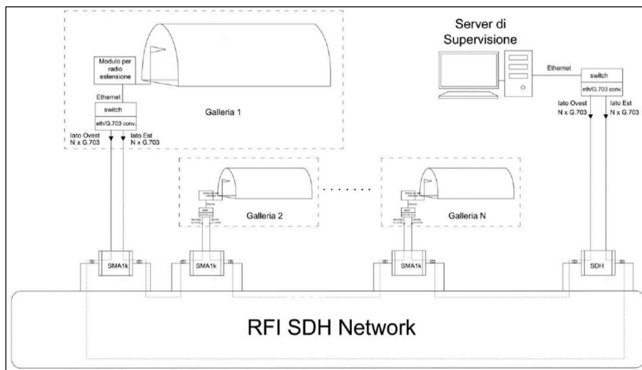
Figura 1: Schematico di Rete sistema di supervisione centrale
