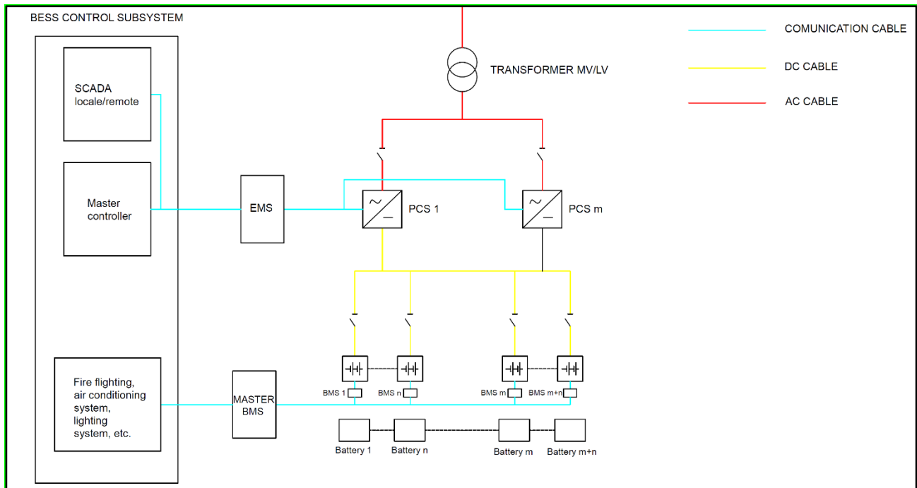
Figura 4.1: Schema di funzionamento del BESS
