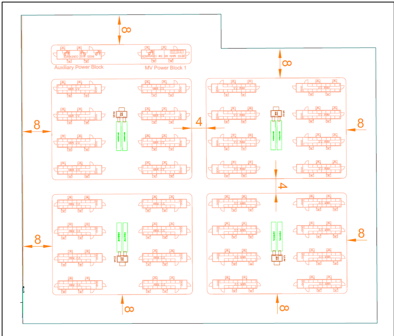
Figura 1.1: Planimetria del progetto preliminare del BESS (ALL 1)
