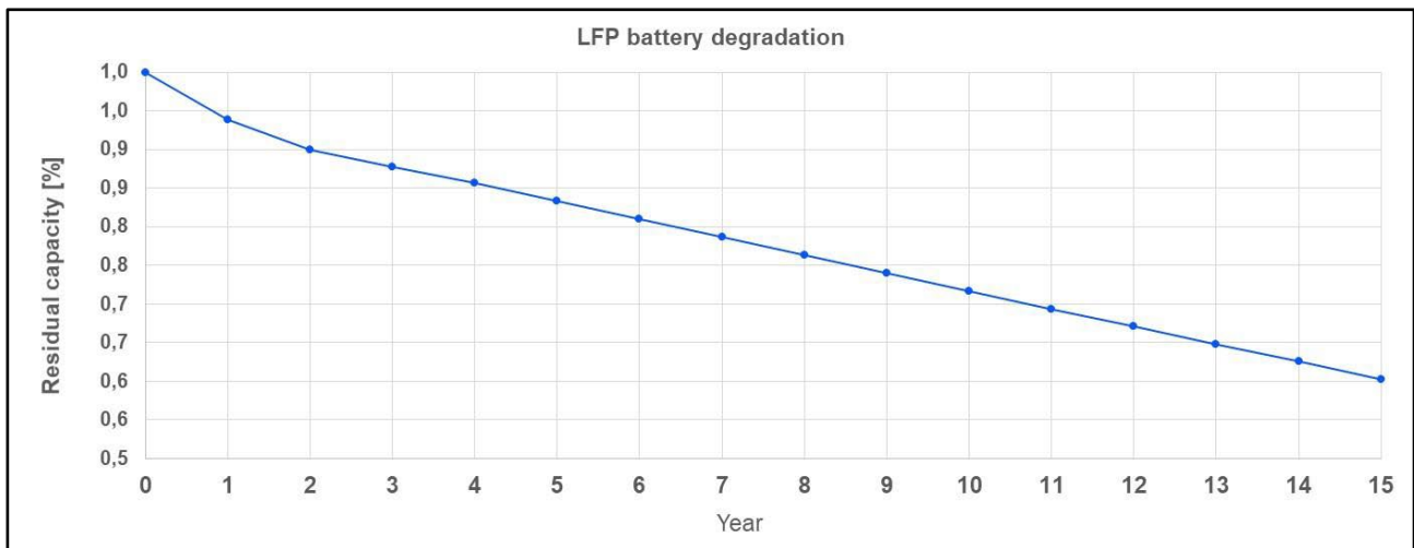
Figura 12.1: Decadimento tecnico del sistema di accumulo (BESS)
