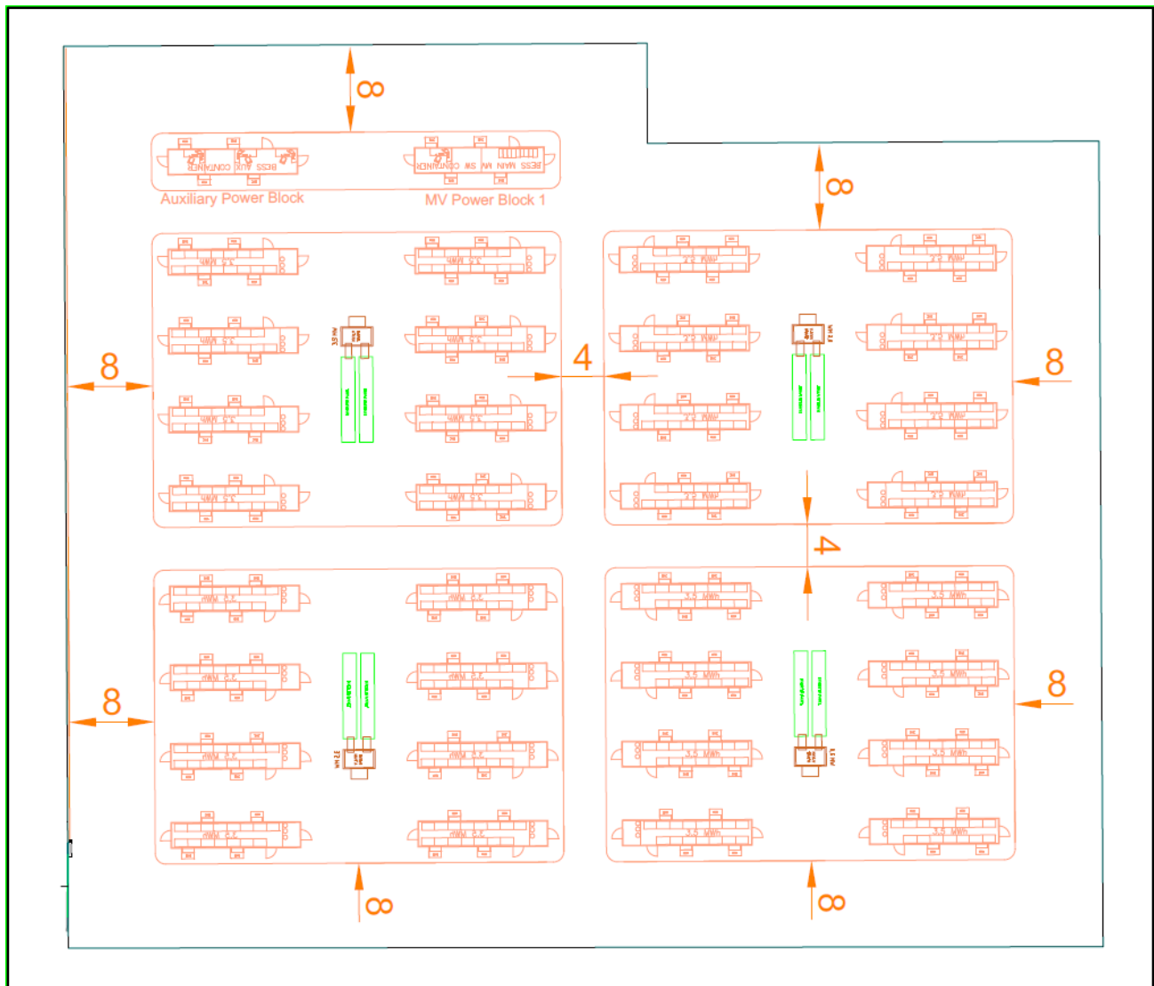
Figura 9.1.3: Esempio di configurazione BESS di potenza 14 MWp
