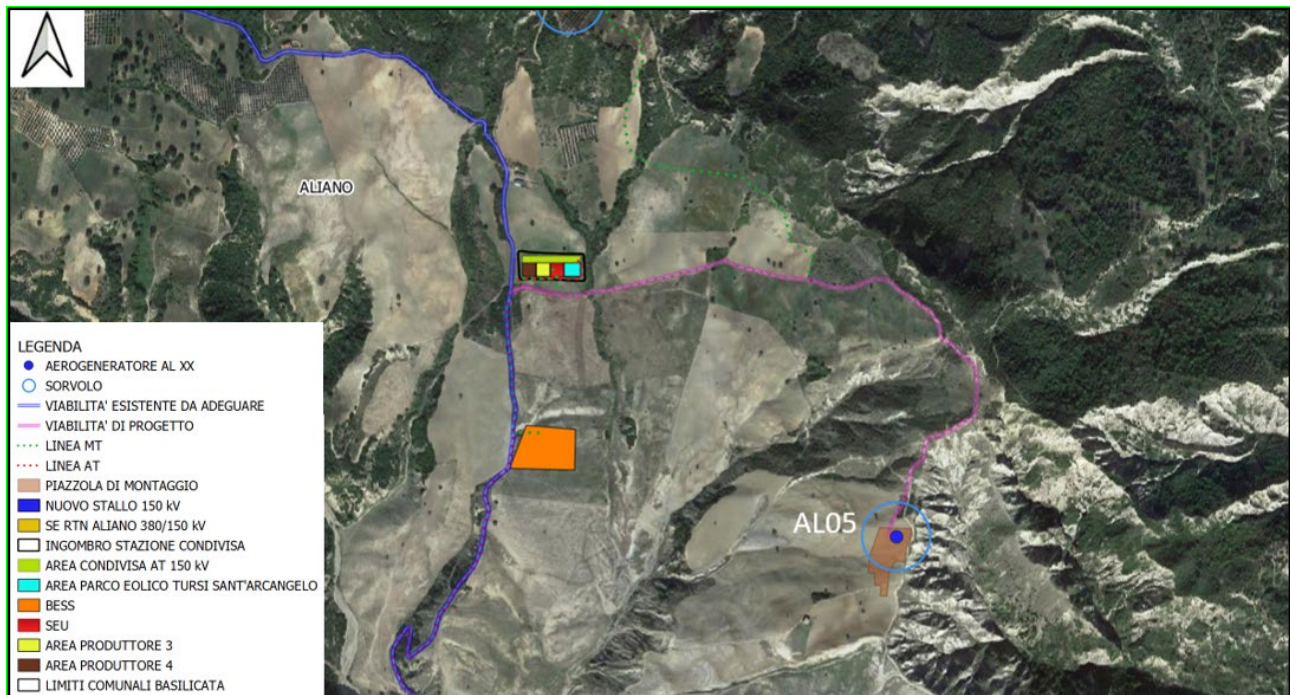
Figura 9.1.1: Localizzazione SEU 150/33 kV e BESS su ortofoto
