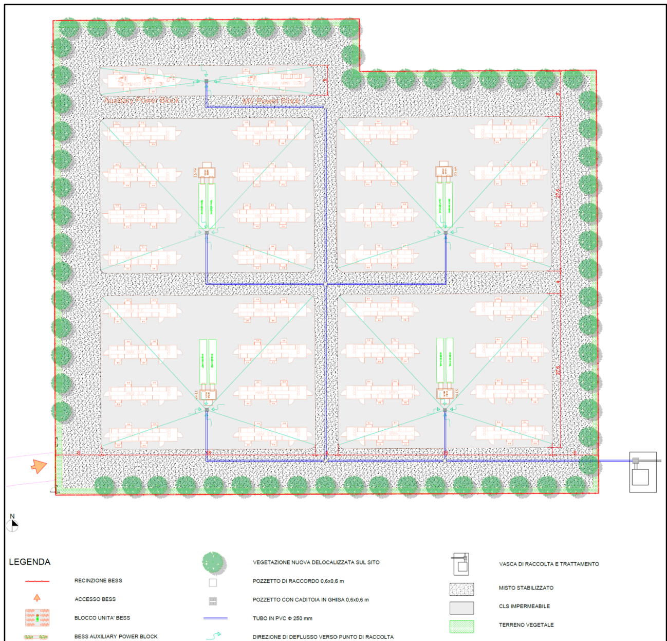
Figura 11.1: Planimetria architettonica BESS con sistema di smaltimento acque
