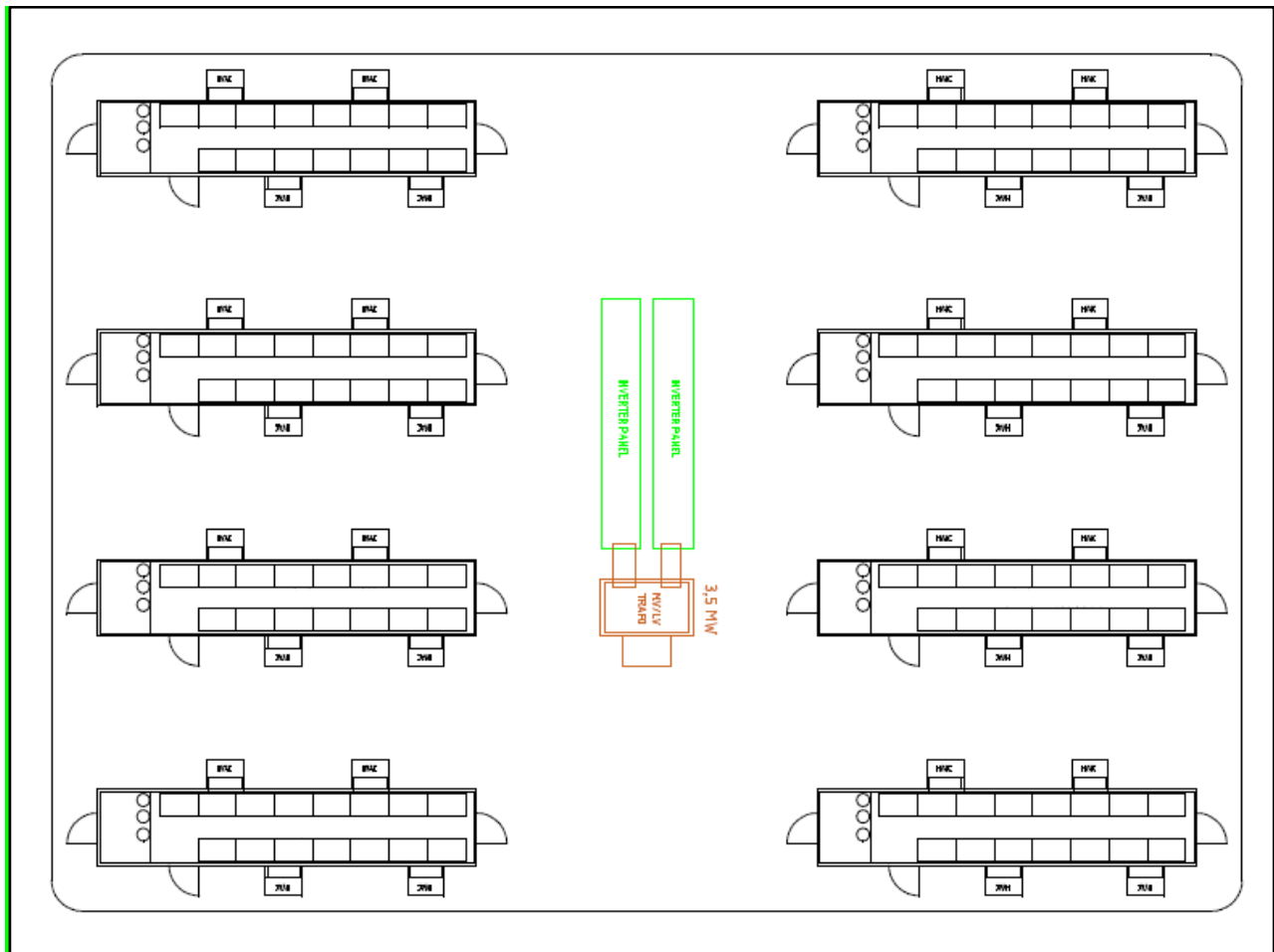
Figura 9.1.2: Unità base da 3.5 MW del BESS
