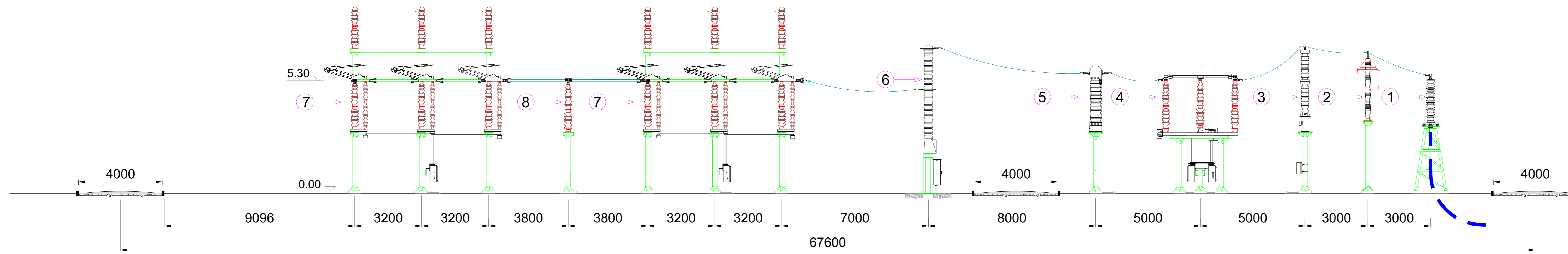
Stallo arrivo in cavo 220 kV - Scala 1:100
