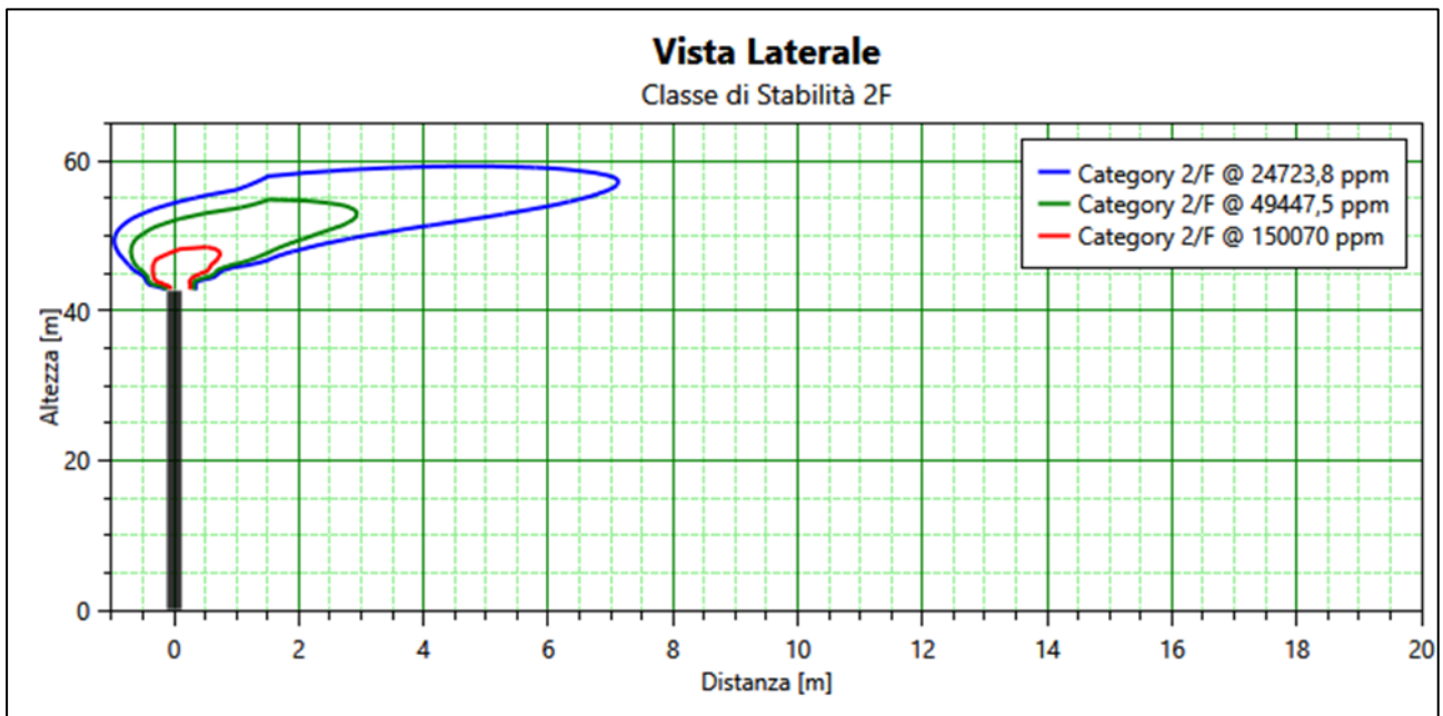
Figura 6 - Dispersione nube infiammabile - Classe Meteo 2F
