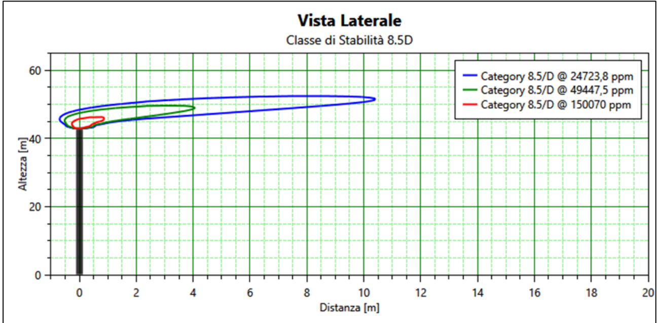
Figura 8 - Dispersione nube infiammabile - Classe Meteo 8.5D
