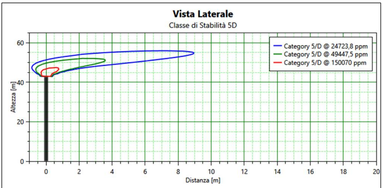
Figura 7 - Dispersione nube infiammabile - Classe Meteo 5D
