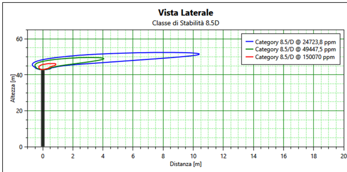
Figura 4 - Dispersione nube infiammabile - Classe Meteo 8.5 D
