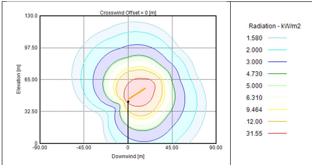
Figura 3 - Mappa di irraggiamento – Vista Frontale
