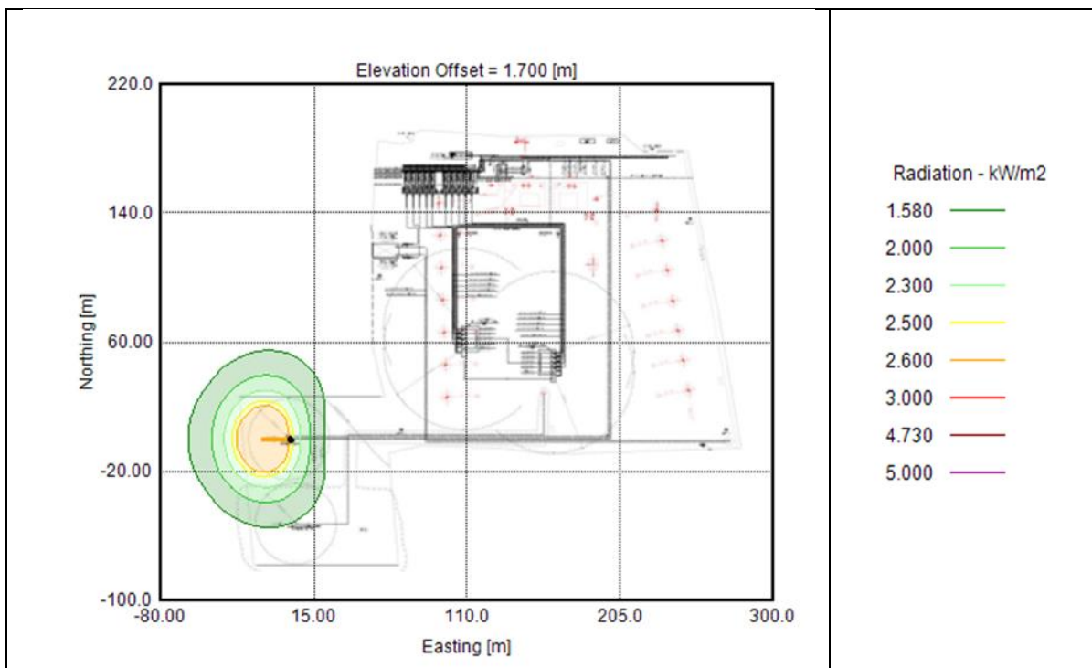
Figura 2 - Mappa di irraggiamento - Pianta
