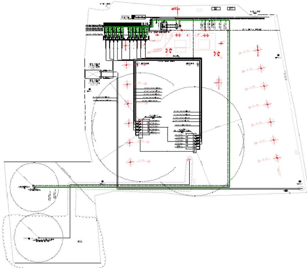
Figura 5- Planimetria andamento tubazioni- Collettore per BDV e PSV
