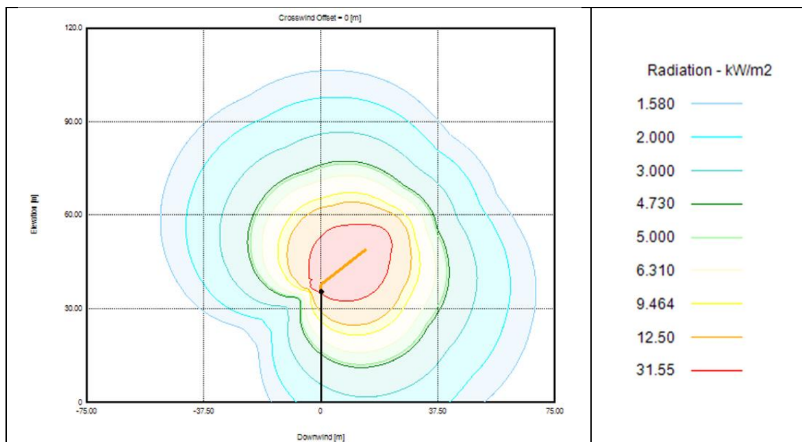
Figura 3 - Mappa di irraggiamento – Vista Frontale
