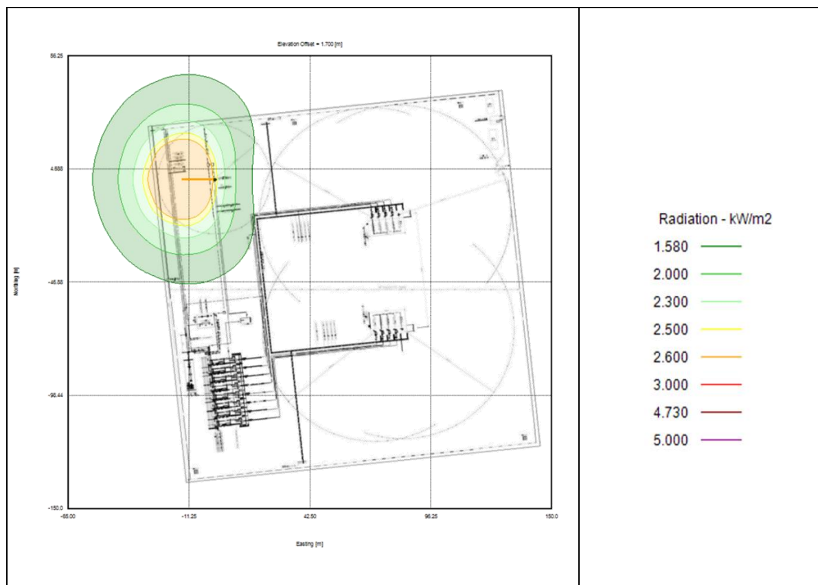
Figura 2 - Mappa di irraggiamento - Pianta
