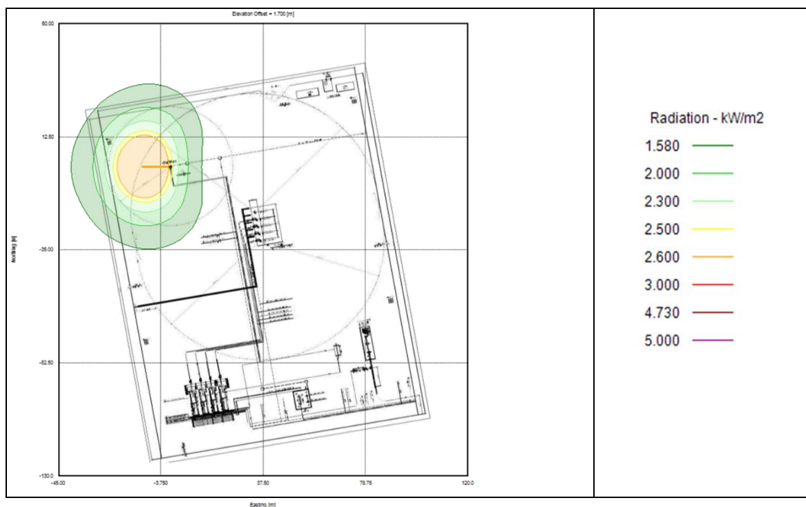
Figura 2 - Mappa di irraggiamento - Pianta
