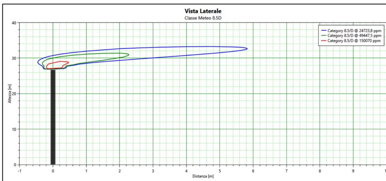
Figura 4 - Dispersione nube infiammabile - Classe Meteo 8.5D
