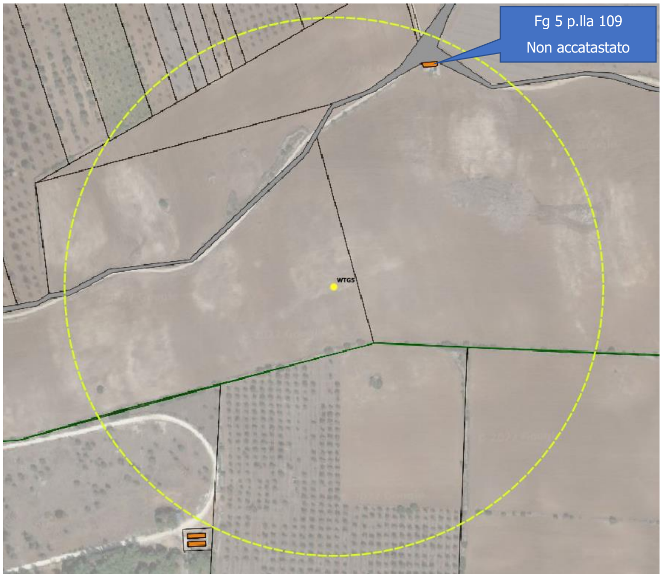
Figure 6 Particolare WTG05
