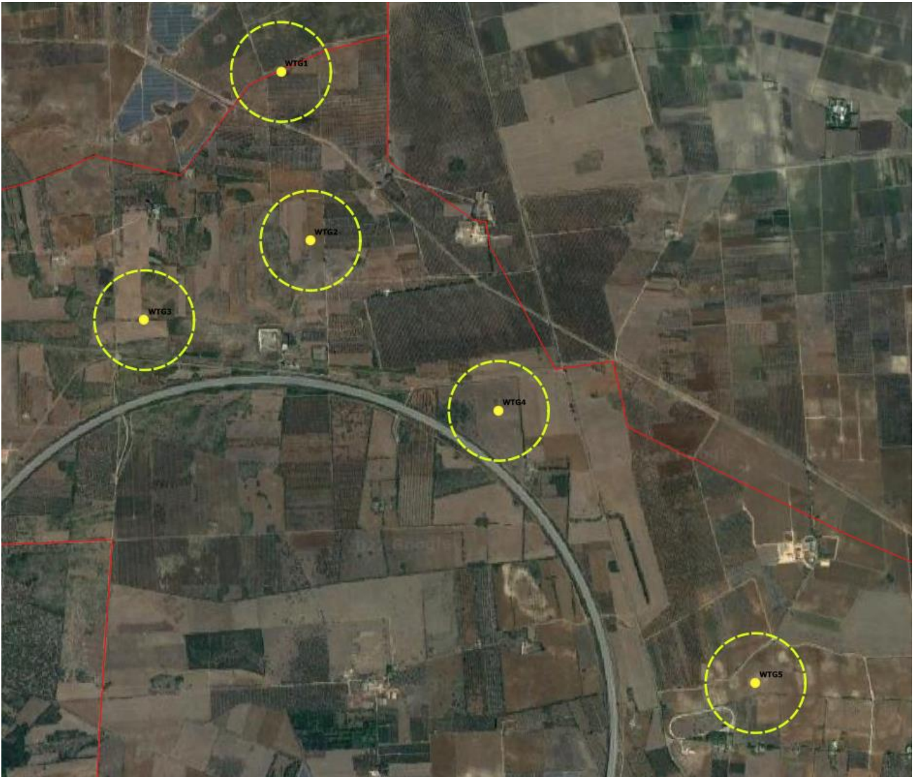
Figura 1 – Indicazione della gittata massima della pala in caso di distacco
