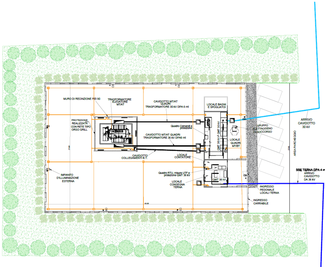
Figura 3-5: Stazione elettrica utente – schema planimetrico
