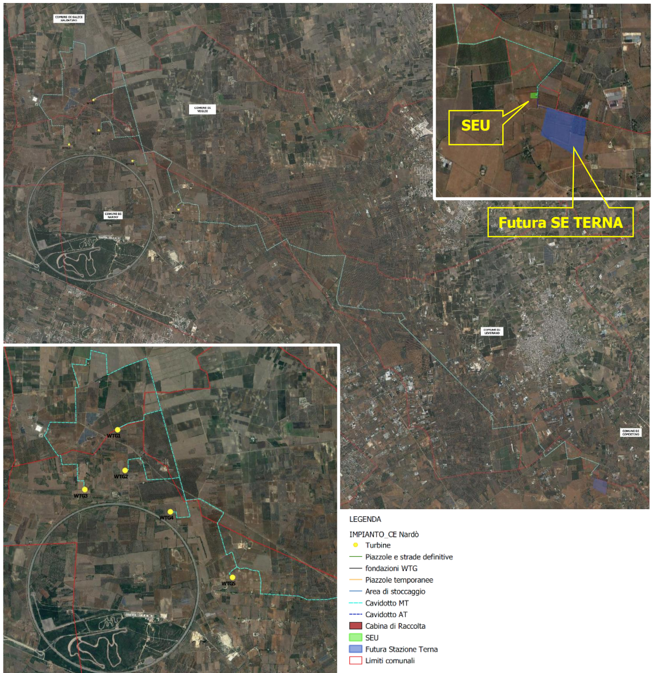
Figura 21: Layout parco eolico e opere di connessione
