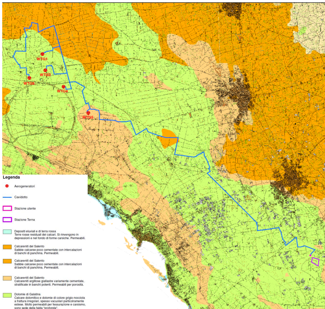
Figura 6-1: Stralcio Carta Geologica
