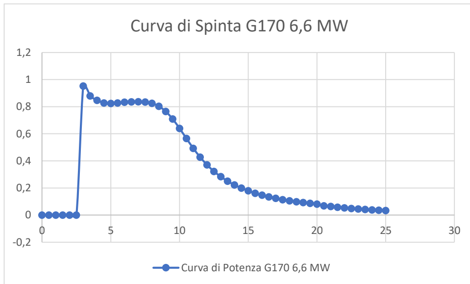
Figura 2 - Curva di spinta Gamesa G170 6,6 MW.
