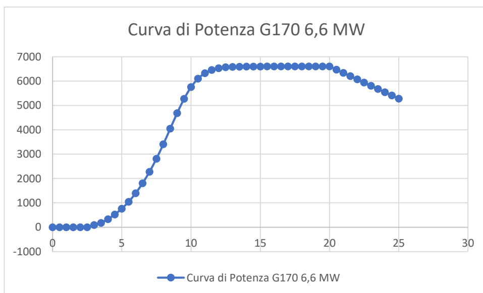
Figura 1 - Curva di potenza Gamesa SG170 6,6 MW.
