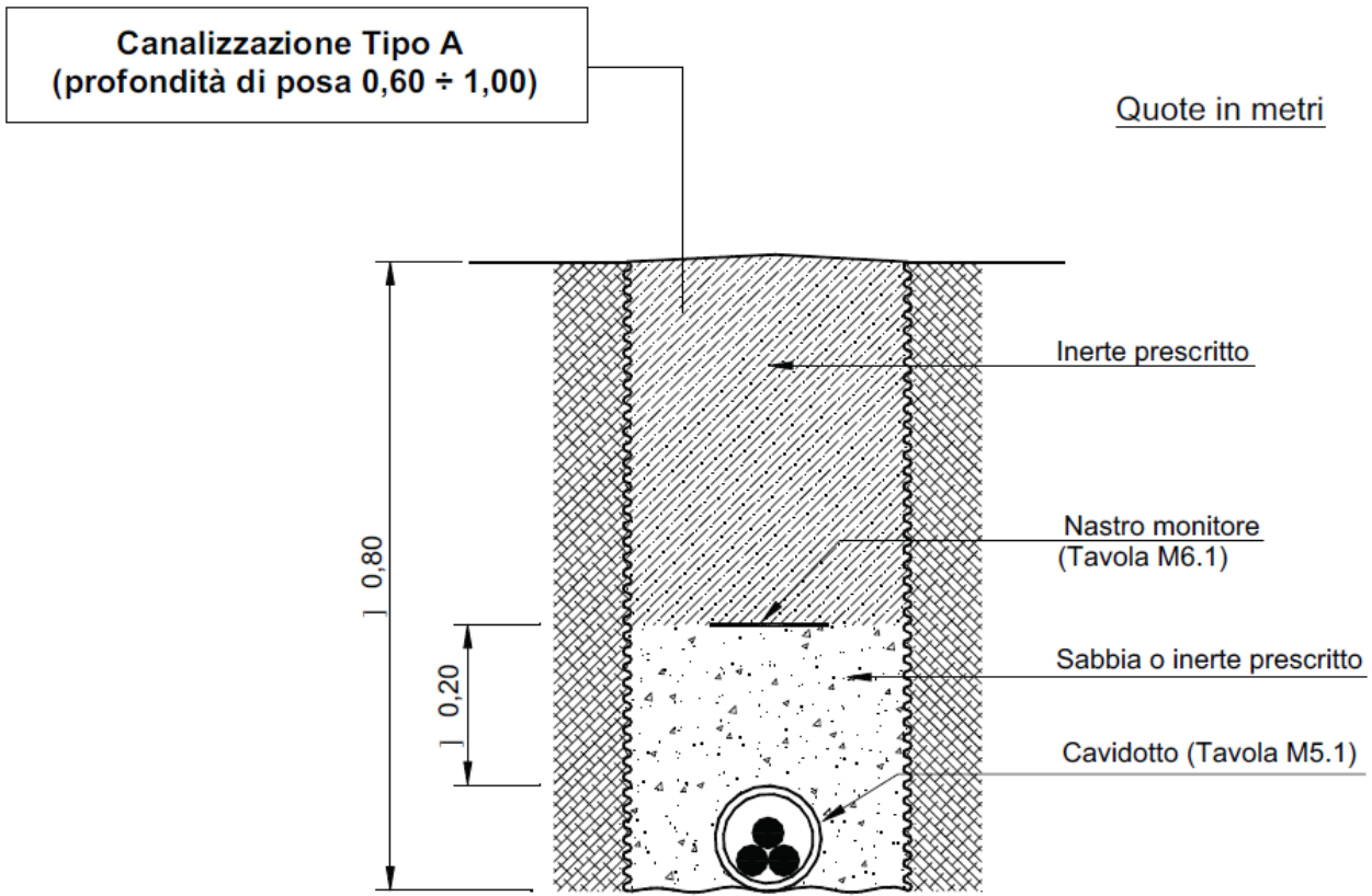
Fig. 14b: Profondità minima dei cavidotti su strada sterrata o terreno agricolo
