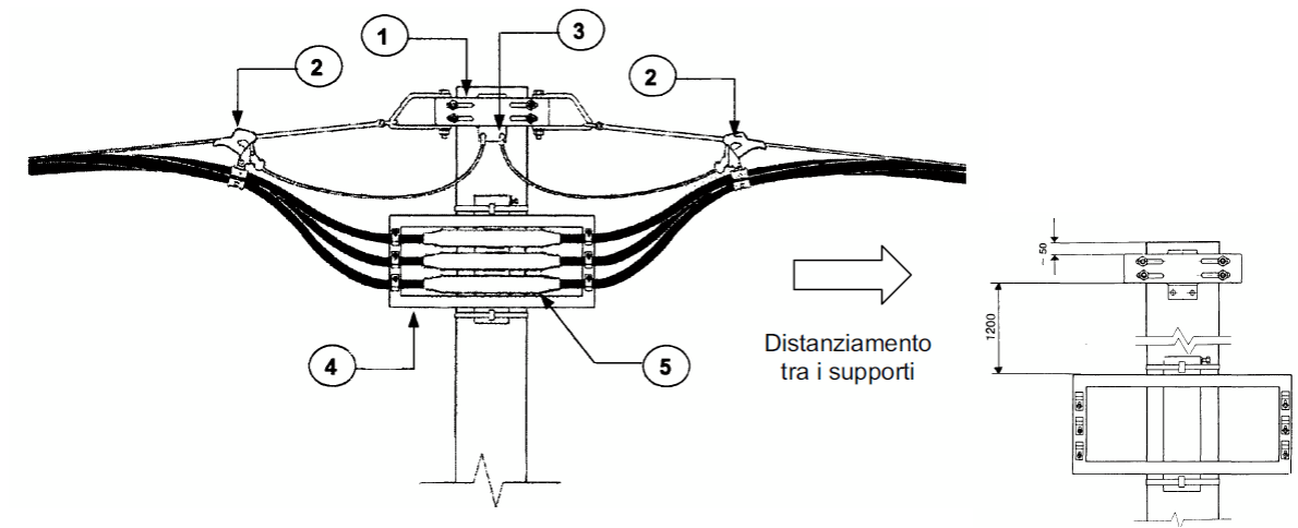
Particolare di giunzione aerea
