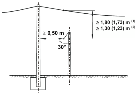
Linea di telecomunicazione, classe zero o prima in cavo aereo
