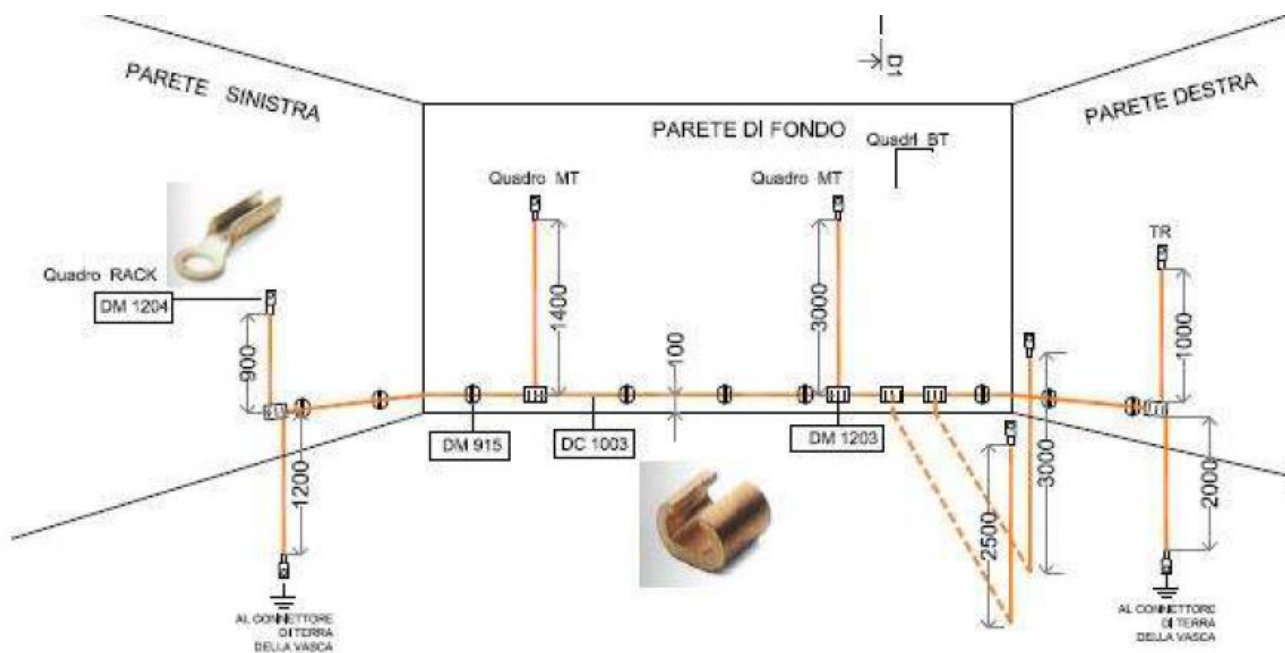
DG 2061: Pianta di terra
