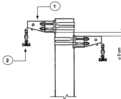
Particolare di sostegno per singola/ doppia terna
