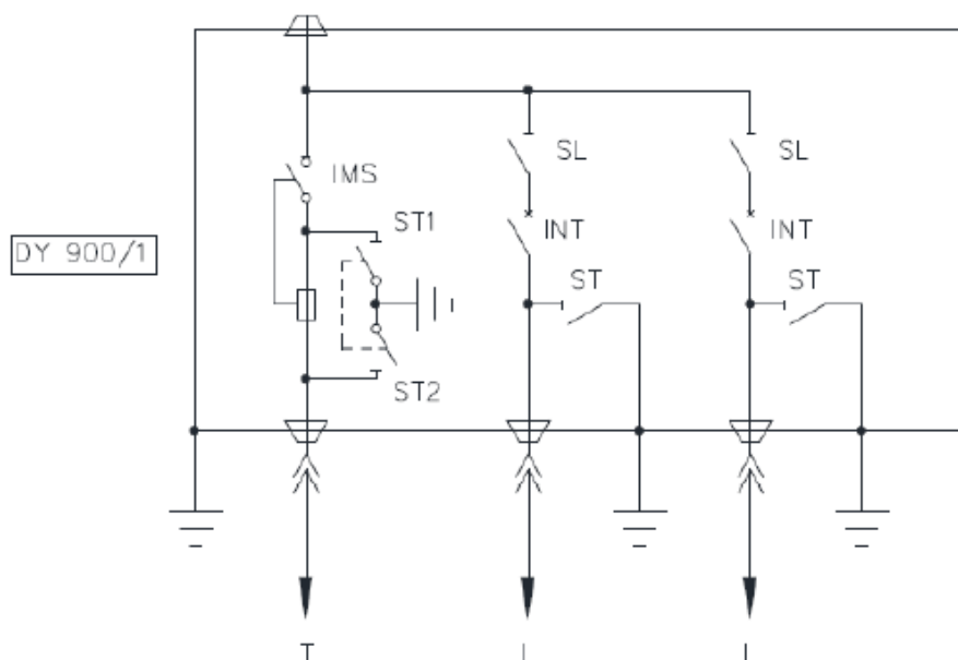
Esempio schema sinottico lato Enel nella configurazione “2LEi + 1T”
