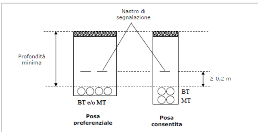
Fig. 16 Disposizione e segnalazione dei cavidotti
