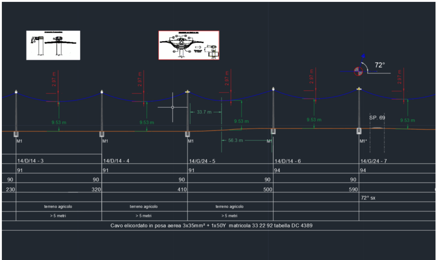
Rappresentazione della catenaria con profilo altimetrico in “dislivello” (campata l: 90 m – h: 3 m – x 1 : 33.7 m - x 2 : 56.3 m)
