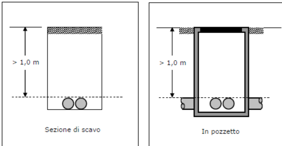
Fig. 15 Profondità minima dei cavidotti
