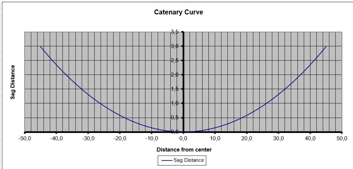
Rappresentazione della catenaria "a livello" più estesa (campata 90 m – max freccia: = 2.97 m)
