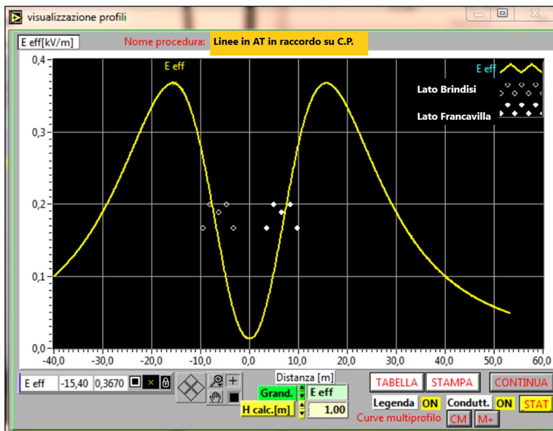
Fig. 5a – Ipotesi di valutazione del campo elettrico sui raccordi RTN di CP Mesagne
