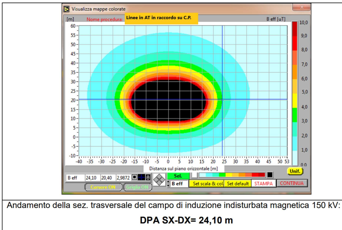
Fig. 5b – Ipotesi di valutazione del campo magnetico sui raccordi RTN di CP Mesagne
