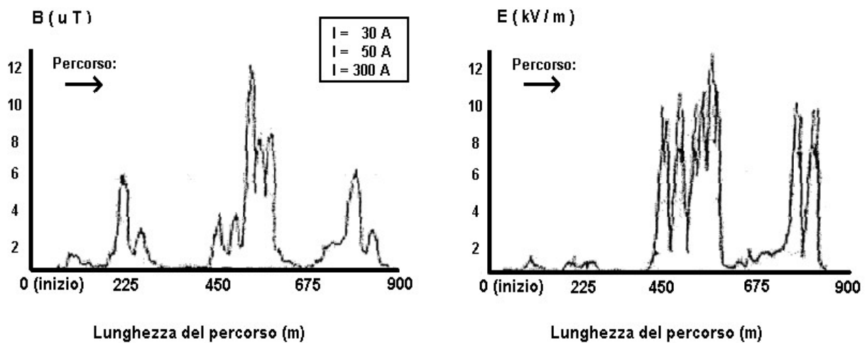
Fig. 2 - Risultati della misura dei campi elettrici e magnetici effettuate lungo le vie interne della sezione a 380 kV della stazione riportata in fig. 1a
