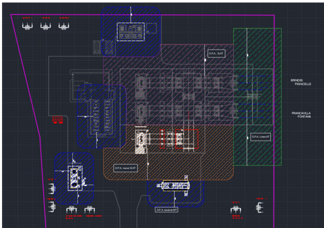
Fig. 6 – Rappresentazione, post opera, del campo magnetico sui raccordi RTN di CP Mesagne
