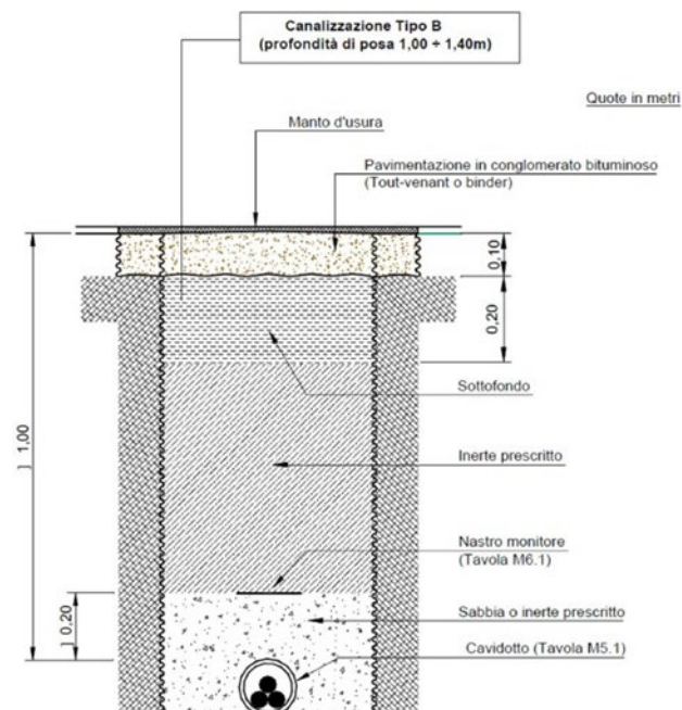
Figura 13 Particolare schema di posizionamento cavidotto
