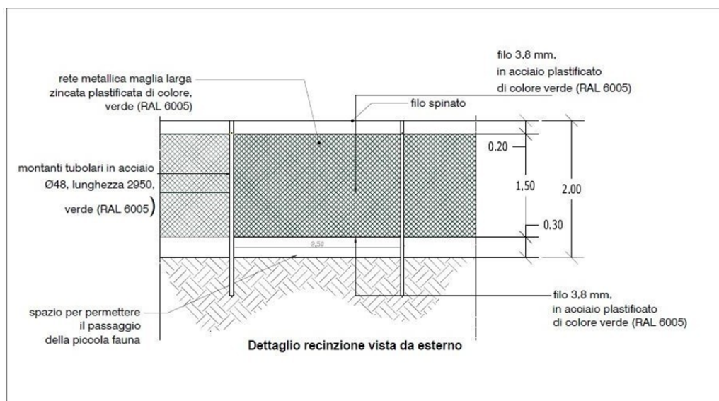
Figura 31 particolare costruttivo recinzione
