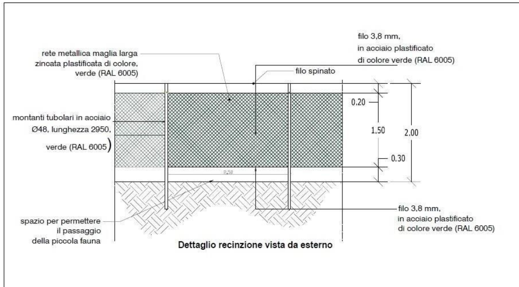
Figura 10 Figura 10 Particolare costruttivo: Recinzione
