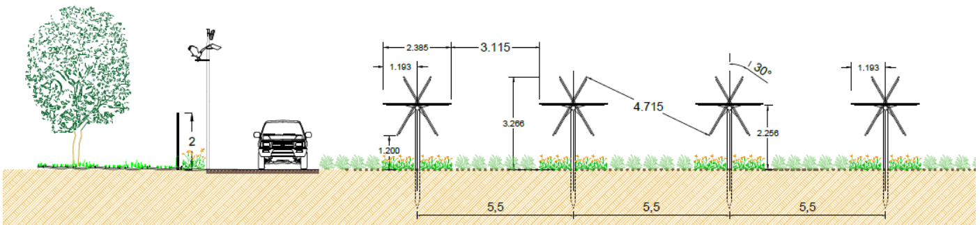
Figura 8 Particolare costruttivo: Strutture di sostegno, tracker 1V30
