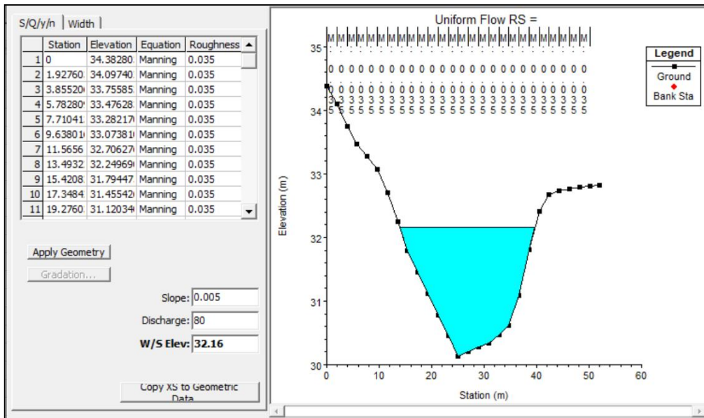
Figura 16 - Verifica idraulica recapito Sigonella 4 (massima capacità idraulica del CIR)
