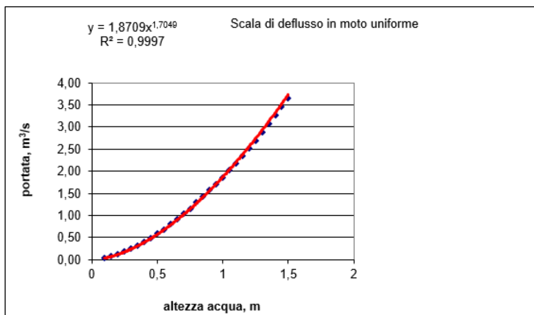
Figura 9. Canali di laminazione: scala di deflusso canale Tipo 1 (formula di Chezy, ipotesi descritte nel testo)
