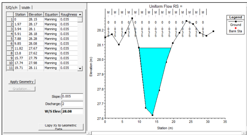
Figura 13 - Verifica idraulica recapito Sigonella 1 (massima capacità idraulica del CIR)
