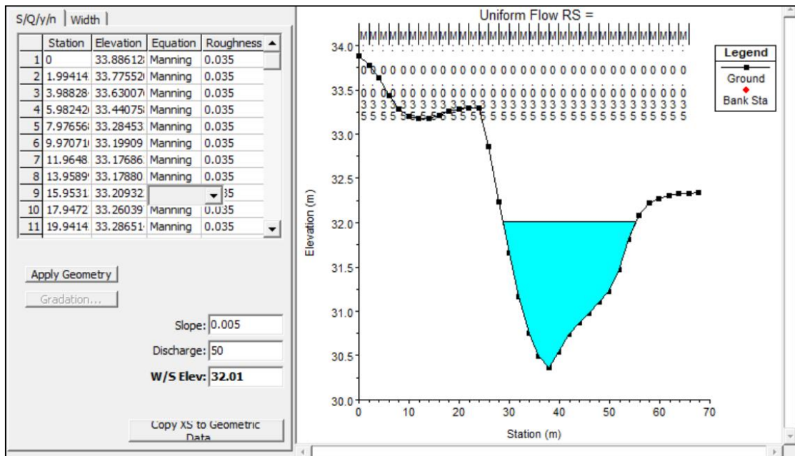
Figura 15 - Verifica idraulica recapito Sigonella 3 (massima capacità idraulica del CIR)
