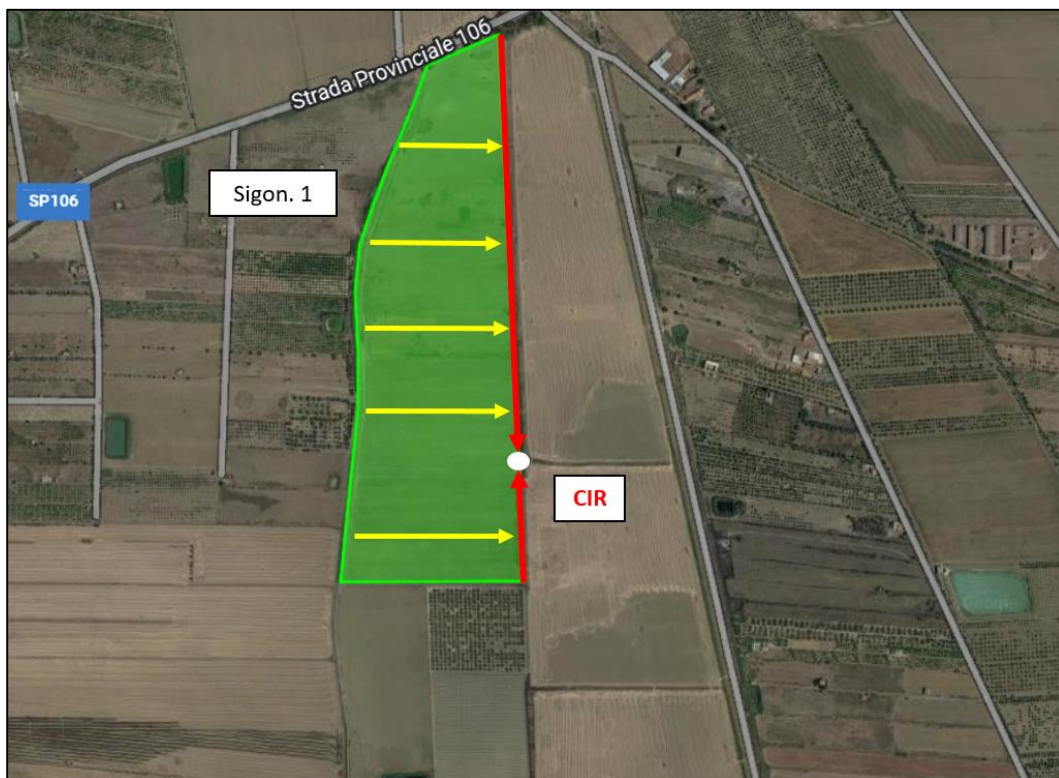
Figura 5. Campo Sigonella 1 – Individuazione sistema di laminazione (in rosso, elementi del sistema di laminazione; in giallo, direzioni di deflusso degli elementi di drenaggio non a scopo di laminazione)
