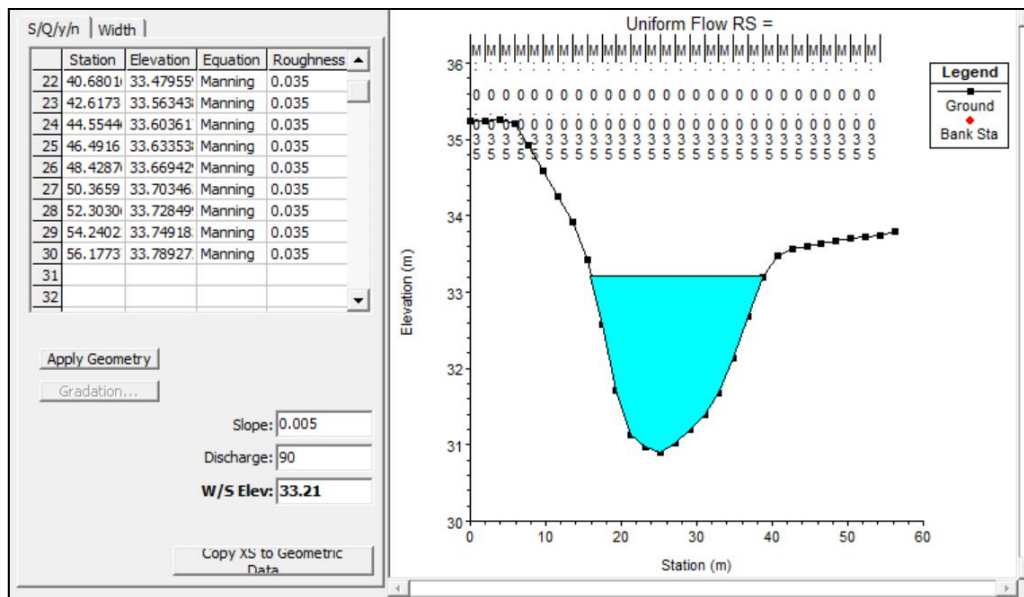
Figura 17 - Verifica idraulica recapito Sigonella 5 (massima capacità idraulica del CIR)
