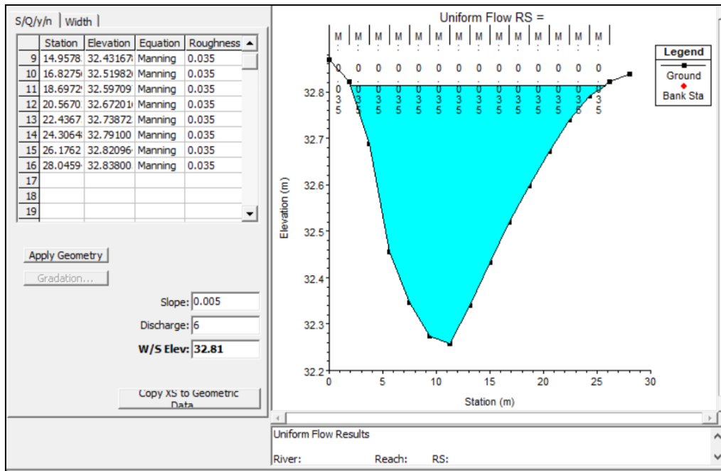
Figura 14 - Verifica idraulica recapito Sigonella 2 (massima capacità idraulica del CIR)
