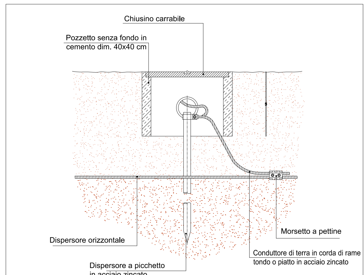
PARTICOLARE POZZETTO DI DISPERSIONE DI TERRA
