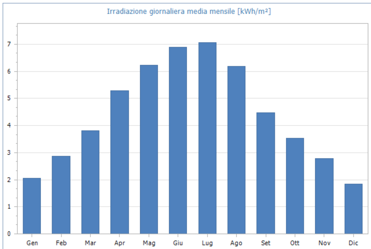
Fig. 1: Irradiazione giornaliera media mensile sul piano orizzontale [kWh/m 2 ]- Fonte dati: UNI 10349:2016 - Stazione di rilevazione: Trapani Fulgatore
