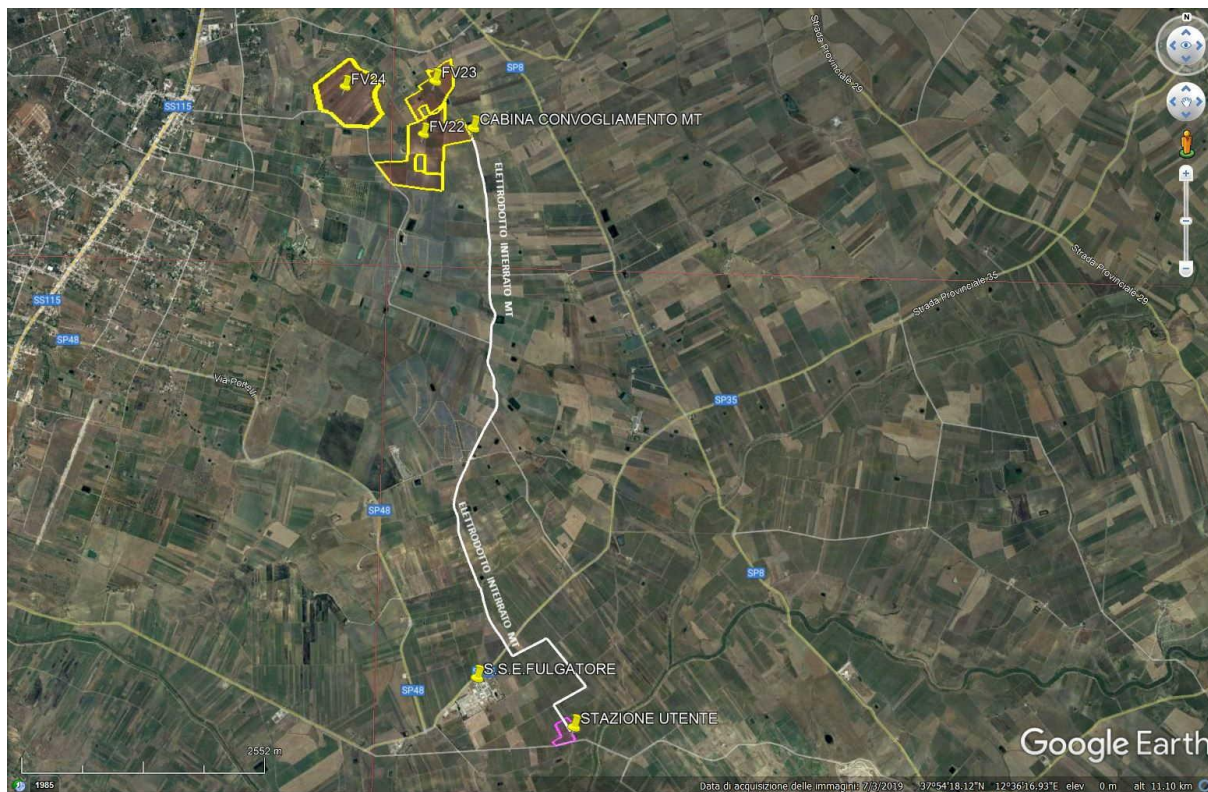
Fig. 4 ELETTRODOTTO MT CONNESSIONE IMPIANTO FV-RTN
