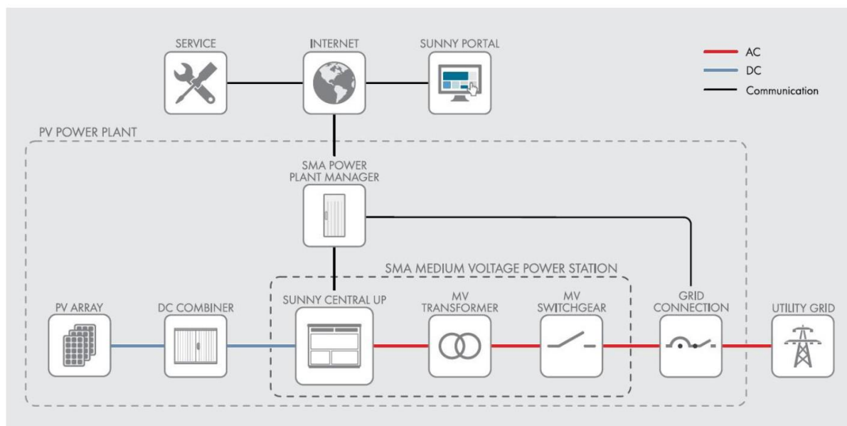
Fig. 6 SCHEMA FUNZIONAMENTO IMPIANTO
