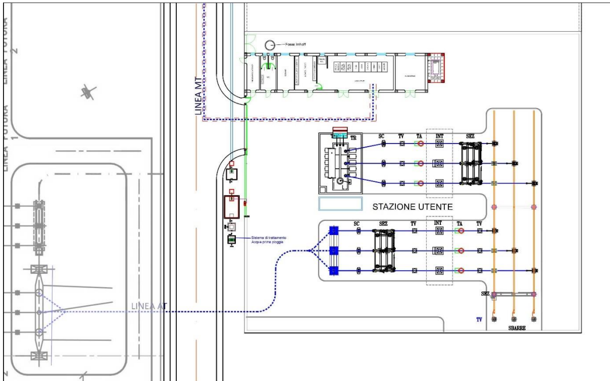
Fig. 5 LAYOUT STAZIONE UTENTE
