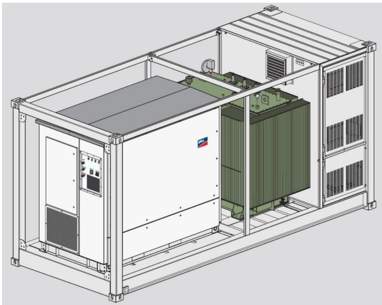
Fig. 8 - POWER STATION TIPO CON QUADRO, INVERTER E TRASFORMATORE ELEVATORE
