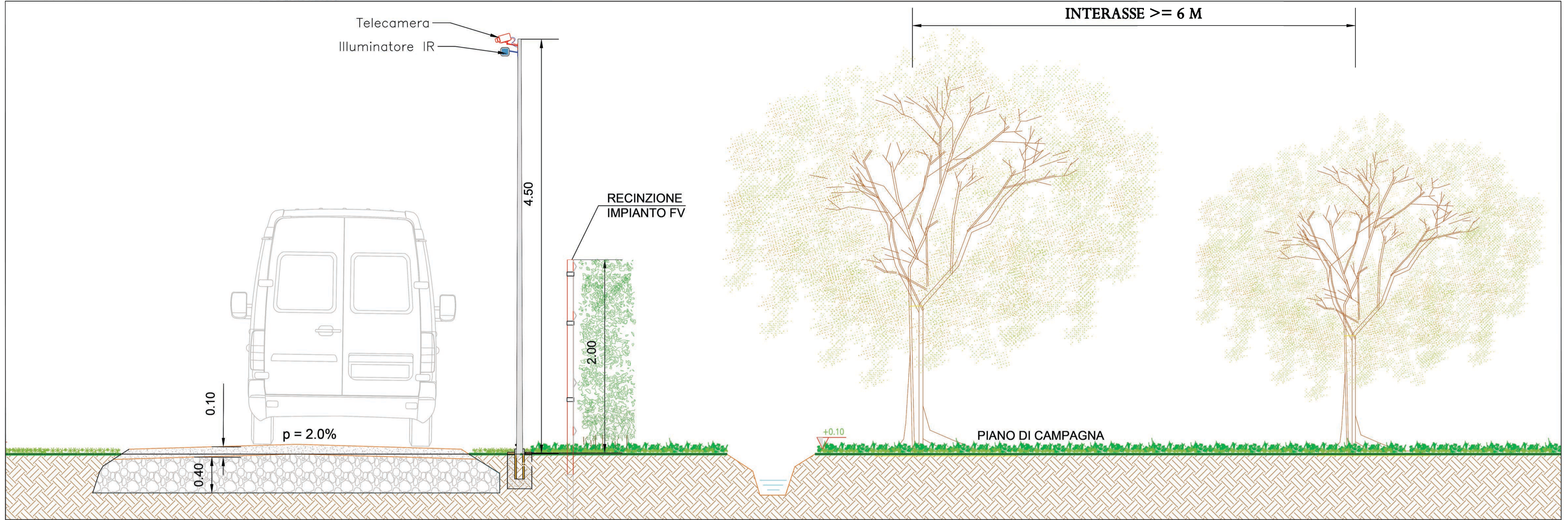
TIPICO FASCIA ARBOREA - VISTA IN PROSPETTO SCALA 1:20
