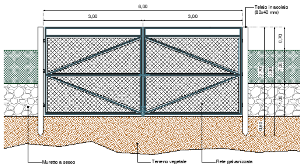
Figura 4 - Cancello
