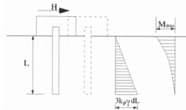
Figura 18 - Resistenza limite del terreno di un palo impedito di ruotare a testa
