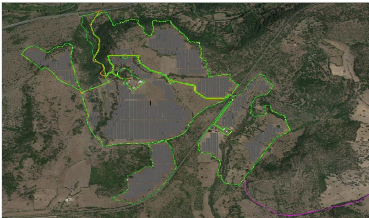
Figura 2 - Area di impianto agrivoltaico
