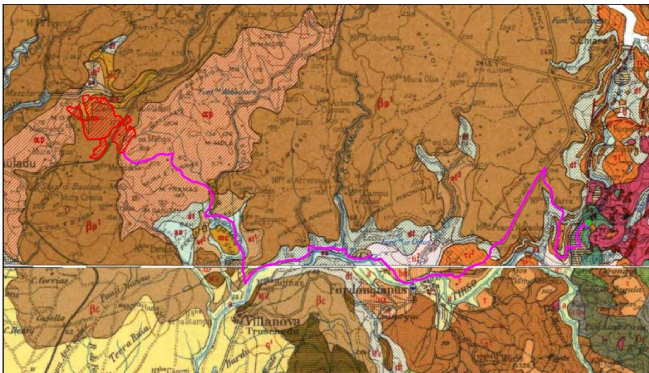
Figura 1 - Stralcio dei Fogli 205-206 "Capo Mannu-Macomer" e 216-217 "Capo S.Marco-Oristano" della Carta Geologica d'Italia, scala 1:100000 relativo al sito di progetto
