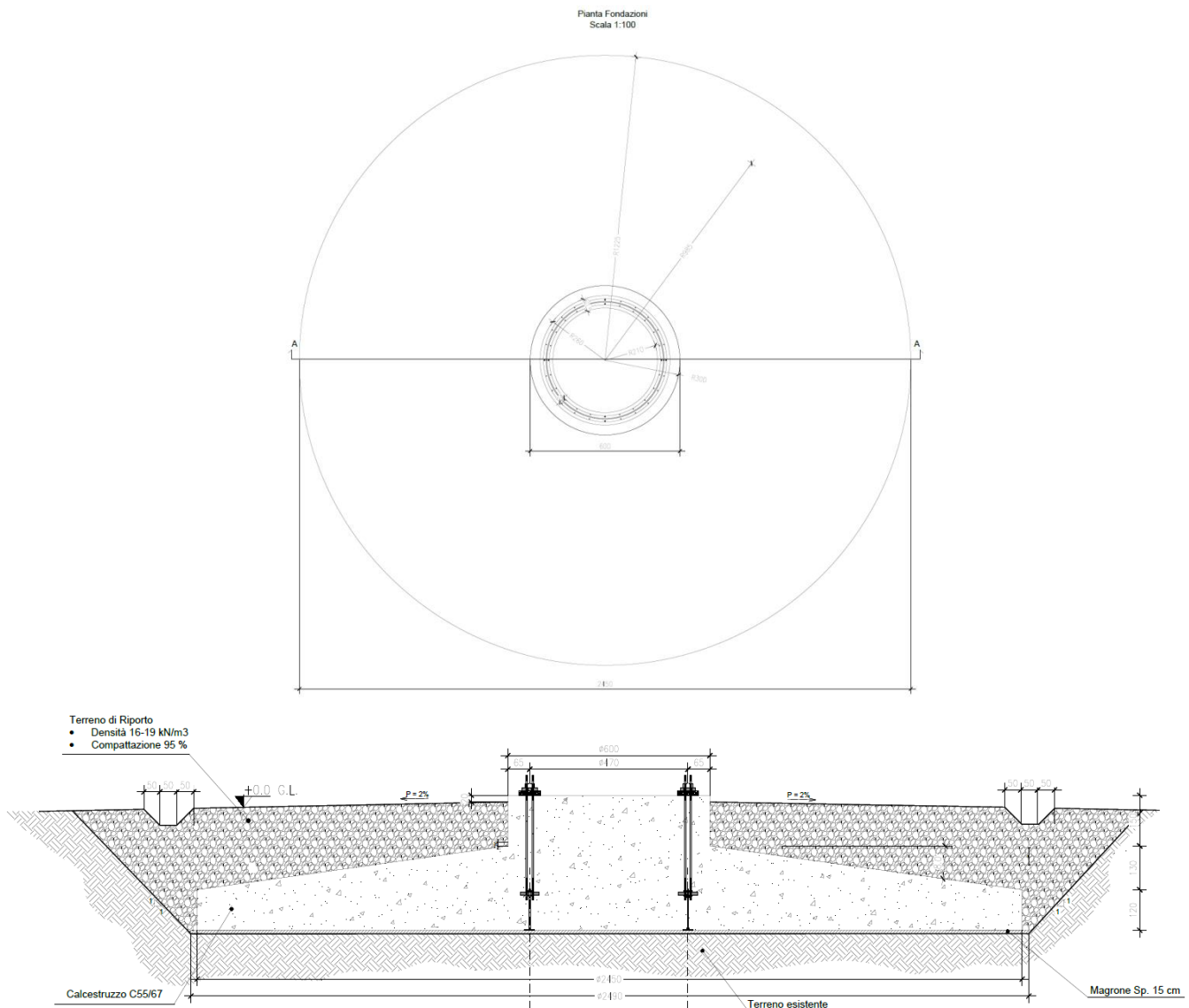
Figura 1: Tipologico fondazione aerogeneratore. Estratto elaborato
