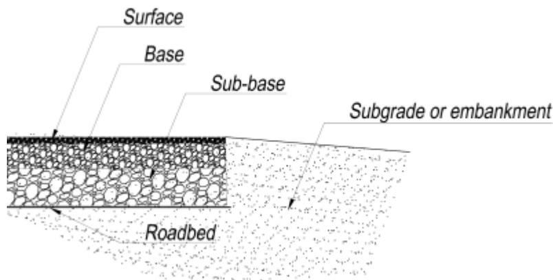
Figura 3: Sezione-tipo stradale con sottofondo
