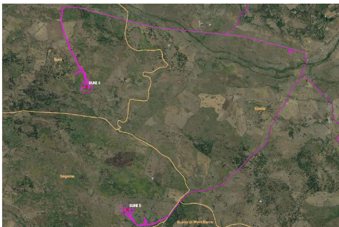
Figura 3: Sovrapposizione del layout di impianto su base satellitare: in magenta la viabilità di impianto ed i tracciati dei cavidotti, in rosso gli aerogeneratori SUNI 4, ricadente nel comune di Suni e SUNI 5 nel comune di Sagama.
