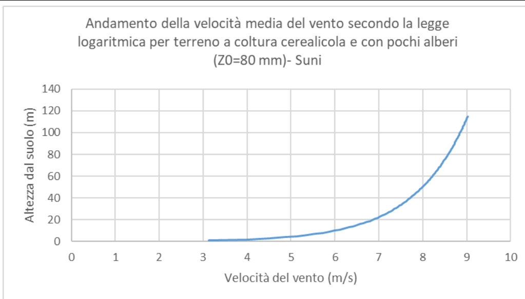
Figura 7: Andamento della velocità media del vento secondo la legge di propagazione logaritmica per terreni a coltura cerealicola ( Z_0=80 mm)
