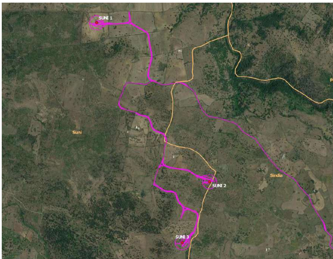
Figura 2: Sovrapposizione del layout di impianto su base satellitare: in magenta la viabilità di impianto ed i tracciati dei cavidotti, in rosso gli aerogeneratori SUNI 1, SUNI 2 e SUNI 3 ricadenti nel comune di Suni.
