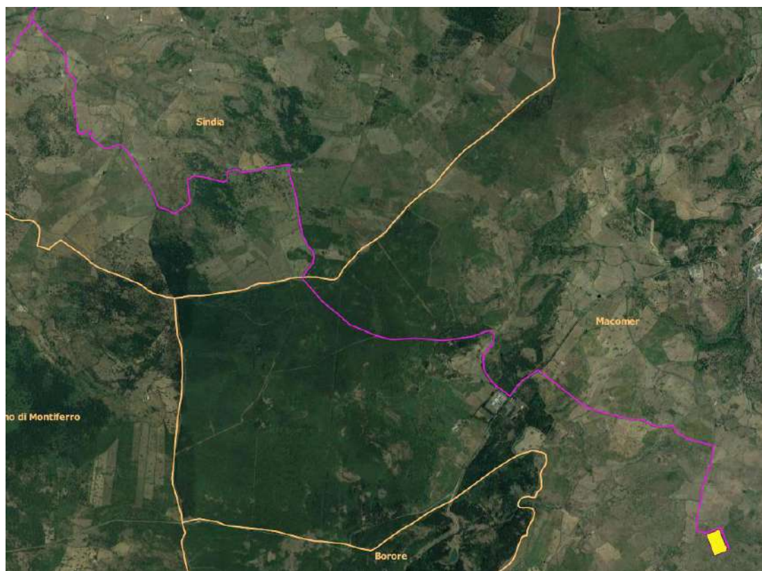
Figura 4: Sovrapposizione del layout di impianto su base satellitare: in magenta il cavidotto di connessione, in giallo la Futura SE di Terna 380/150/36 kV “Macomer 380”
