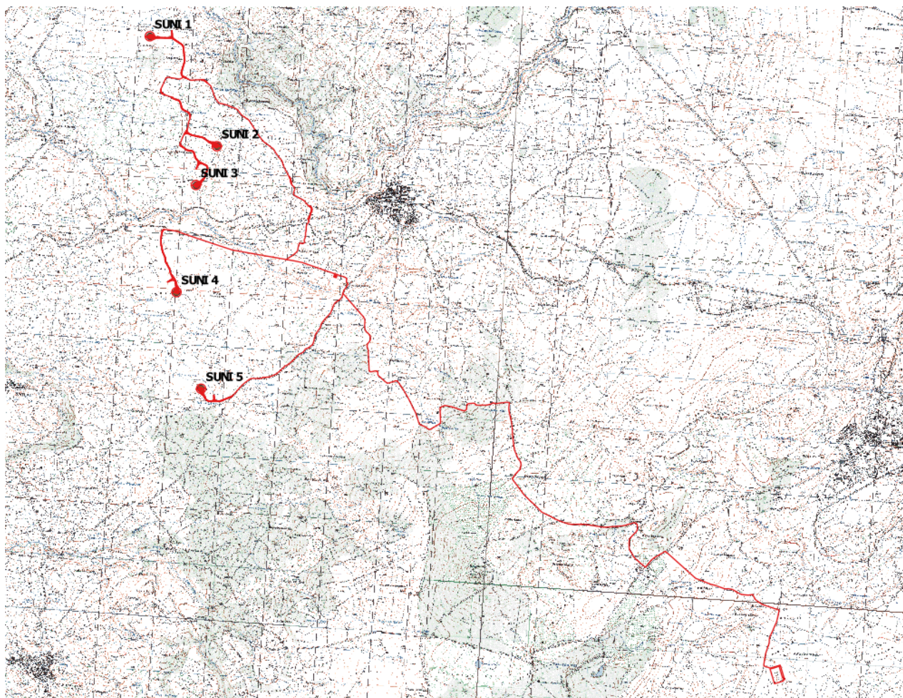
Figura 1: Inquadramento su base IGM 1:25000 del layout di impianto (in rosso)
