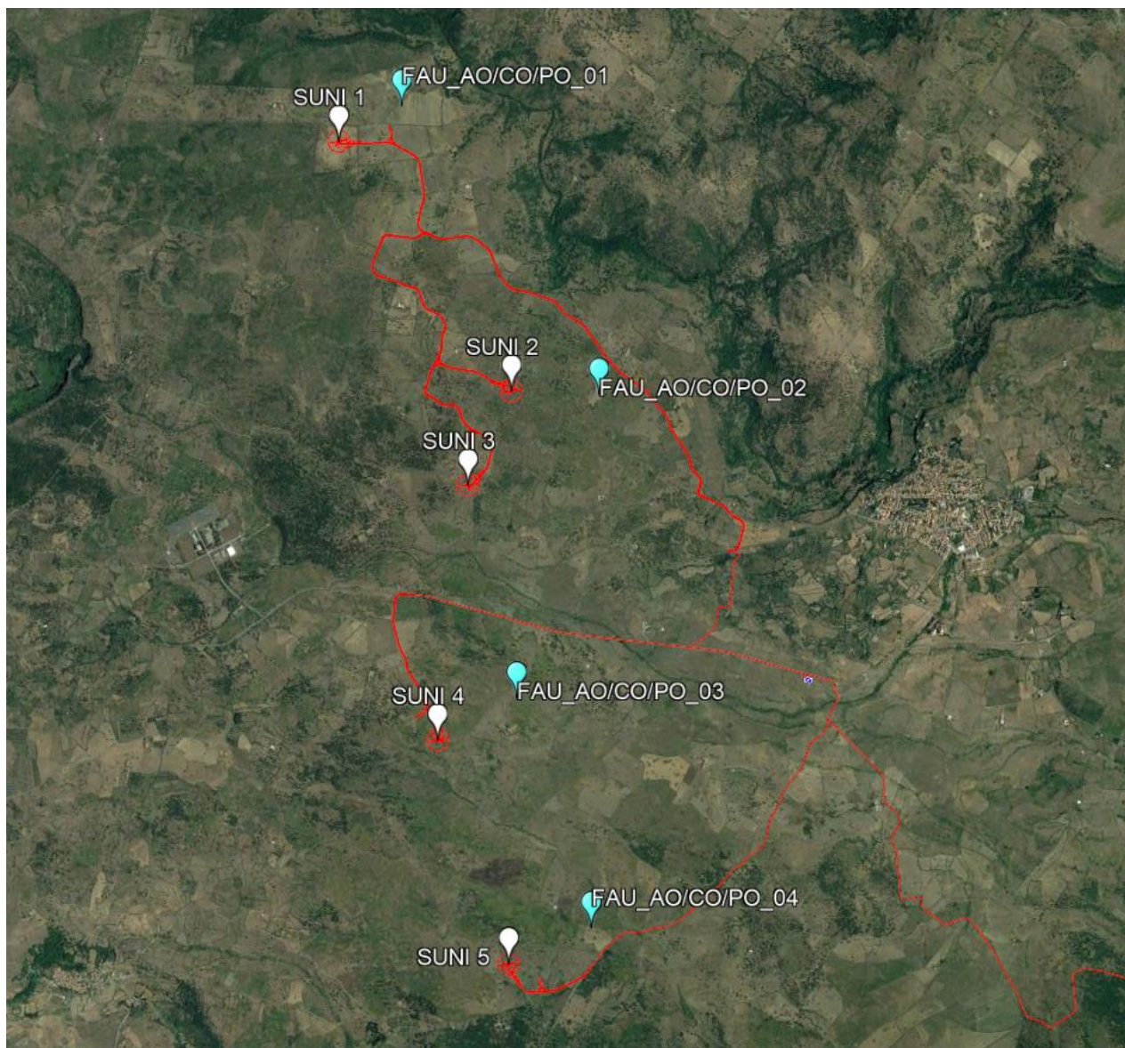
Figura 8: Inquadramento punti di monitoraggio della fauna (puntatori in azzurro) in prossimità degli aerogeneratori (puntatori in bianco)
