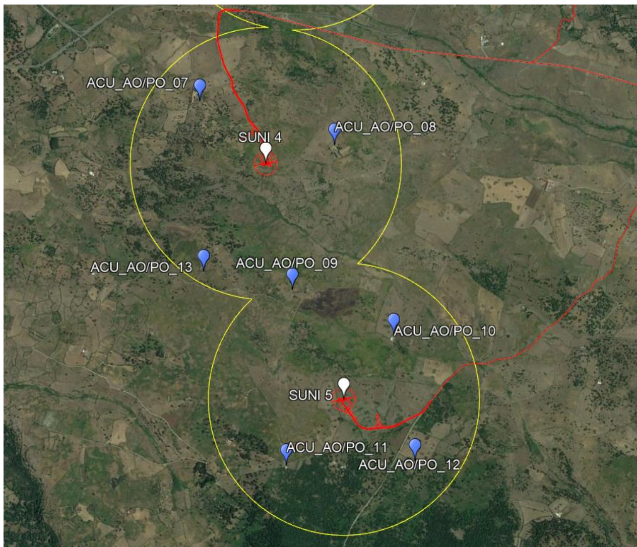
Figura 12: Ubicazione dei punti di monitoraggio per la componente rumore (puntatori blu), su base satellitare
