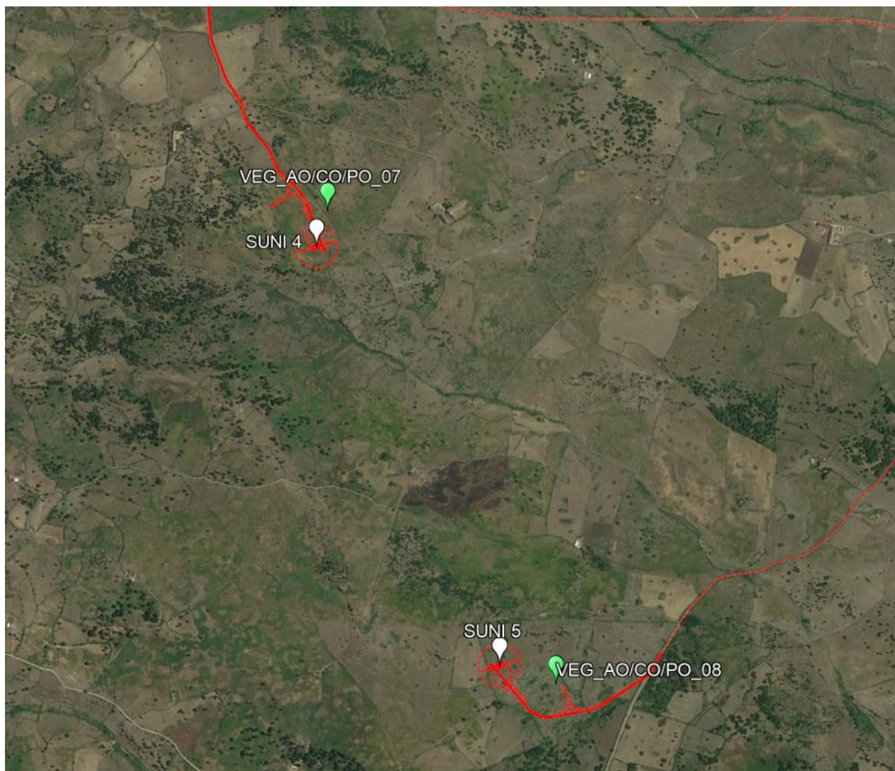
Figura 6: Inquadramento dei punti di monitoraggio per flora e vegetazione (in verde) rispetto al layout di progetto (in rosso) su immagini satellitari (Fonte: Google satellite)
