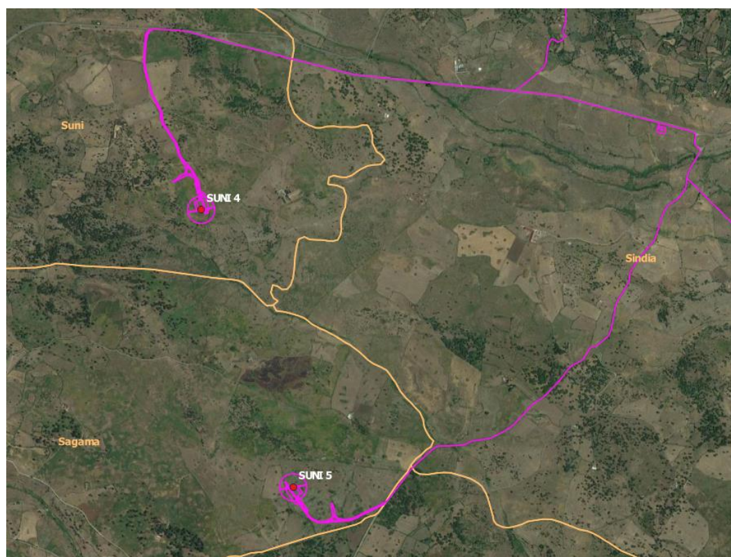
Figura 3: Inquadramento territoriale su base satellitare del layout di impianto (in magenta) – in figura sono illustrate gli aerogeneratori (pallini rossi) SUNI 4, SUNI 5 e i relativi cavidotti di connessione
