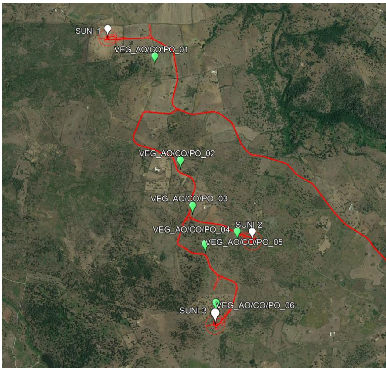
Figura 5: Inquadramento dei punti di monitoraggio per la componente vegetazione (puntatori verdi) rispetto al layout di impianto su immagine satellitare _ Fonte: Google Earth
