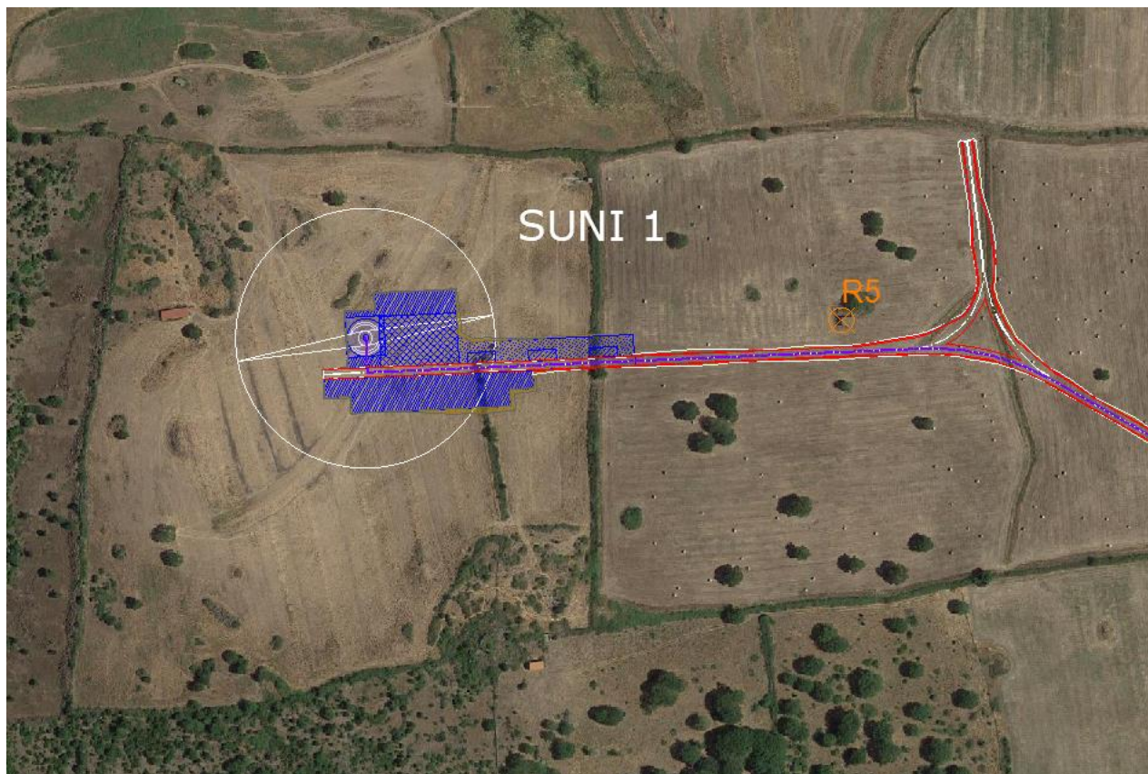
Figura 10: Inquadramento su base satellitare del recettore R5 rispetto all'aerogeneratore SUNI 1
