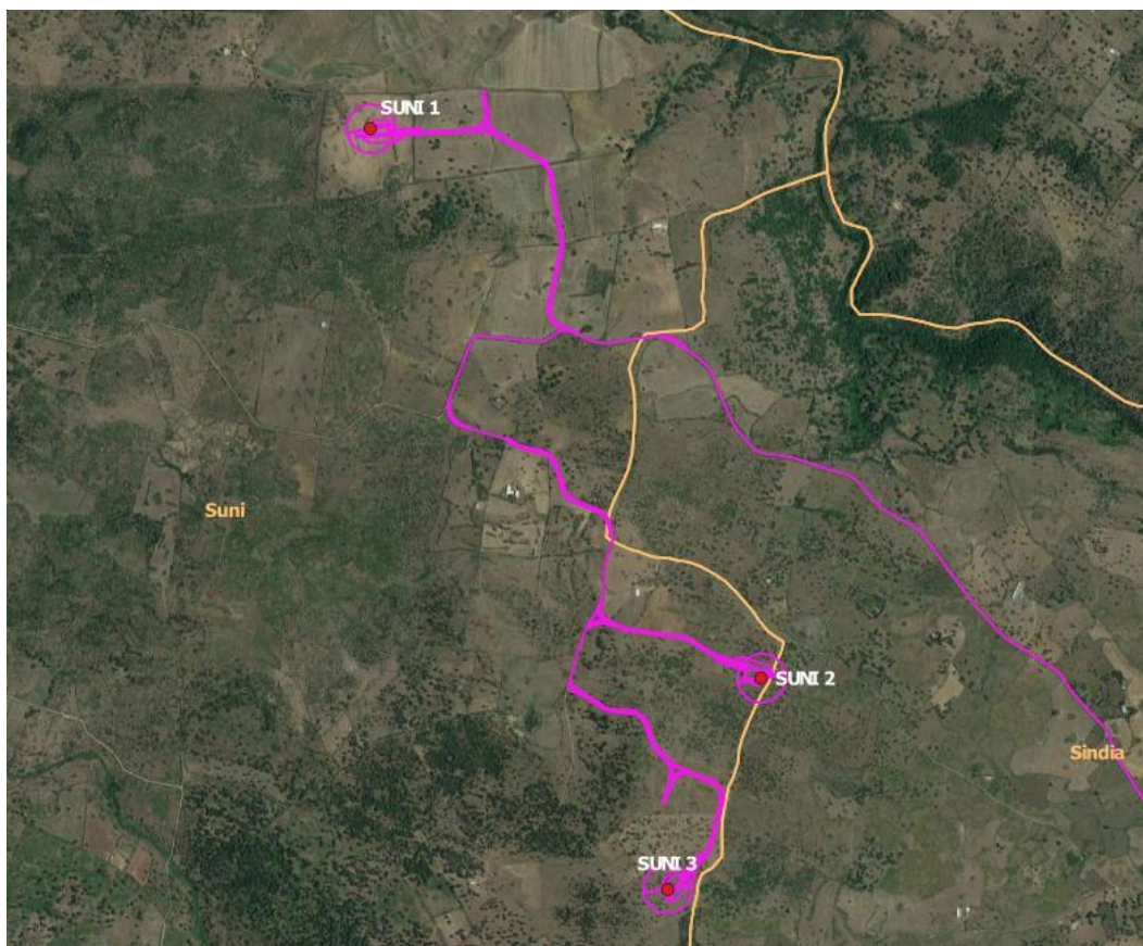
Figura 2: Inquadramento territoriale su base satellitare del layout di impianto (in magenta) – in figura sono illustrate gli aerogeneratori (pallini rossi) SUNI 1, SUNI 2, SUNI 3, e i relativi cavidotti di connessione
