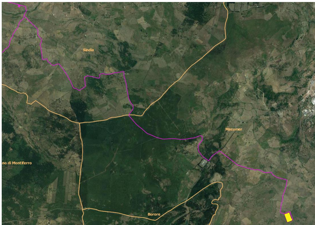
Figura 4: Inquadramento territoriale su base satellitare del layout di impianto – in figura il cavidotto di connessione AT (in magenta) e la Futura SE Terna 380/150/36 kV “Macomer 380”
