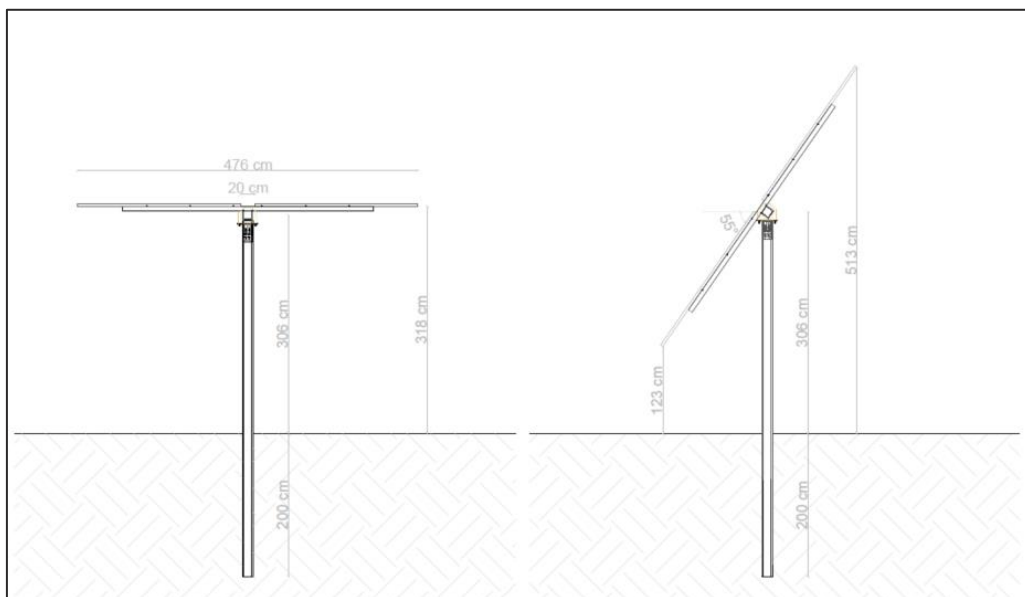
FIGURA 2: TRACKER TIPO AD ASSE VARIABILE
