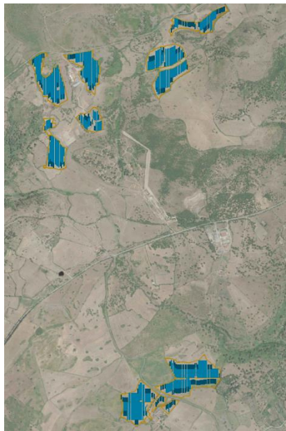
FIGURA 4: LAYOUT DI PROGETTO
