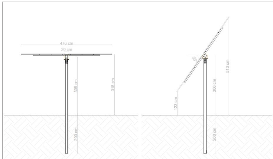
FIGURA 1: TRACKER SOLARE TIPO
